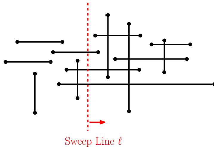
図 3.4: 水平・垂直線分の平面走査法
