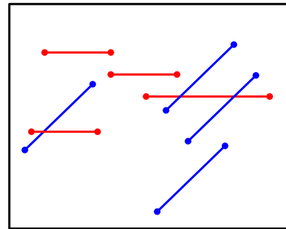
(b) 各2種類の異なる傾きの線分集合に対して交差を計算
