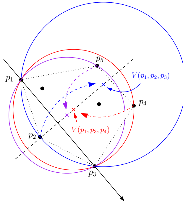
図 2.4: E(p_1, p_3) の終点を計算する . 有向直線 \overrightarrow{p_1 p_3} の左側にある S の凸包上の点は p_4 と p_5 がある . (p_1, p_3, p_4) で定義される円の方が大きいので , E(p_1, p_3) の終点は V(p_1, p_3, p_4) である . 逆に , 有向直線 \overrightarrow{p_3 p_1} の左側には p_2 だけがある . よって , E(p_3, p_1) の終点は , V(p_3, p_1, p_2) = V(p_1, p_3, p_2) である .
