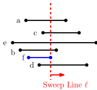
(a) 走査線状態から線分 f を削除
