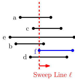
(a) 走査線状態に線分 f を追加
