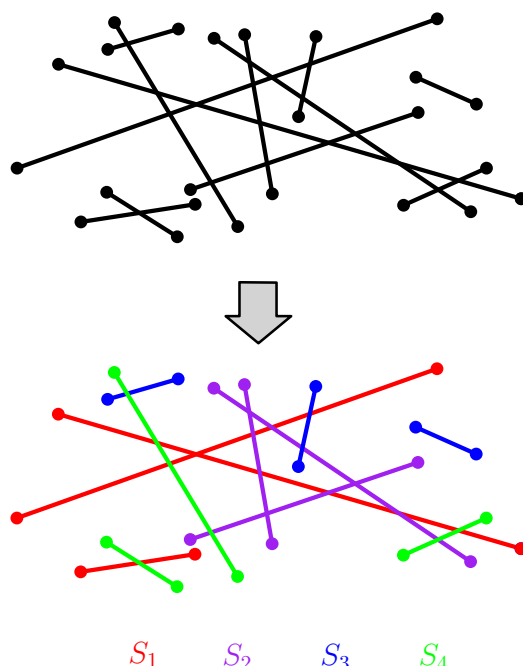
図 3.2: S をそれぞれちょうど 3 本の線分を含む部分集合 S_1, S_2, S_3, S_4 に分割． |S_i| = 3, i = 1, 2, 3, 4 ．
