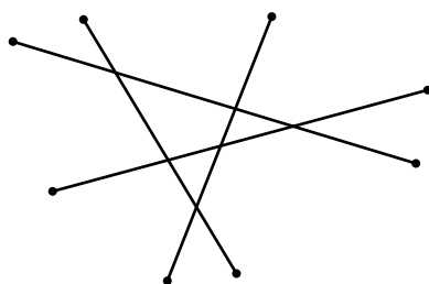
図 3.8: 分割数が最悪となる場合
