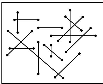
(a) 4種類の傾きをもつ線分集合
