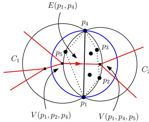
図 2.5: 青い円は線分 \overline{p_1 p_4} を直径とする円である． E(p_1, p_4) の始点と終点は, それぞれ V(p_1, p_2, p_4), V(p_1, p_4, p_5) である．よって, (p_1, p_2, p_4), (p_1, p_4, p_5) で定義される円をそれぞれ C_1, C_2 とすると, どちらの円も与えられた点を包含する円である．しかし, C_1, C_2 よりも線分 \overline{p_1 p_4} を直径とする円の方が小さい．
