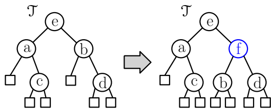
(b) \mathcal{T} の変化
