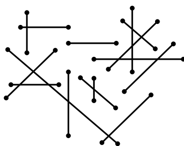
図 3.9: 4 種類の傾きをもつ線分集合の例
