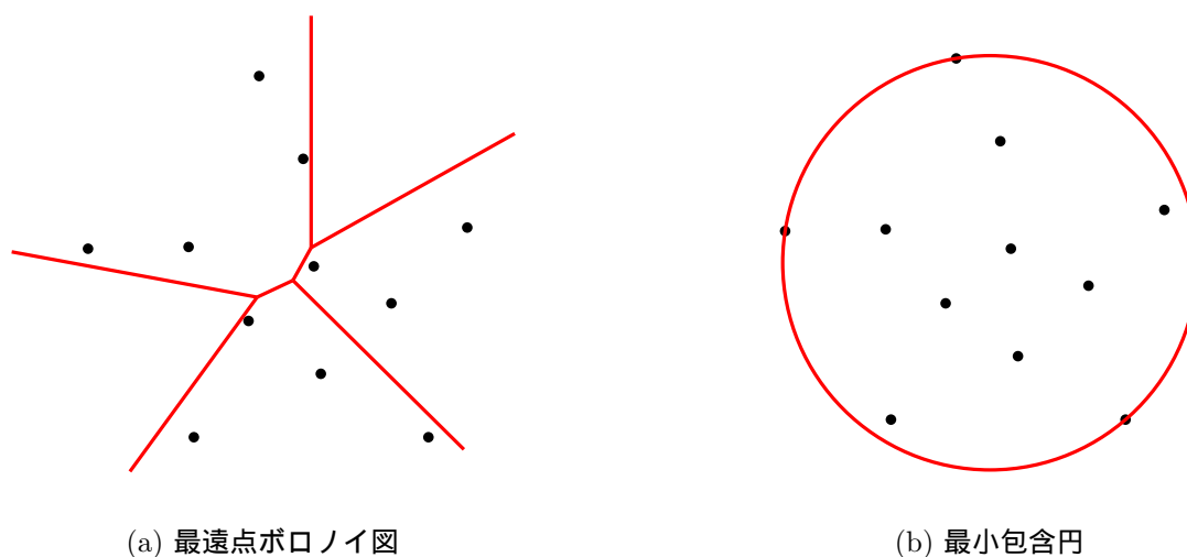
図 2.1: 点集合 S に対する最遠点ボロノイ図と最小包含円
