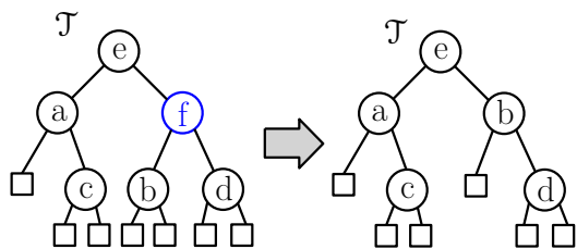
(b) \mathcal{T} の変化
