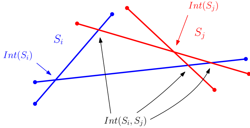
図 3.3: 第二段階で検出される交差
