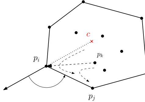
図 2.3: 重心 c と p_i を始点とする半直線を利用し, p_i の反時計回りに次の凸包上の頂点を見つける.
