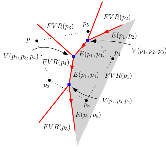
図 2.2: 最遠点ボロノイ図． \{p_1, \dots, p_5\} は凸包上の点， FVR(p_i) は点 p_i に対するボロノイ領域， E(p_i, p_j) は 2 点 p_i, p_j に対するボロノイ辺を表す．
