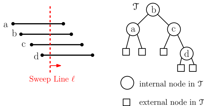
図 3.5: 平面の走査線状態と探索木 \mathcal{T}
