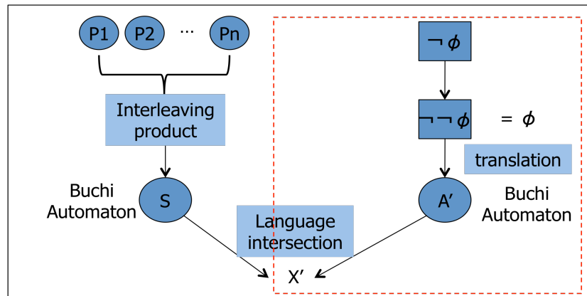
図 6 正例出力の考え方
