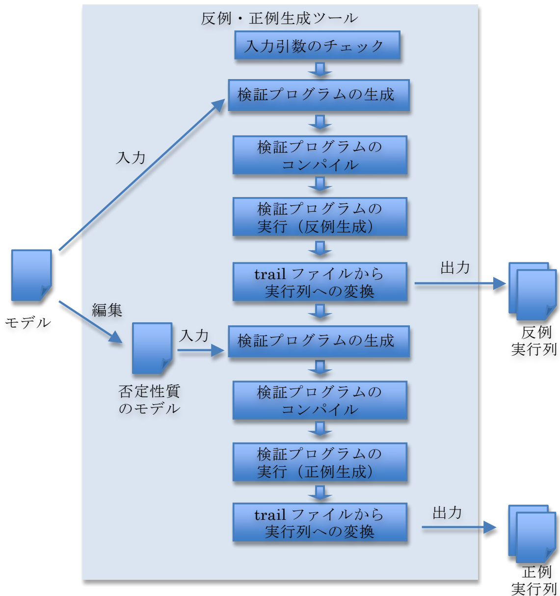
図 8 反例・正例生成ツールの処理フロー
