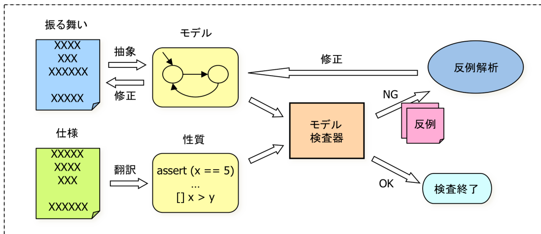
図 1 モデル検査の流れ
