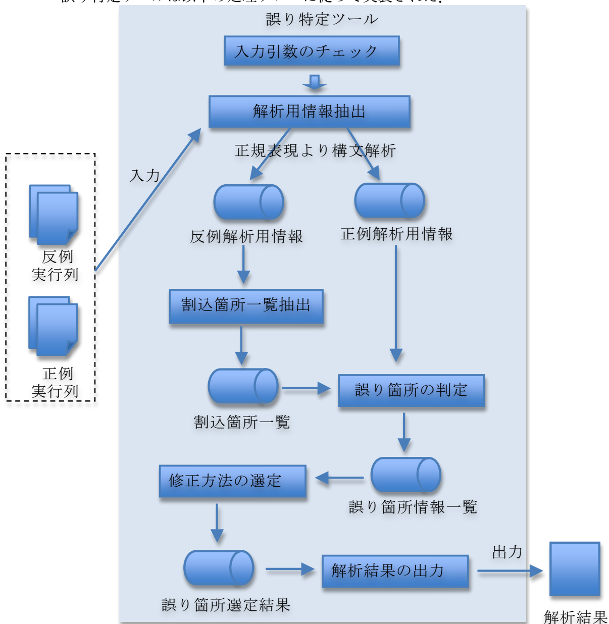
図 9 誤り特定ツールの処理フロー
