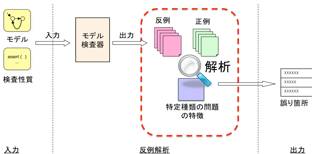
図 2 提案手法の概念図
