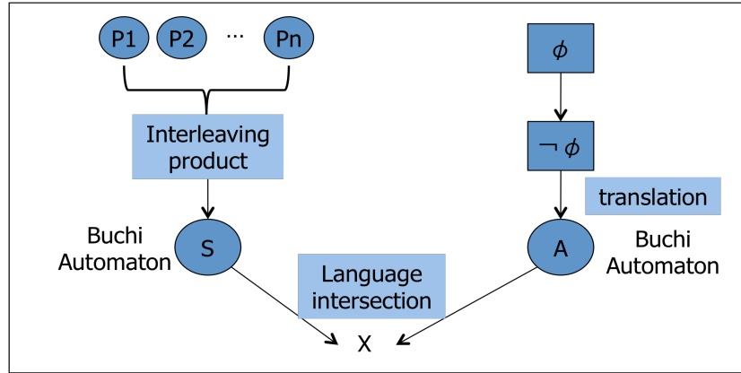
図 5 SPIN の検証アルゴリズム
