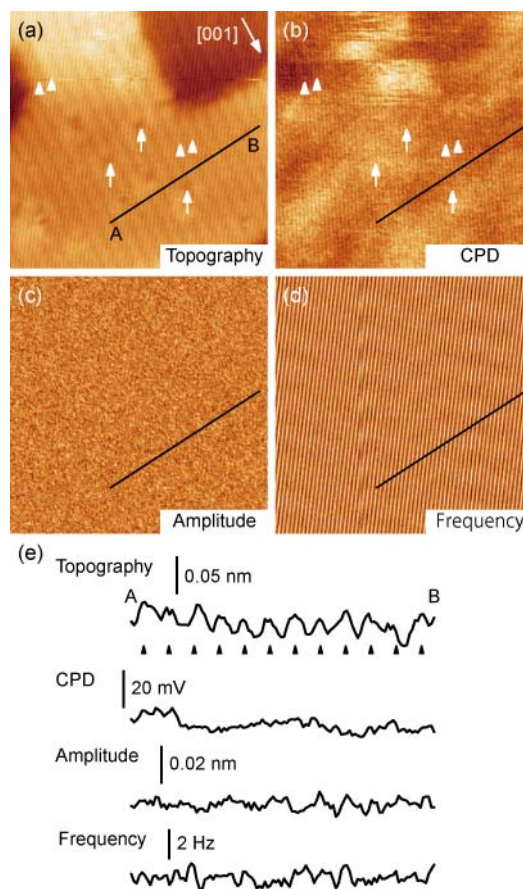
図2. \text{TiO}_2(110)-(1 \times 1) 表面の KPFM 測定結果。(a)凹凸像、(b)CPD 像、(c)探針の振動振幅像、(d)探針の振動周波数像。凹凸像では物理的に高い部分、CPD 像では CPD がより小さい部分、振幅像では振幅がより小さい部分、周波数像では周波数がより低い部分が明るく表されている。(e)画像中の直線に沿った断面図。矢頭は O 原子列の位置を表す。画像サイズ: 15 nm × 15 nm、周波数シフト ( \Delta f ): -88 Hz、カンチレバーの振動の全振幅 ( A_{pp} ): 3.3 nm。
