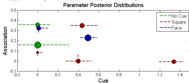
図 6: Wu & Kirkham (2010)の実験データに対し、推定された、手がかり、連想関係パラメータの事後分布。
