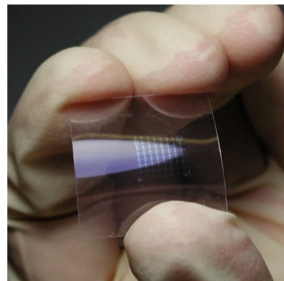
図2 細野教授が発明した IGZO TFT
