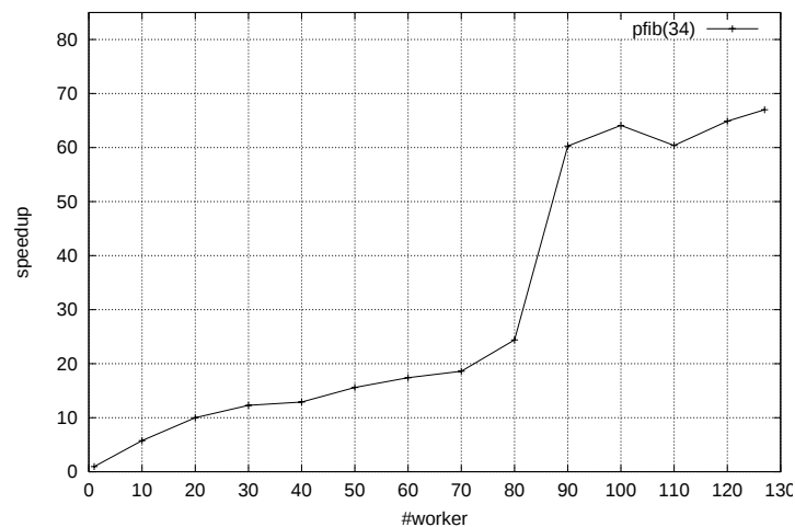
図 6.1: pfib(34) の速度向上比
