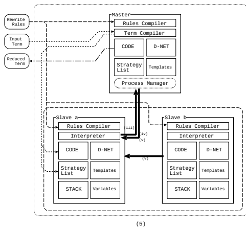
図 5.21: 超並列 TRAM の処理の詳細な流れ
