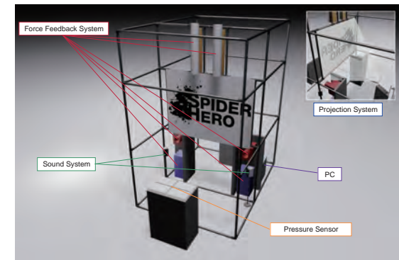
図2 (上図) システムの全体構成 (下図) システムレイアウト Fig. 2 (Upper) System overview (Lower) System layout
