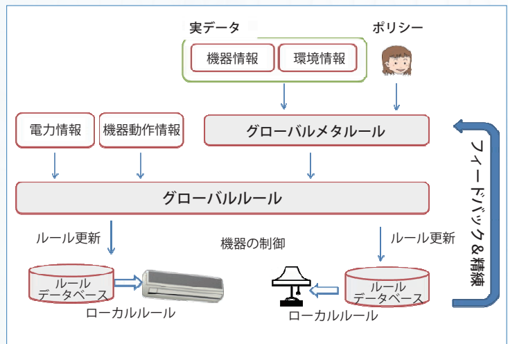
図-4 ルール変換のアーキテクチャ
