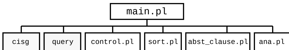
図 C.1 本システムのモジュール構成
