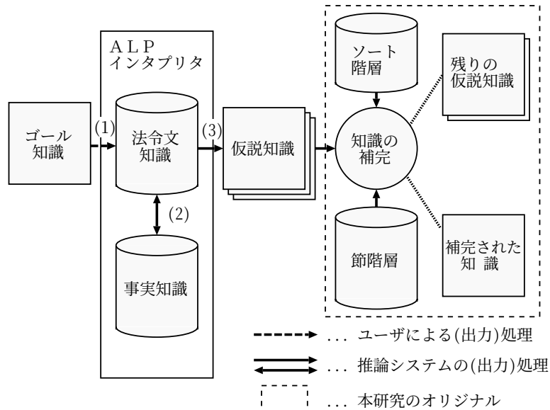
図 4.6: 類推解釈機構
