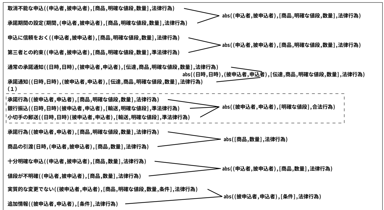
図 5.2: 知識階層生成実験により生成された節階層
