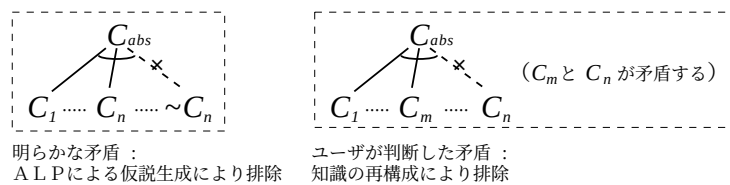
図 4.9: 不正な更新の回避
