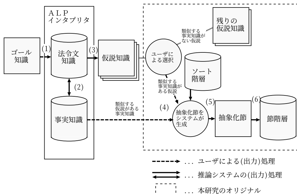
図 4.2: 知識階層生成機構
