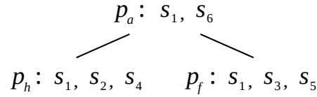
図 4.4: 生成される節階層
