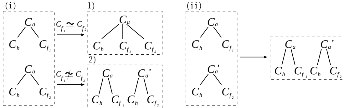
図 4.5: 生成される節階層の相互作用
