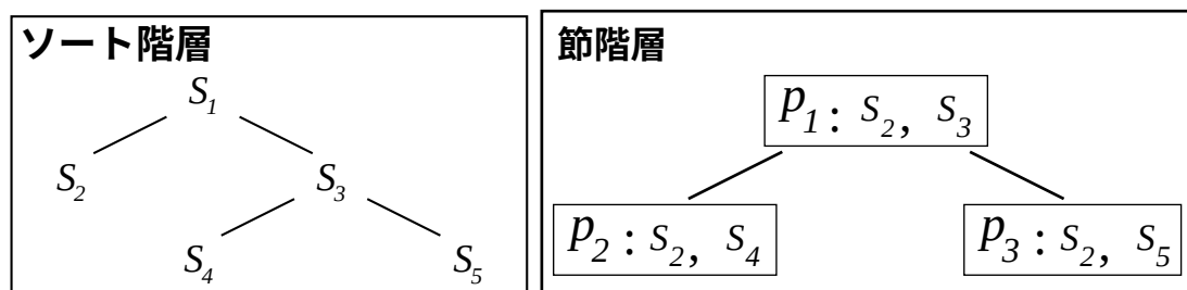
図 4.3: ソート階層と節階層
