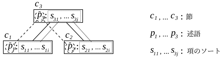
図 4.8: 抽象化節の生成
