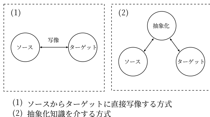
図 3.1: 類推モデル
