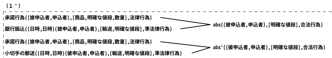
図 5.3: ユーザが解釈を替えた場合の節階層
