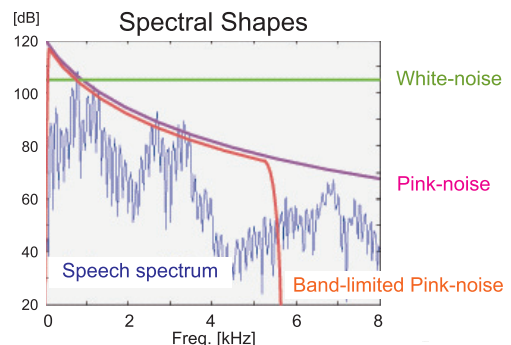
図2 ホワイトノイズ、ピンクノイズ、帯域制限されたピンクノイズによるマスキングの概念図
