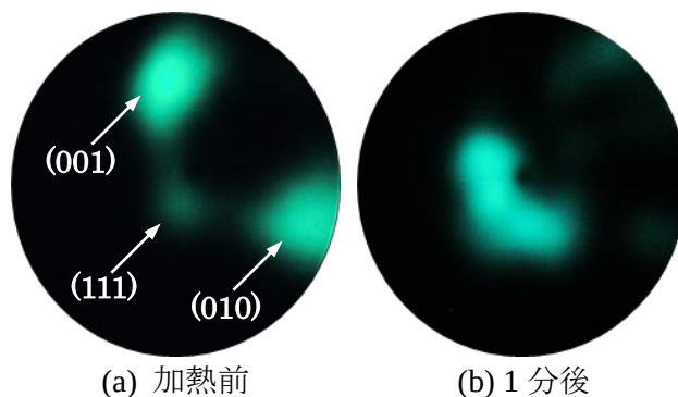
図1 Ptをスパッタ堆積させた多結晶Wを加熱してbuild upしたときのFEM像 (-0.25kV)
