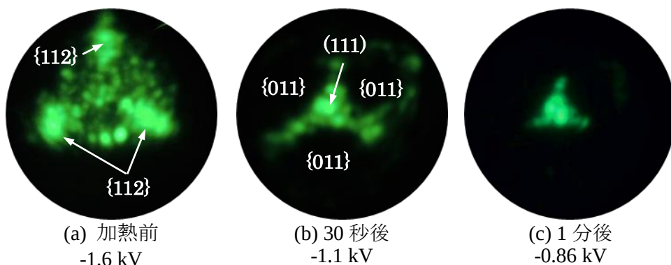
図2 [111]方位の単結晶Wを高電界下で加熱してbuild upしたときのFEM像
