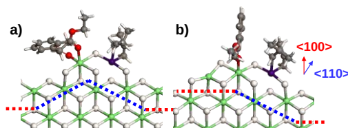
図2 最も確からしい活性点：a) {110} エッジ (例：フタル酸ジエチル)、b) {110} ステップ (例：安息香酸エチル)
