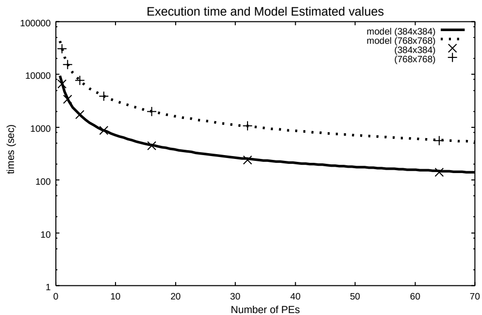
図 6.7: 実行時間とモデルによる見積もり（1次元領域分割）
