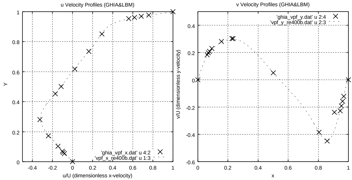
図 6.3: Re = 400 のキャビティ流れの速度プロファイル
