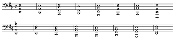
図 2 長調の和声
