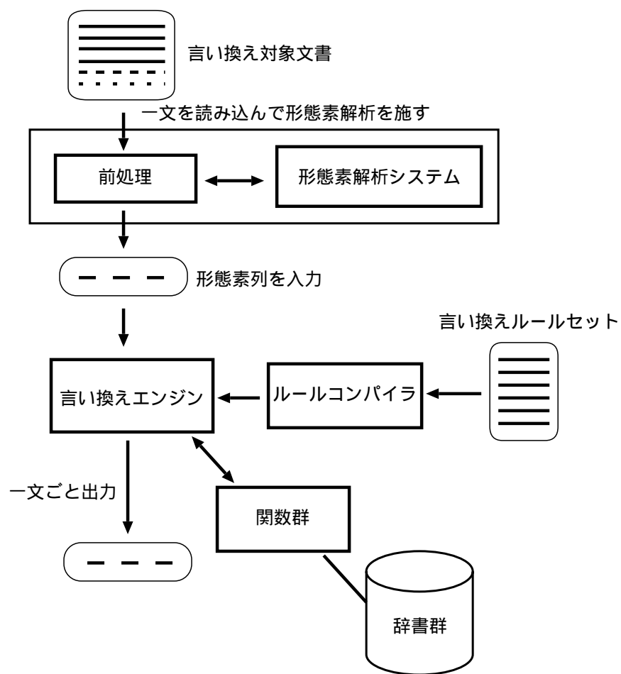
図 3.1: 言い換えシステムの概要
