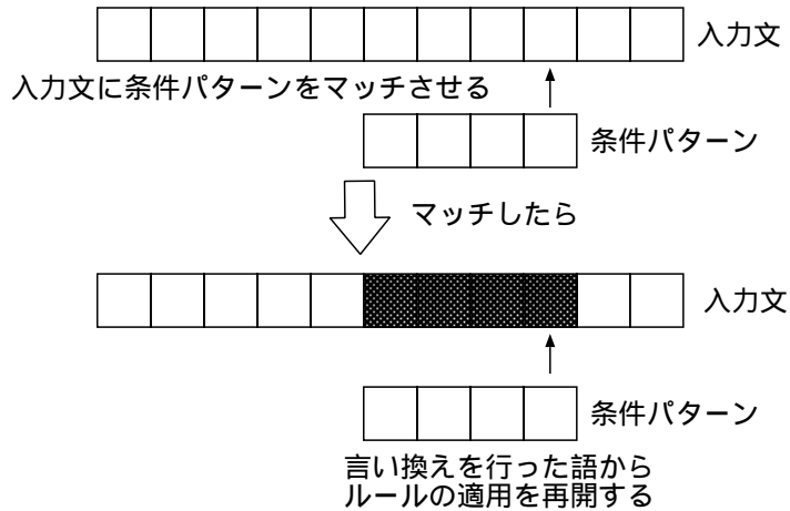
図 3.5: 走査方法が backward で再開位置が local のケース
