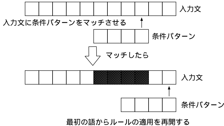
図 3.6: 走査方法が backward で再開位置が global のケース
