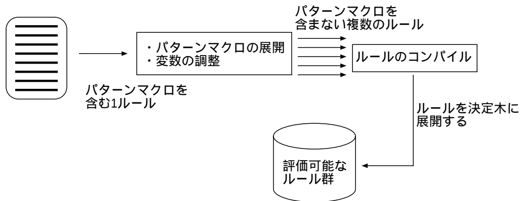
図 3.7: ルールコンパイラ
