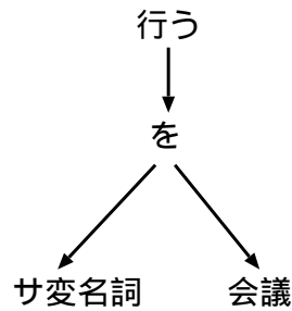
図 3.9: 決定木の例
