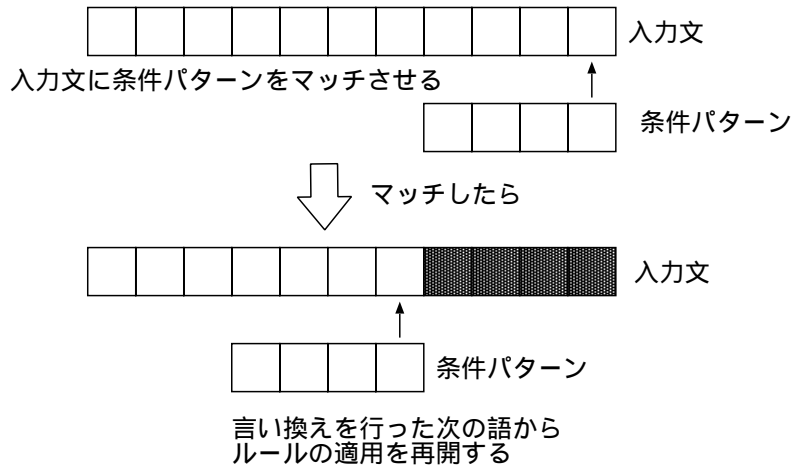
図 3.4: 走査方法が backward で再開位置が skip のケース
