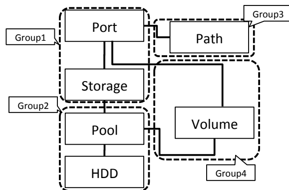
図 4.3: グループ化の一例
