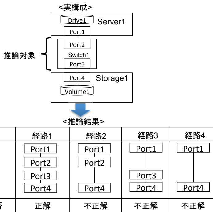
図 6.9: 推論結果の例
