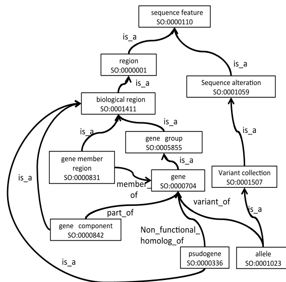
図 2 SO で提供されている遺伝子と関連概念の相互関係
