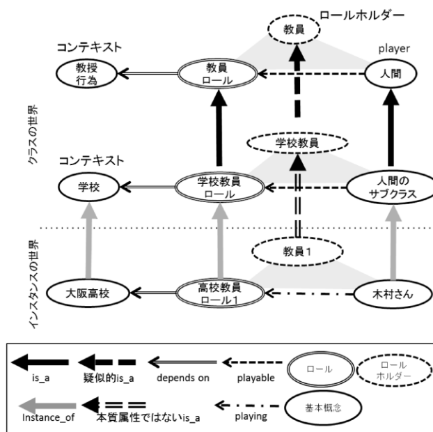
図4 ロールの基本モデル (Mizoguchi 2012 から改変)
