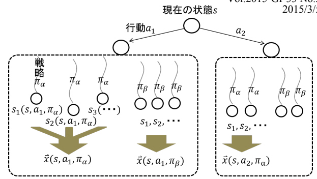
図 2 効用要素推定器の全体像
