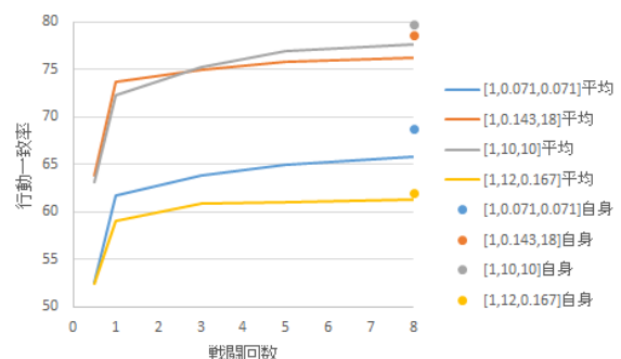
図 6 行動一致率・設定別
