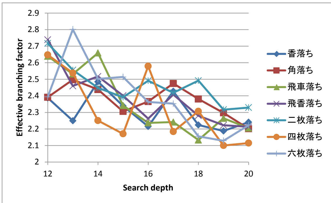
(b) ウインドウを [-\infty, 0] にした探索における有効分岐因子
