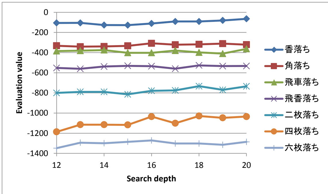
(a) ウインドウを [-\infty, 0] にした探索における評価値
