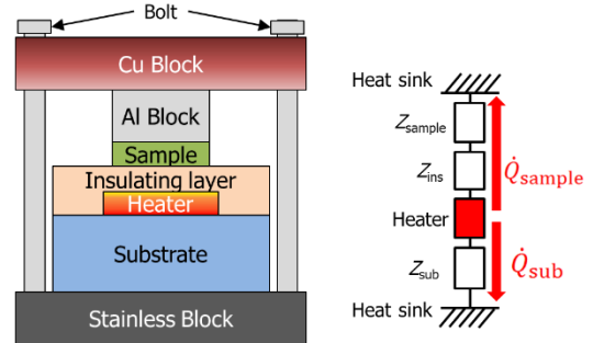
図2 二方向熱流モデルの模式図
