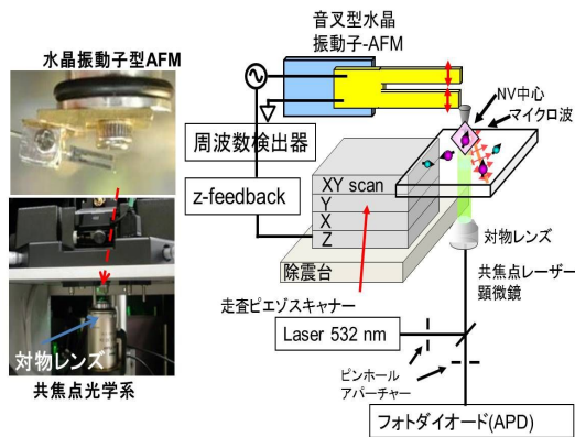
図2、共焦点レーザー蛍光顕微鏡、水晶振動子型AFM、NV中心プローブの複合装置
