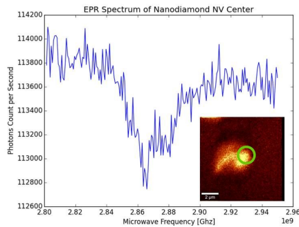
図4、ナノダイヤモンド粒子中の少数 NV 中心から得られた磁気共鳴信号
