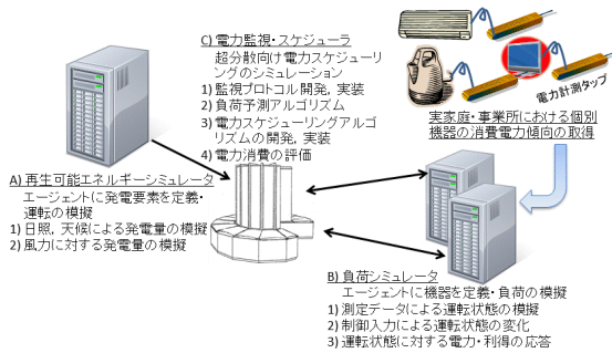
図 2 本提案の実施イメージと構築するシミュレーションシステム
