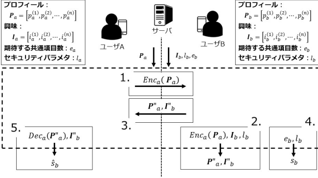
図 3.3: BVT プロトコルの全体像
