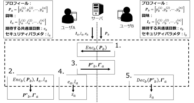
図 3.3: BVT プロトコルの全体像
