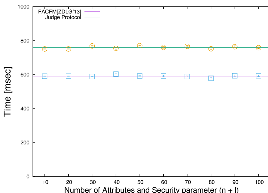
図 5.2: FACFM プロトコル [31] と閾値判定プロトコルの実行時間
