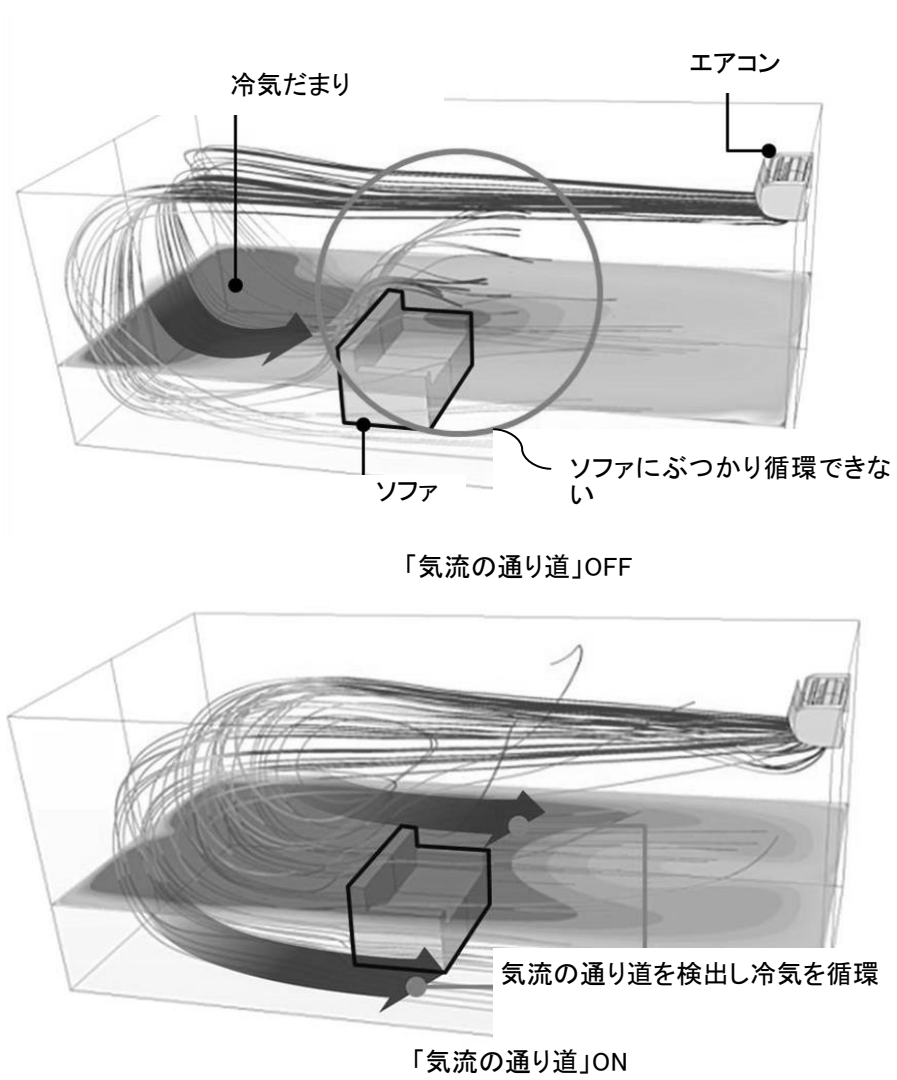
図 22 冷房運転時の「気流の通り道」
