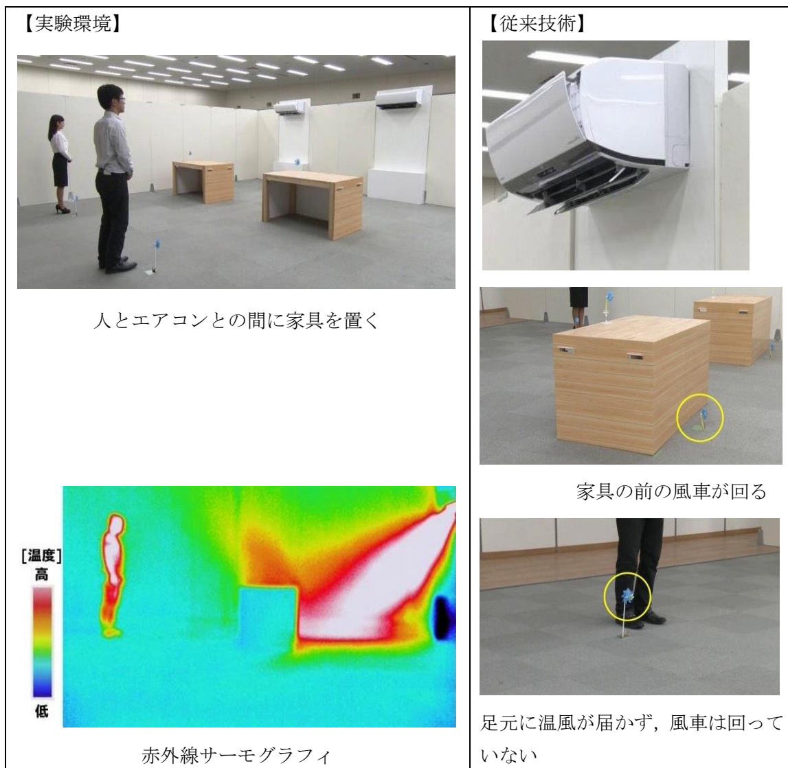
図 25 気流の通り抜けない家具がある場合(従来技術)
