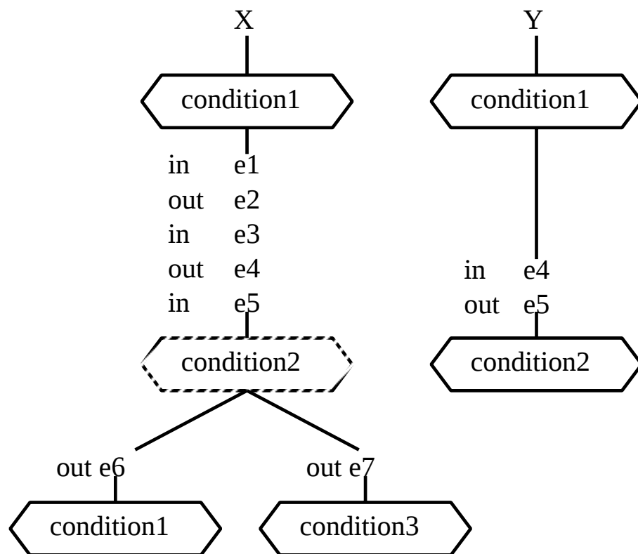
図 4.12: 各オブジェクトごとのイベント列
