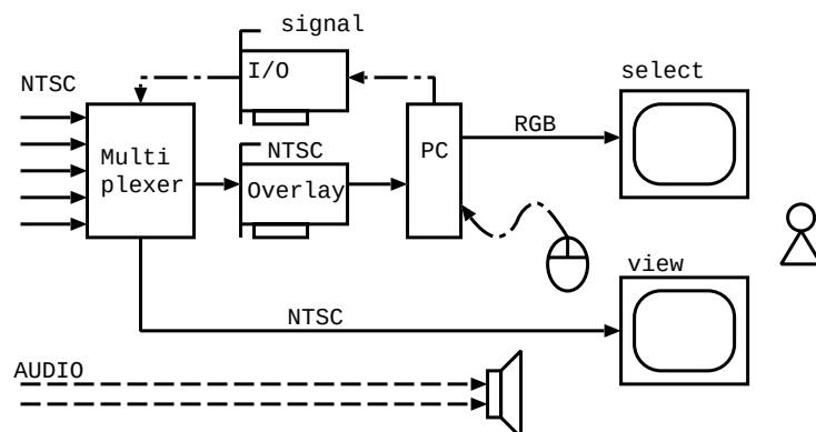
図 4.1: UI
