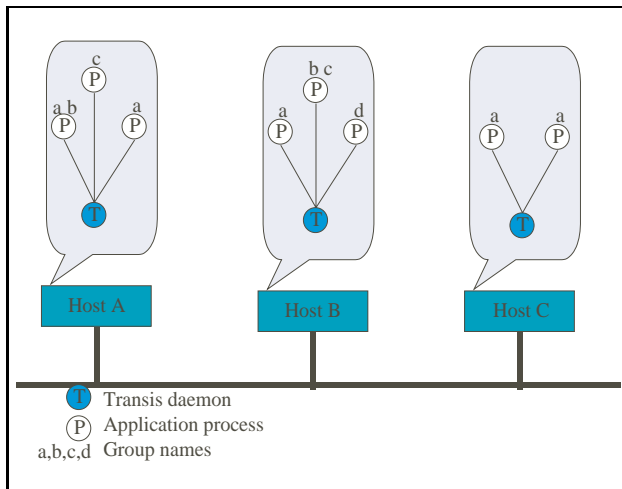
図 3.3: Transis システム
