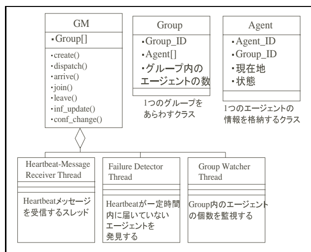
図 5.1: GM の構成
