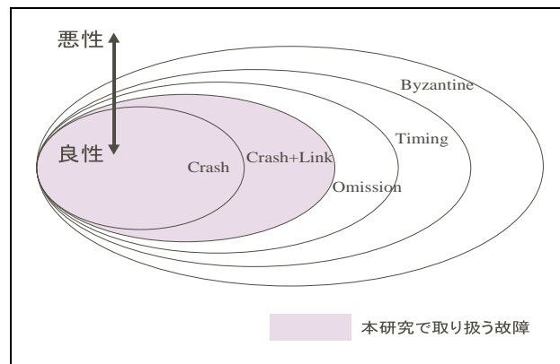
図 4.2: 故障モデル
