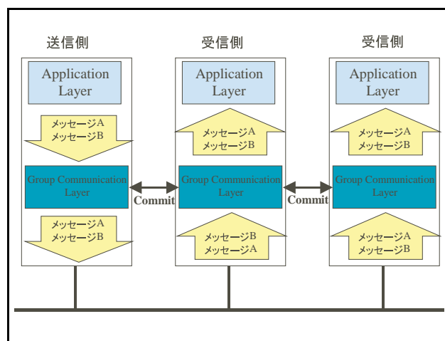
図 3.2: 仮想同期
