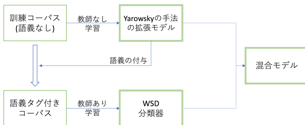
図 5.1: 教師あり機械学習と教師なし機械学習の併用
