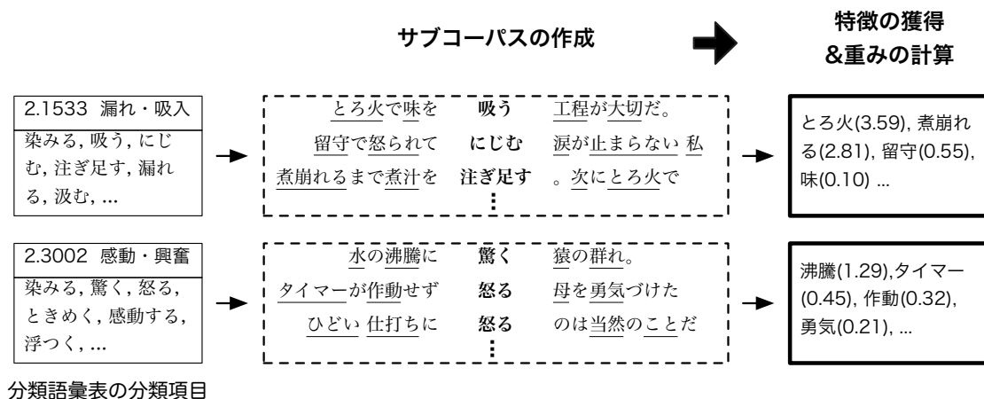
図 3.1: Yarowsky の手法 [9] の概要
