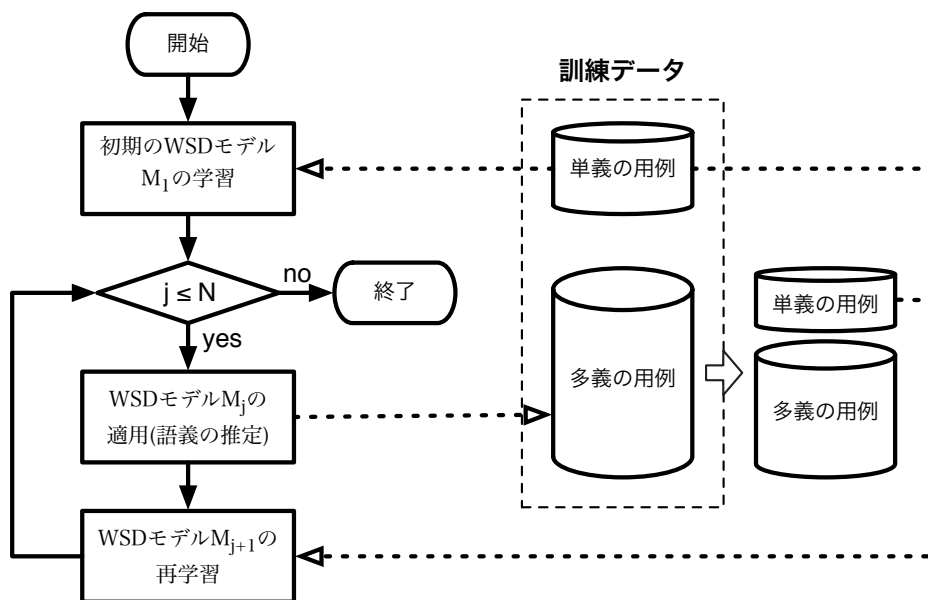
図 3.7: 語義推定モデル
