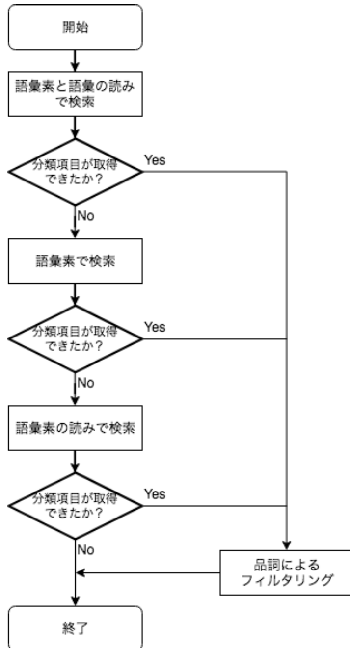
図 3.9: 分類項目の辞書引きの手続き
