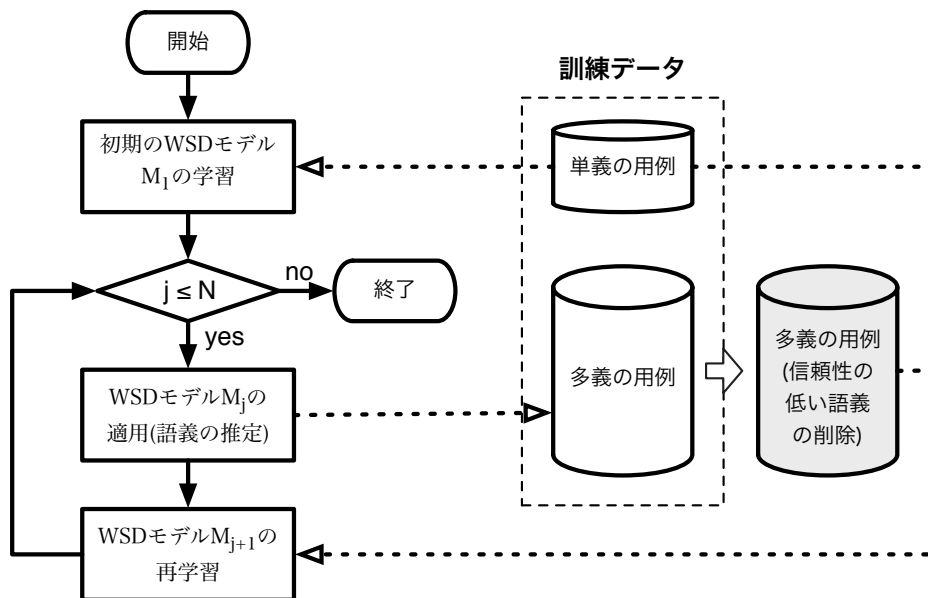
図 3.8: 語義絞り込みモデル
