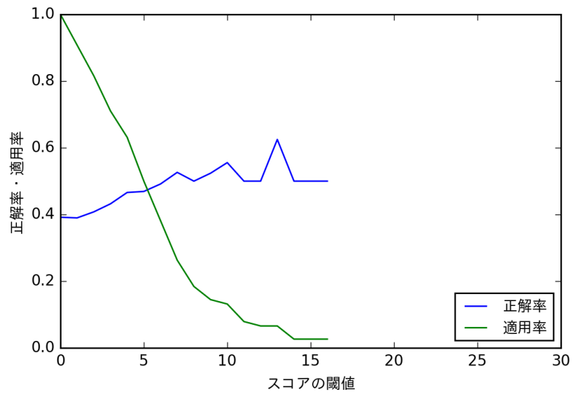
図 4.4: Yarowsky のモデルの正解率と適用率 (その他)
