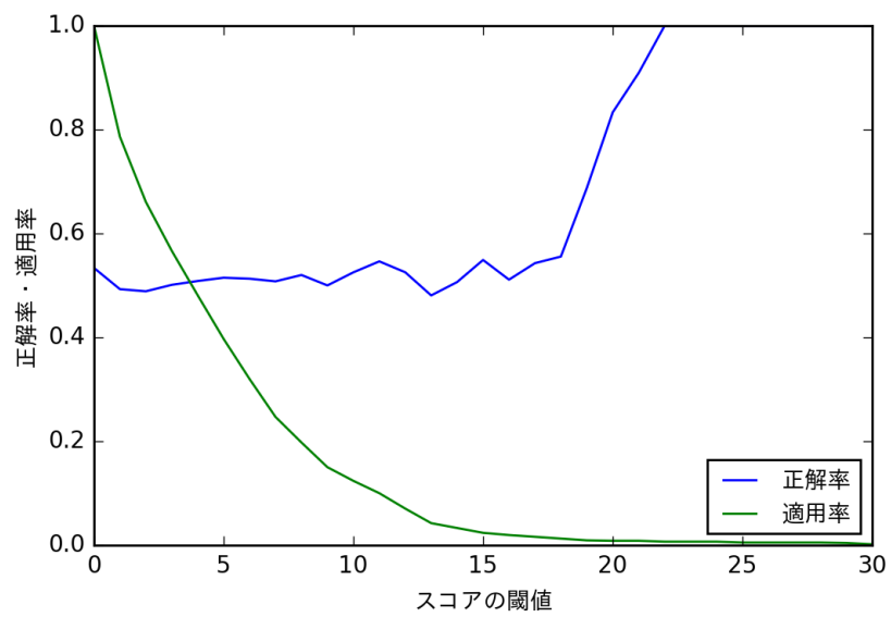
図 4.2: Yarowsky のモデルの正解率と適用率 (名詞)
