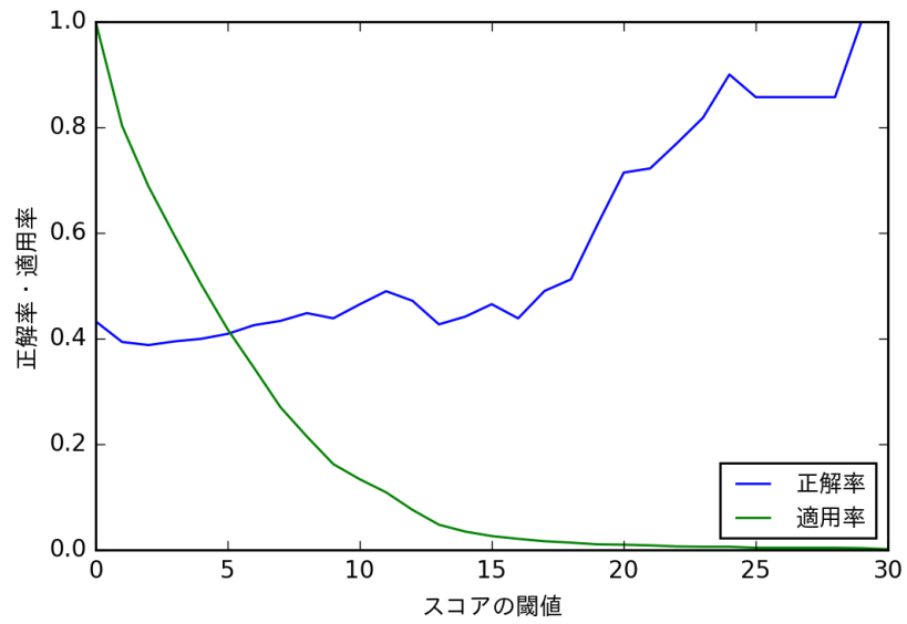
図 4.1: Yarowsky のモデルの正解率と適用率 (全品詞)
