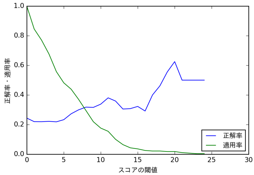
図 4.3: Yarowsky のモデルの正解率と適用率 (動詞)
