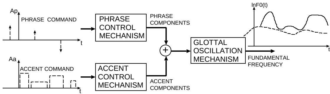
図 3.1: 藤崎 F0 モデルの概要
