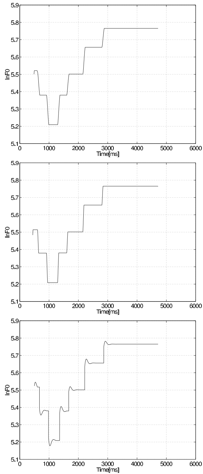
図 3.13: 合成音の F0. 上から POLTA1、POLTA2、OUS の F0 を表す
