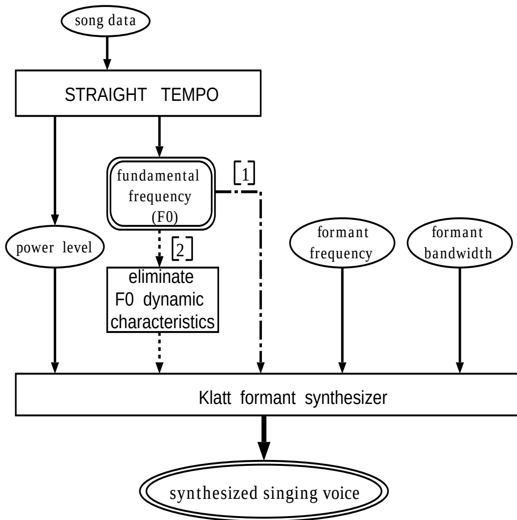
図 2.4: F0 動的変動成分を除去した合成音の作成手順
