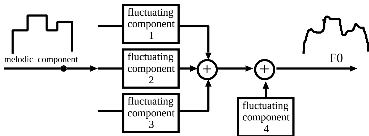
図 3.3: 本研究で提案した F0 制御モデルの概要
