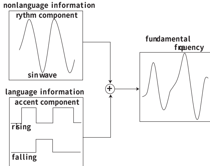
図 3.1: 藤崎 F0 モデルの概要
