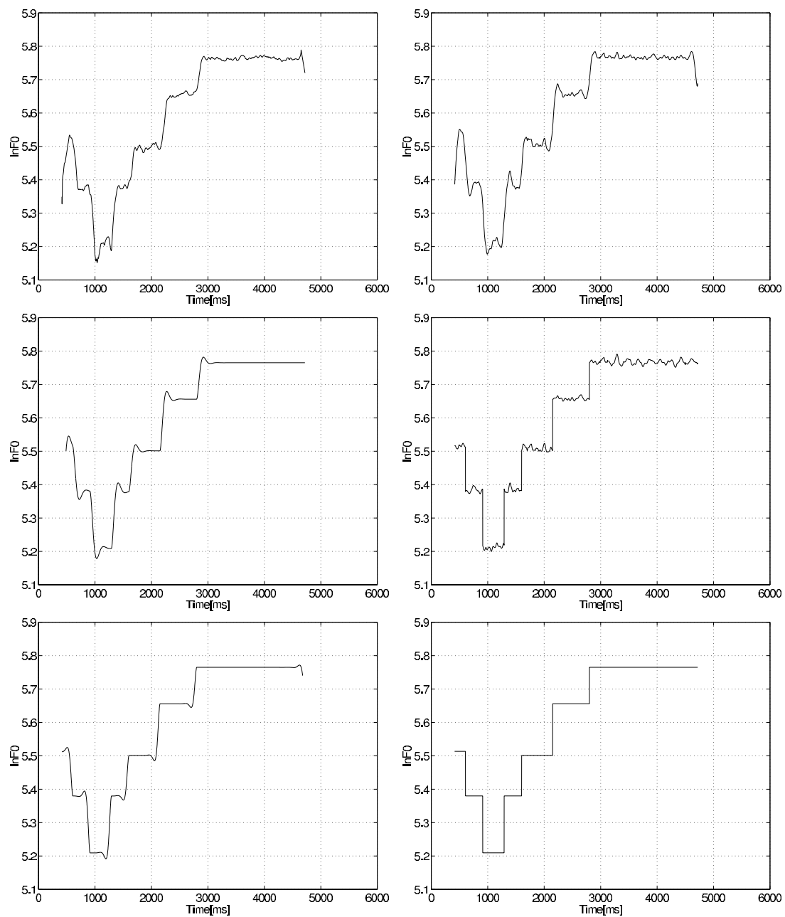
図 3.11: 歌声合成に用いた F0. 上段の左から順に NORMAL, SYN-ALL. 中段 SYN-OUS, SYN-VB. 下段 SYN-PRE, SYN-BASE の F0 を示す
