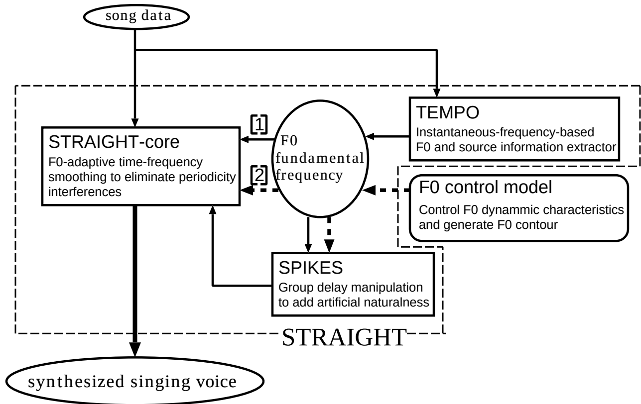
図 3.15: STRAIGHT の構成と歌声合成の手順
