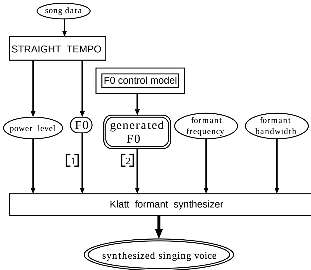
図 3.10: 歌声合成の手順 (Klatt Formant Synthesizer)
