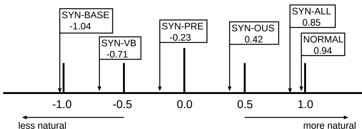
図 3.16: 合成音の自然性の関係
