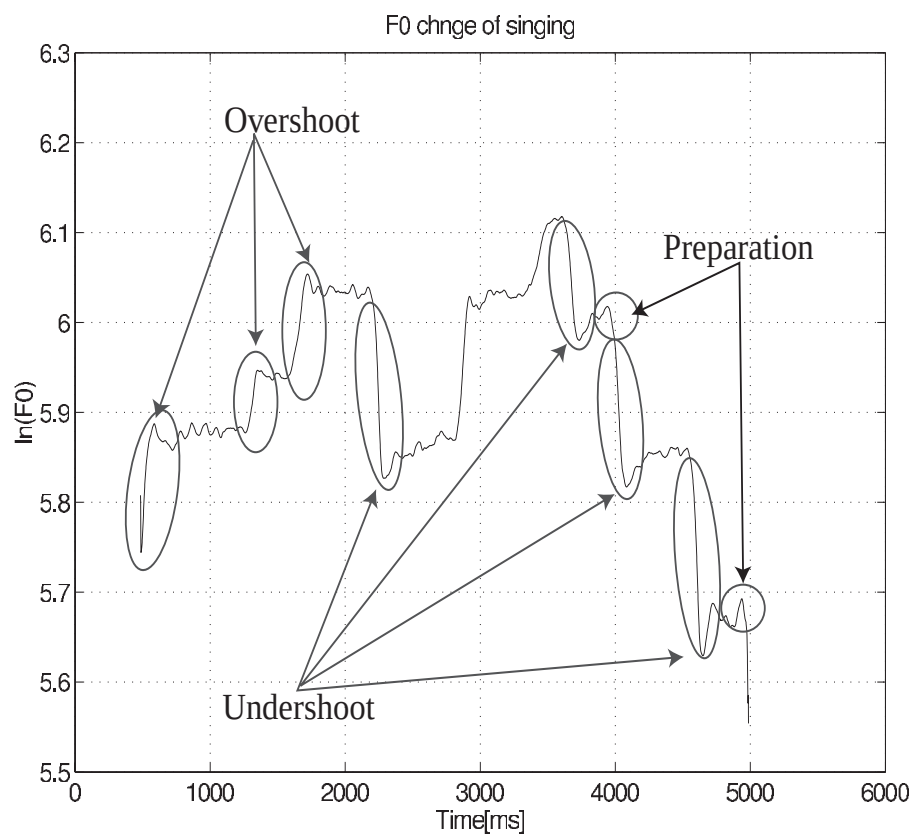
図 2.2: F0 中の動的変動成分 1
