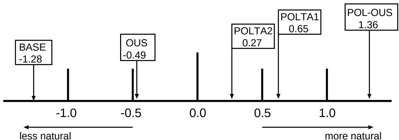
図 3.14: 歌声刺激の自然性の関係
