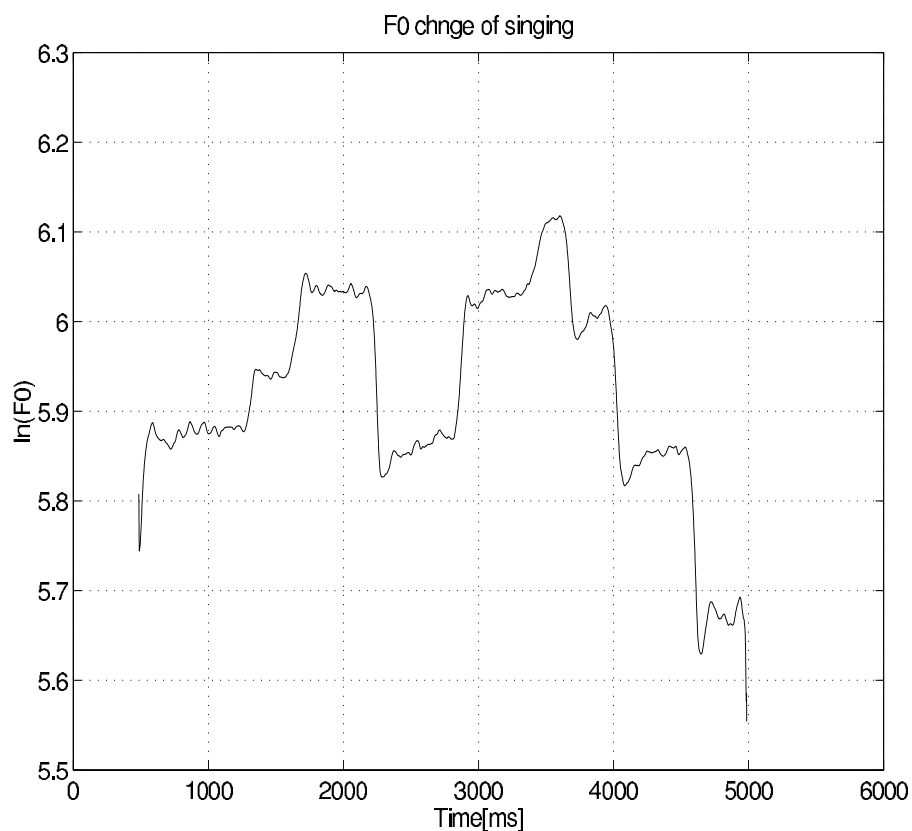
図 2.1: “かわいい七つの” 歌唱時の F0
