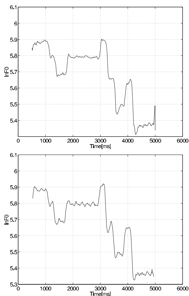
図 3.6: 「カラスなぜなくの」歌唱時の、上：実音声の F0, 下：モデルで生成した F0
