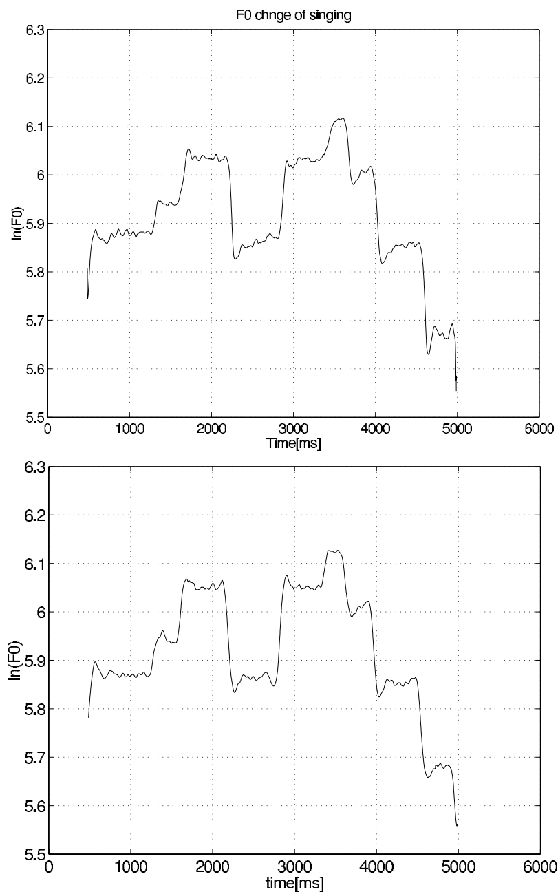
図 3.8: 「かわいい七つの」歌唱時の、上：実音声の F0, 下：モデルで生成した F0
