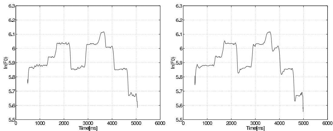
図 2.5: 左:オーバータラゲット、アンダータラゲットを除去した F_0(\text{NO-OUS}) 、右:ヴィブラート・微細変動を除去した F_0(\text{NO-VB})
