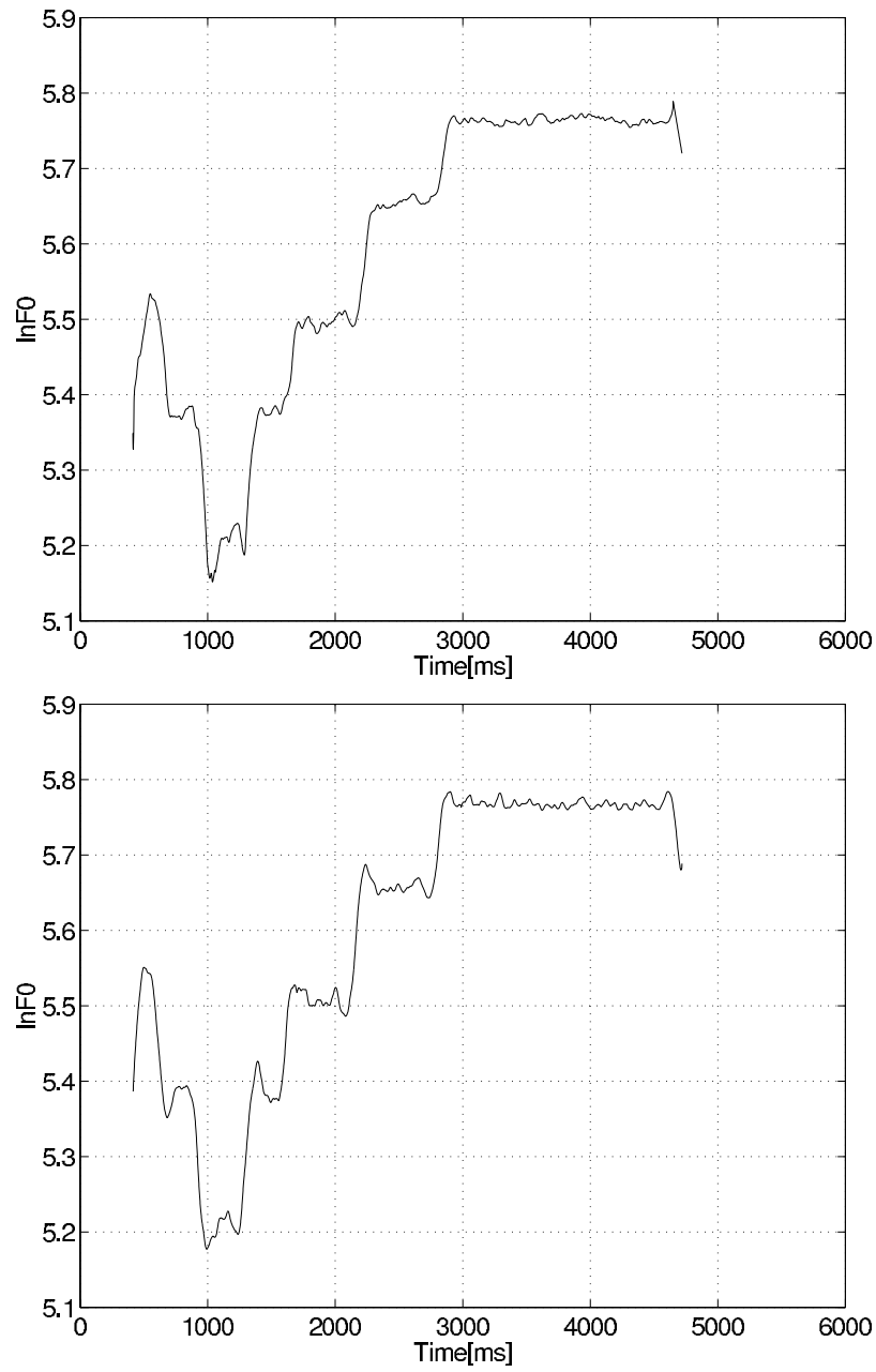
図 3.7: 「カラスは山に」歌唱時の、上：実音声の F0, 下：モデルで生成した F0
