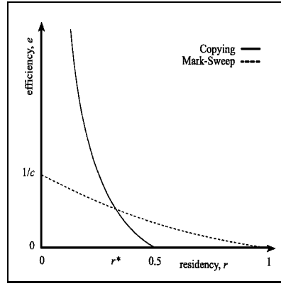
図 7.1: 効率とプログラムとメモリの占有率の関係
