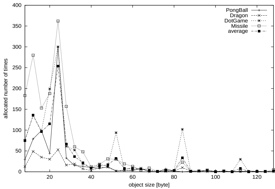
図 4.3: 大きさ 0~128byte のオブジェクトと回数の関係
