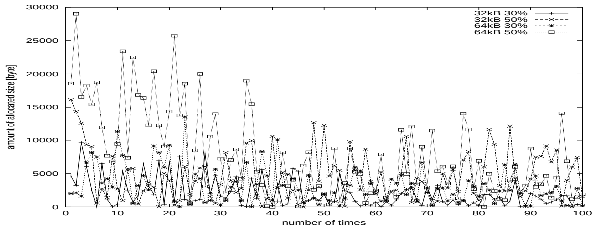
図 5.2: First fit 法のシミュレーション結果
