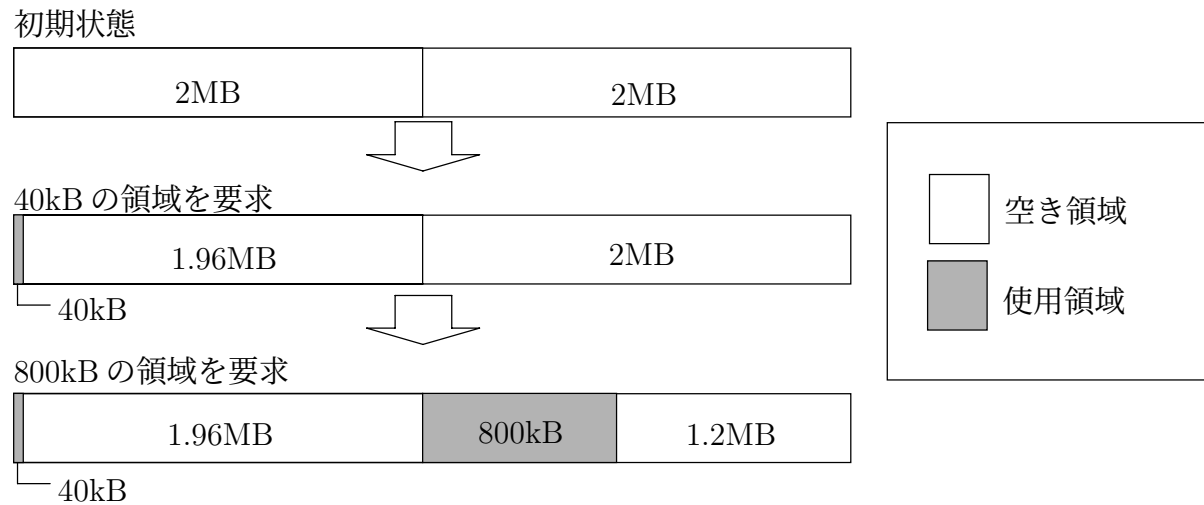
図 3.7: Separate first fit 法
