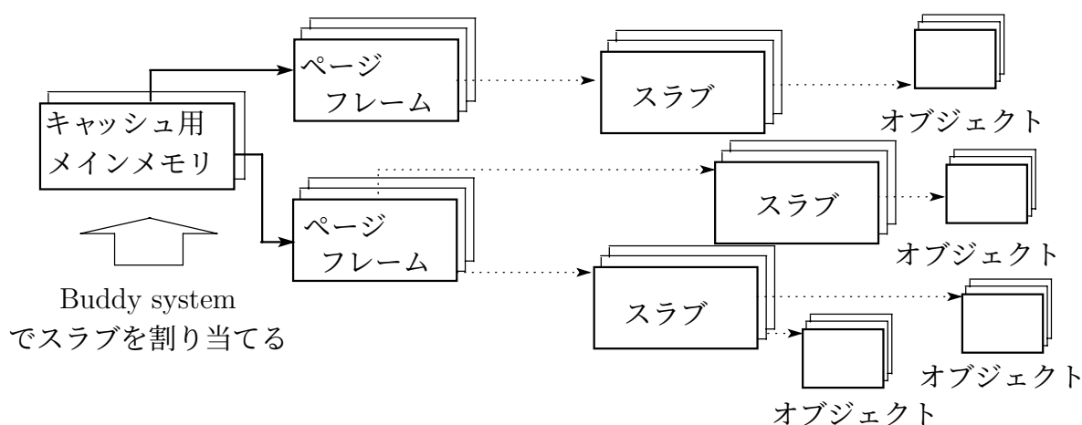
図 2.5: スラブアロケータの構成
