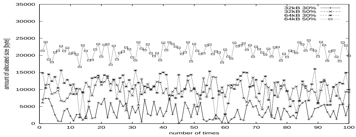
図 5.4: Block buddy system のシミュレーション結果
