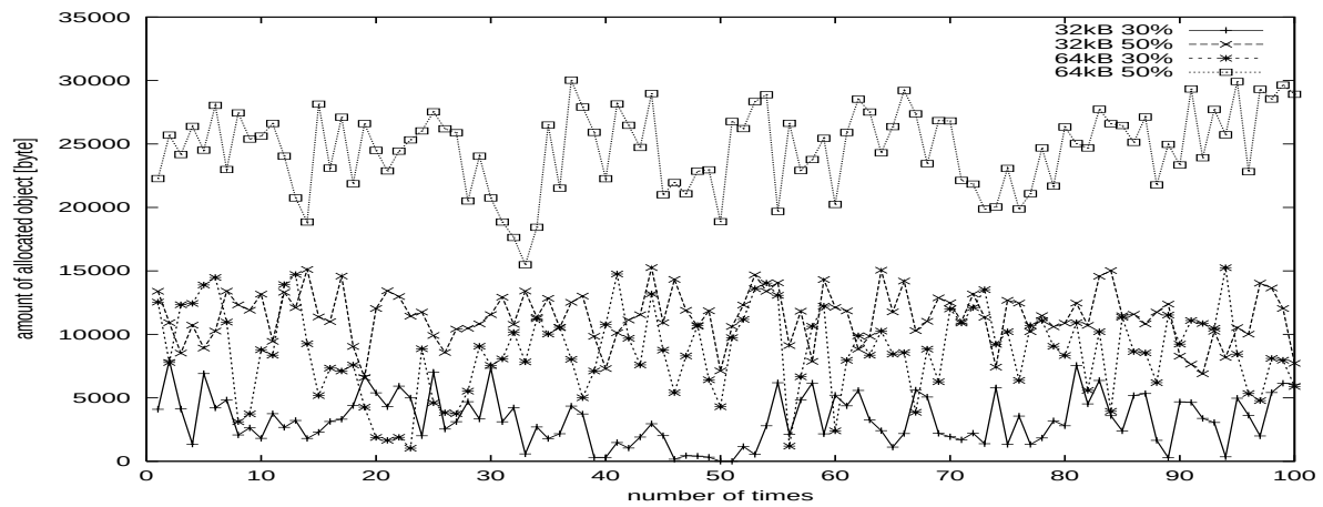
図 5.3: Separate first fit 法のシミュレーション結果
