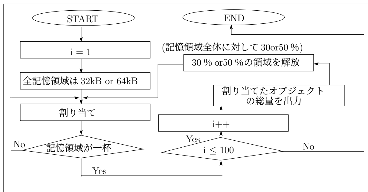
図 5.1: シミュレーションのアルゴリズム
