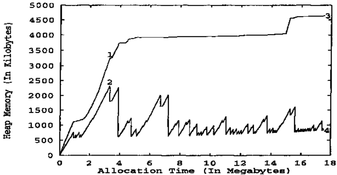
図 6.1: GCC のメモリ使用量
