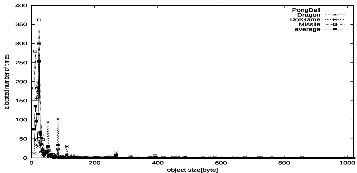
図 4.2: 割り当てられたオブジェクトの大きさと回数の関係
