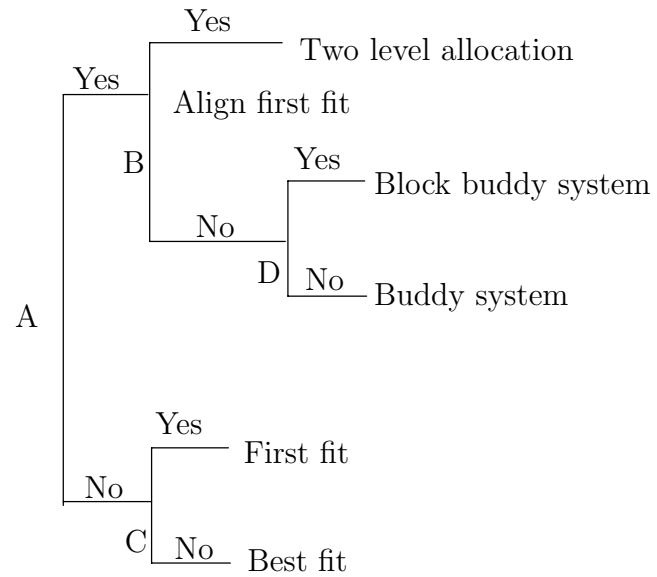
図 5.5: 割り当て方法の選択
