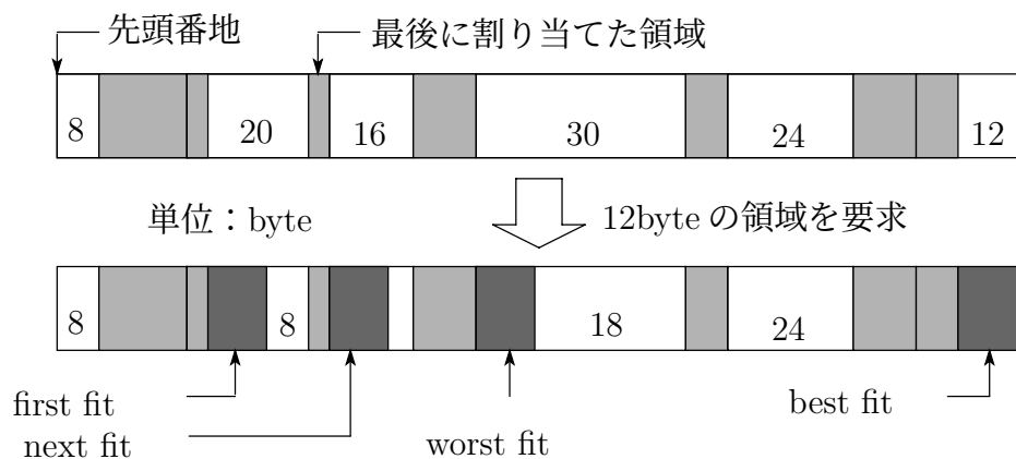
図 2.1: 各 Fit 法の空き領域の探索方法
