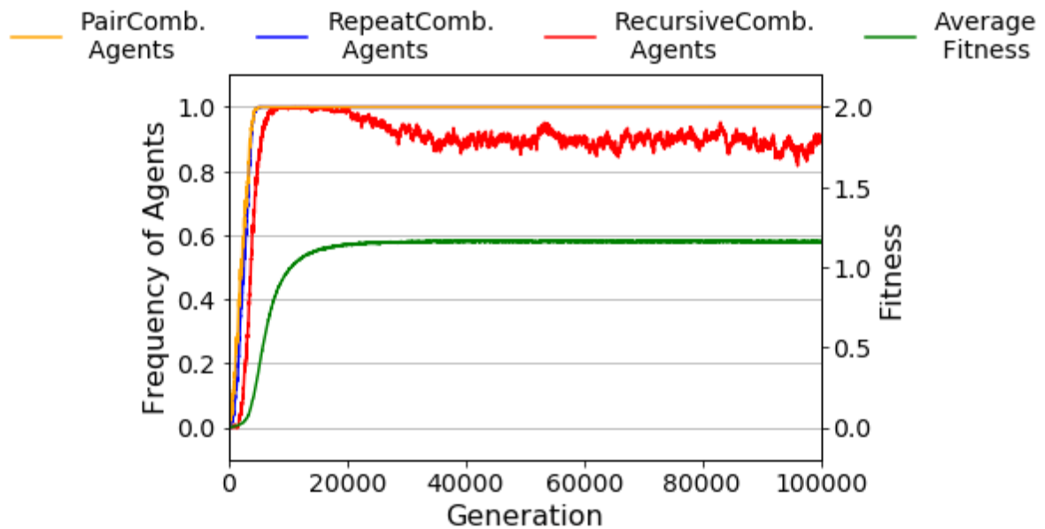
図 3.16 各結合を使用するエージェントの割合と適応度の世代変移 ( F_{IV} , 200 試行の平均)
