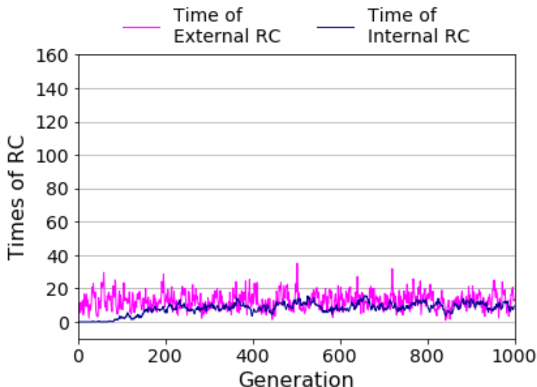
図 4.5 エージェント一個体あたりの再帰的結合の使用回数の世代変移 ( R_t , 1 試行)
