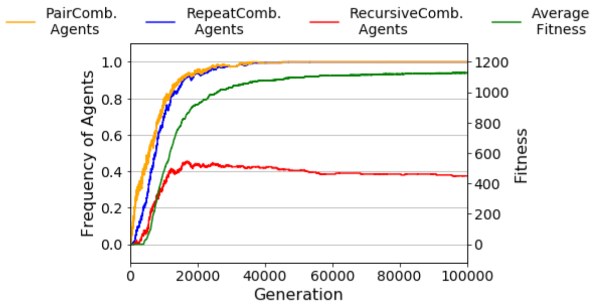
図 3.7 各結合を使用するエージェントの割合と適応度の世代変移 ( F_{II} , 200 試行の平均)
