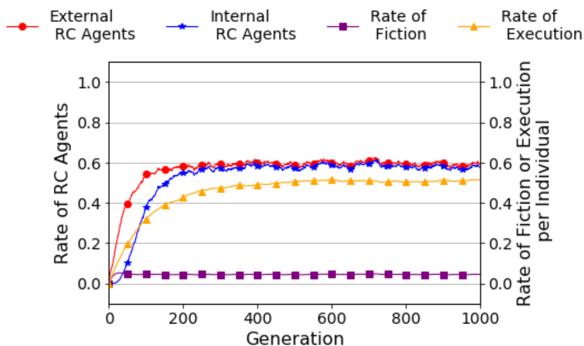
図 4.3 再帰的結合を使用するエージェントの割合と表象操作確率の世代変移 ( R_1 , 200 試行の平均)
