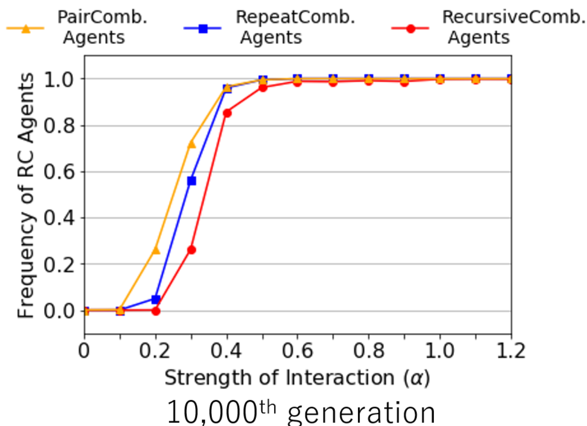
図 3.18 資源獲得競争の強さごとの各結合を使用するエージェントの割合 ( F_{IV} , 200 試行の平均. 10,000 世代目)
