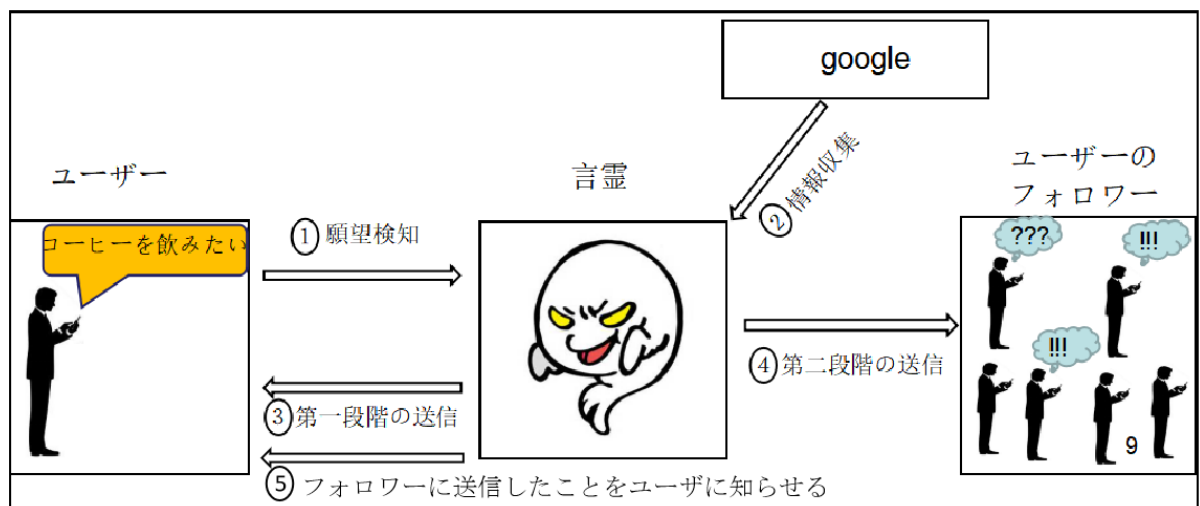
図 3. 2 「言霊テロ」システムの処理の流れ
