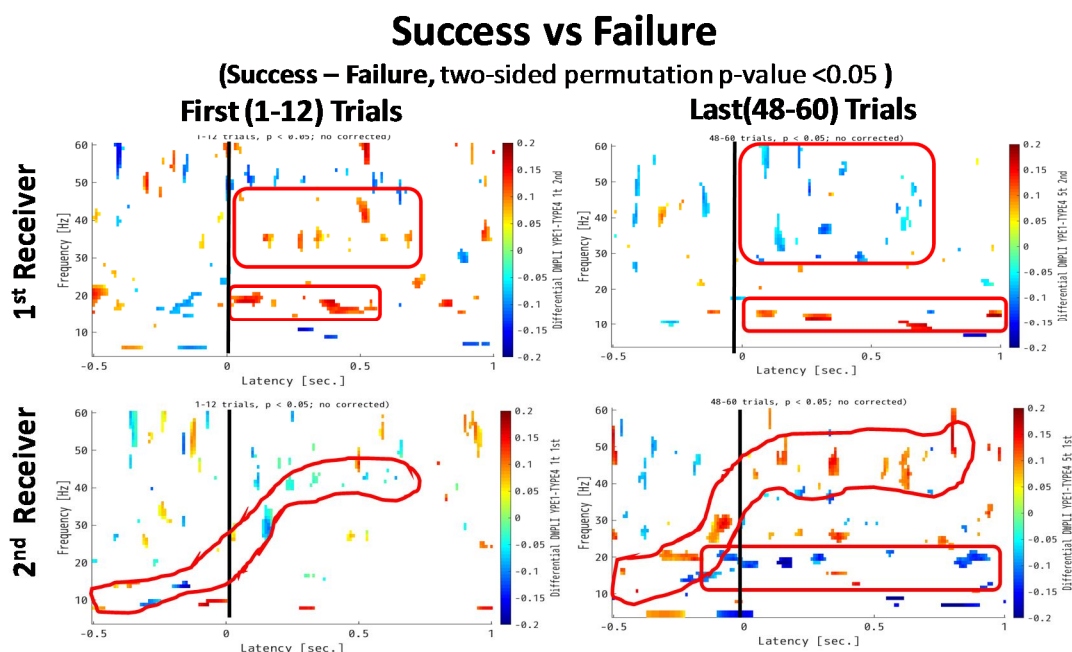
図 2 受信時の脳波位相同期 (DWPLI) スペクトルの変化．意図共有群と失敗群の全参加者・全チャンネル間の脳波位相同期の平均の差が有意な部分のみ表示．上段：後手送信群，下段：先手送信群，左列：初期，右列：終期．横軸：受信からの潜時，縦軸：周波数帯．
