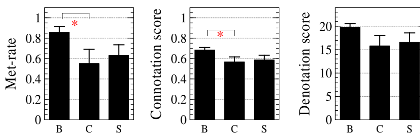
図 3 左から、課題成功率、言外の意味の理解率、字義的意味の理解率．横軸：有意なミュ波抑制が両方 (B), CG のみ (C), SG のみ (S)
