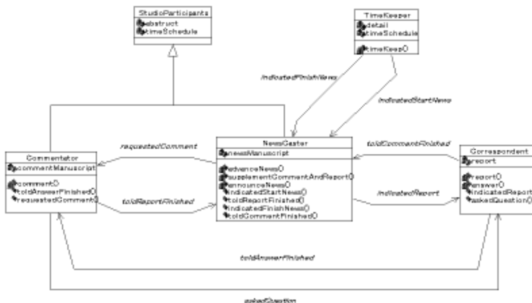
図 5.6: ニュース放送システムのクラス図
