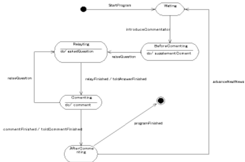
図 5.9: Commentator の状態チャート図
