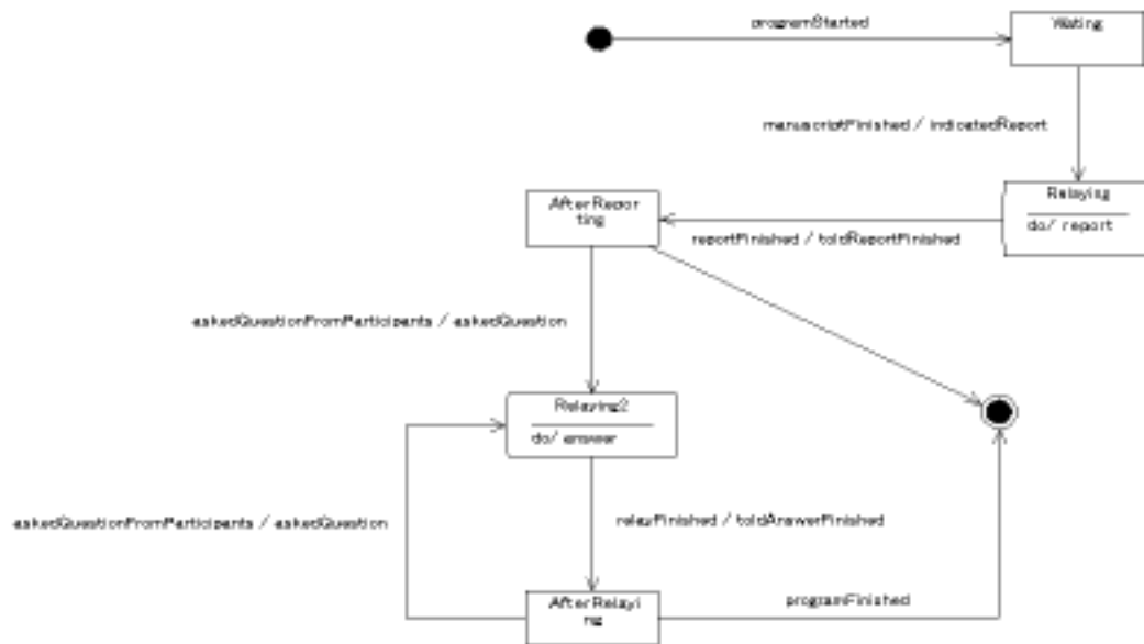
図 5.10: Correspondent の状態チャート図
