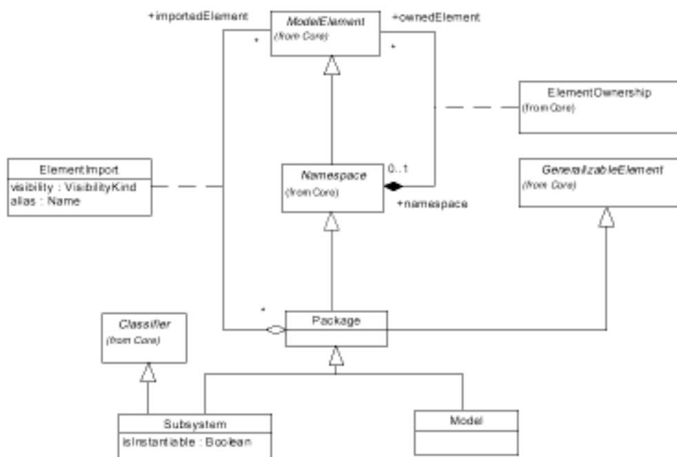
图 A.15: Model Manegement
