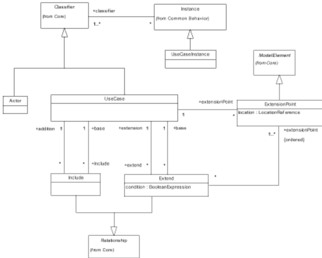
图 A.11: Use Cases
