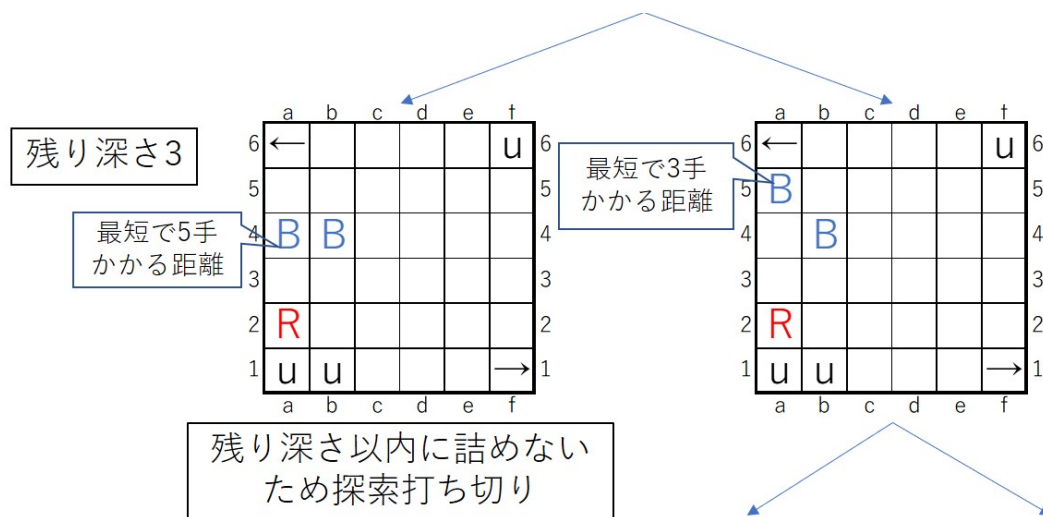
図 5.4: 探索打ち切り例
