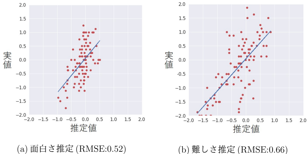
図 7.5: 面白さ，難しさ推定
