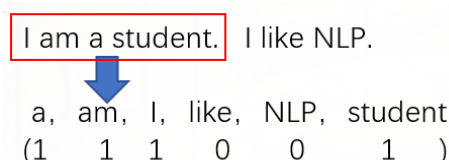
図 1.1 : Word2Vec の例
