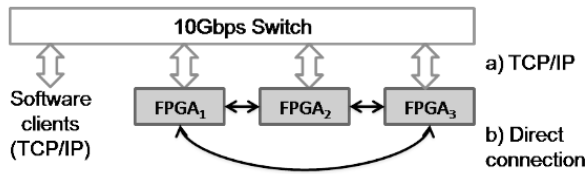
図 5 István らによる FPGA SmartNIC への ZAB 実装[34]
