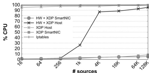
図 3 Miano らによる評価(ホスト CPU 利用率)[23]
