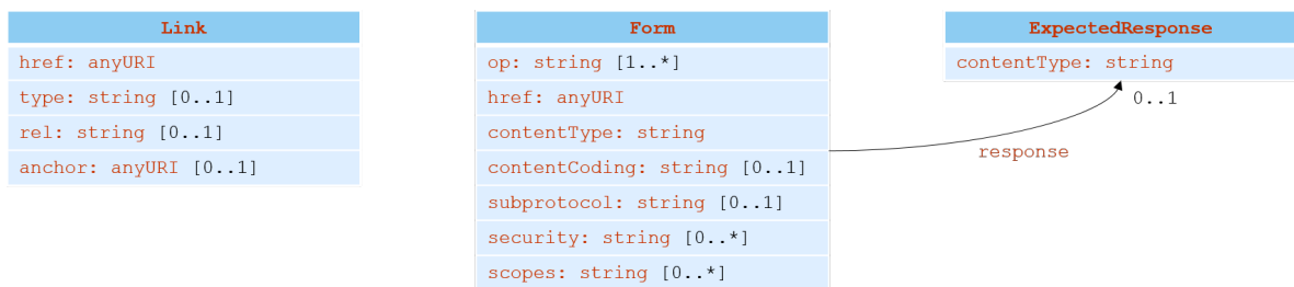
図 2.23 Hypermedia controls vocabulary[18]
