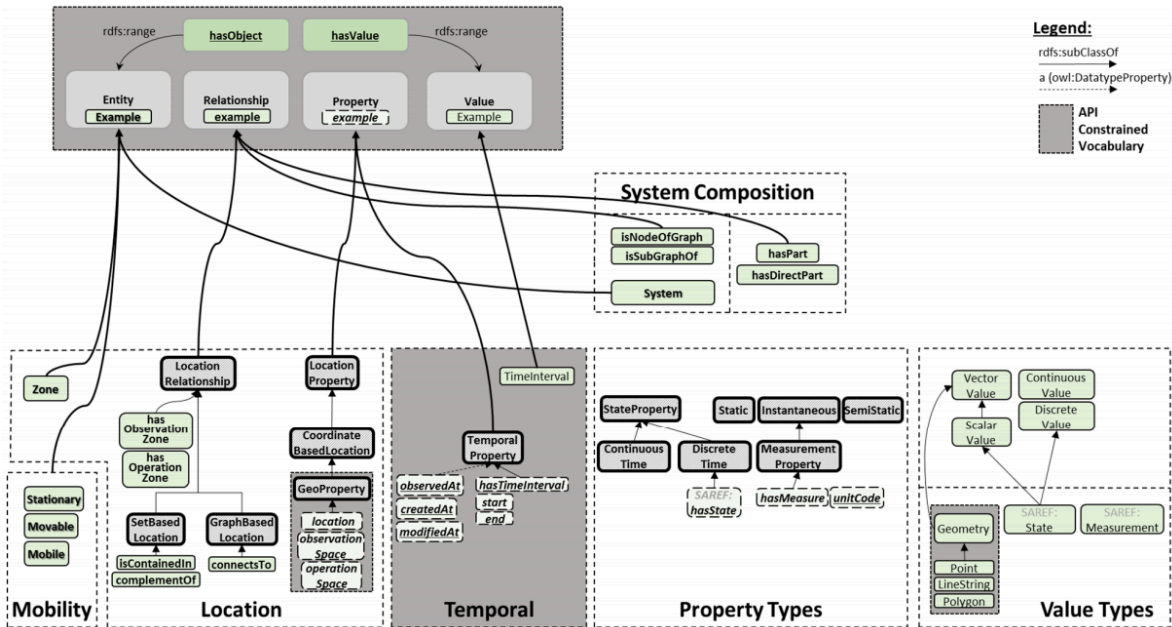
図 2.15 NGSI cross-domain model[17]
