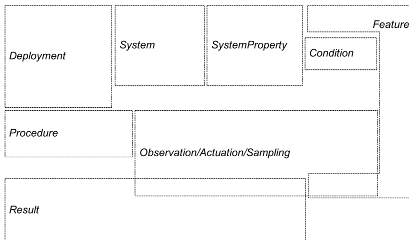
図 2.28 SSN OntStructure Overview[23]
