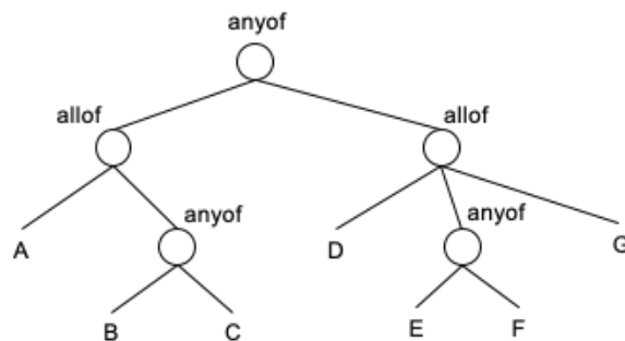
図 4.10 論理式をツリーで表す
