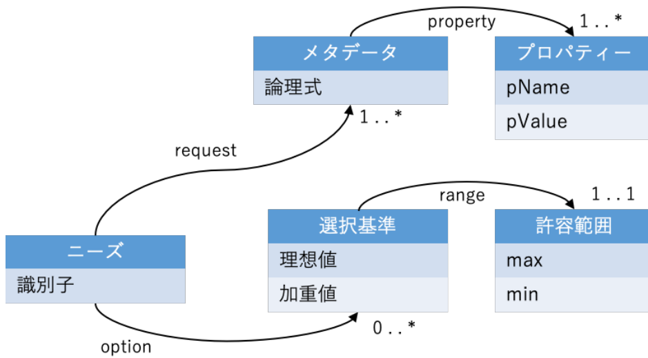
図 4.9 ニーズ記述モデル
