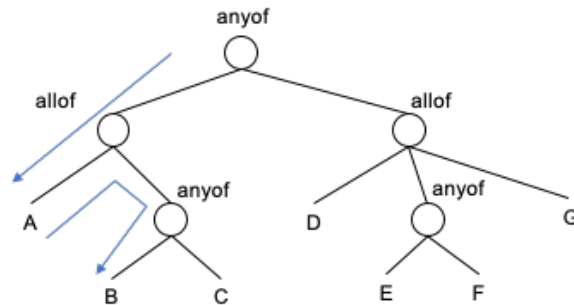
図 5.3 論理式のツリー表現の変換
