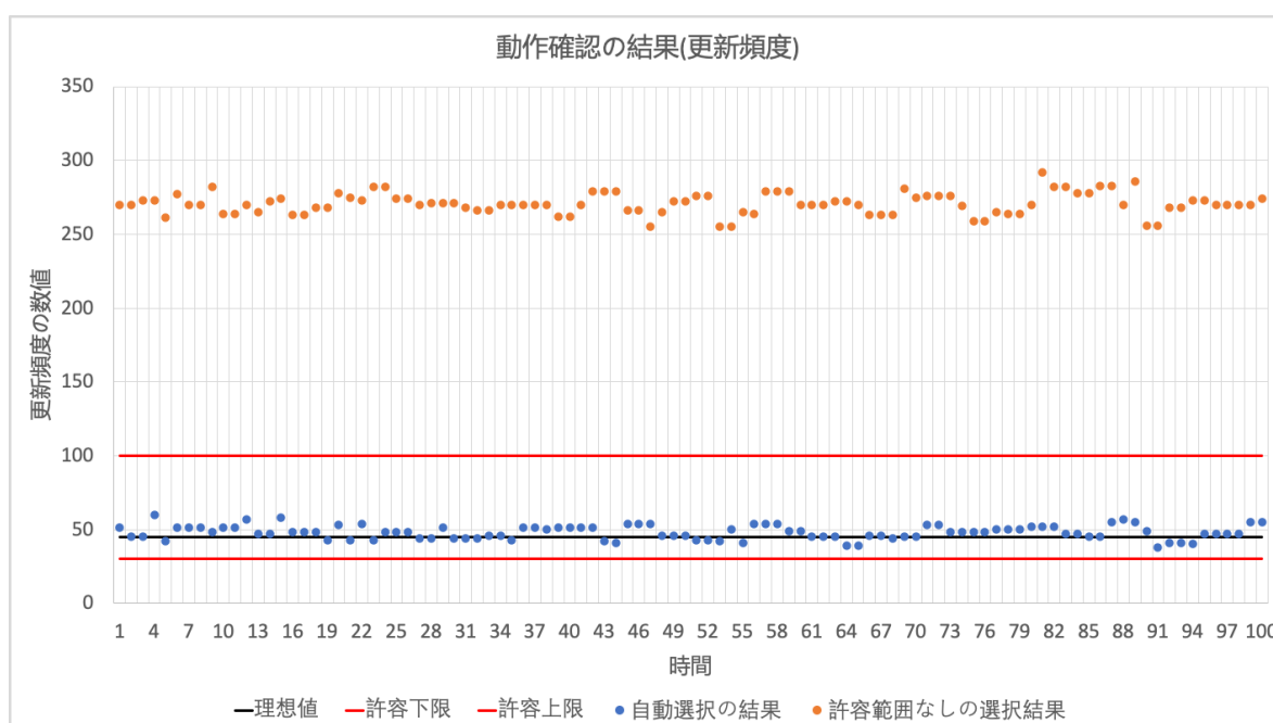
図 6.2 動作確認結果 (提供頻度, 重み=2)
