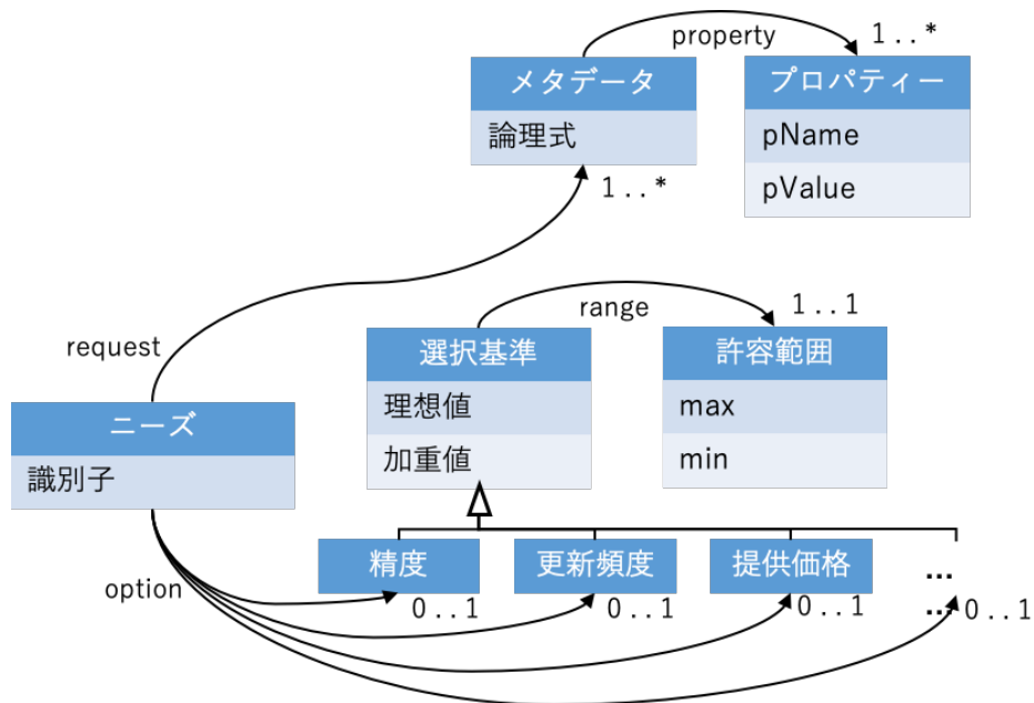
図 5.2 提案システムにおける記述モデル
