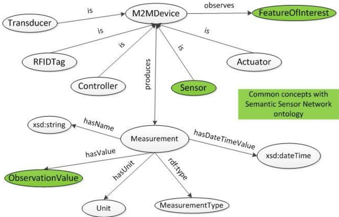
図 2.32 M3 ontology[24]
