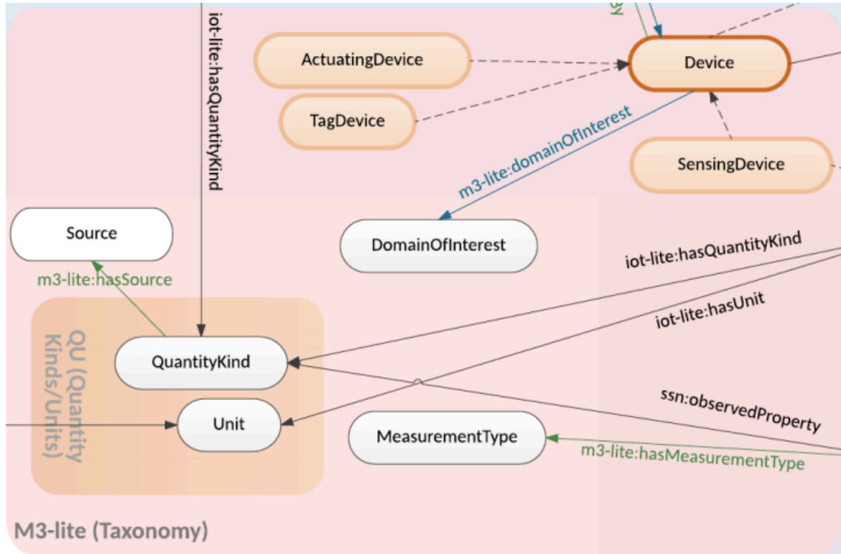
図 2.33 M3-lite モデル [22]
