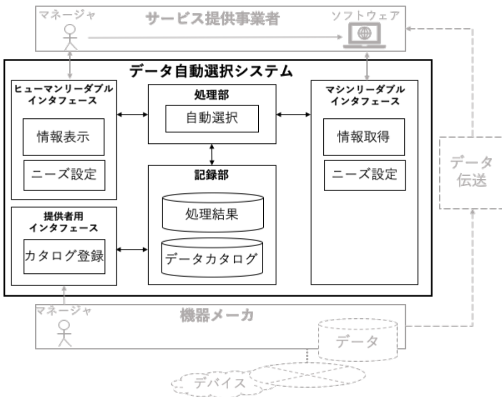
図 5.1 提案システムの実装概要図
