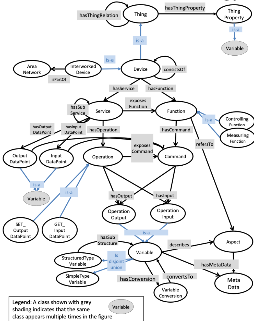
図 2.1 oneM2M Base Ontology[5]
