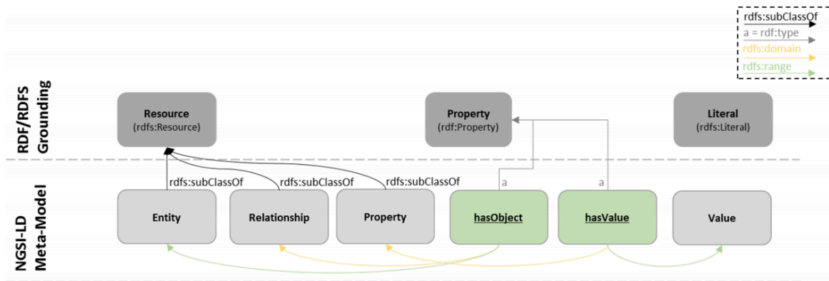
図 2.14 NGSI-LD core meta-model[17]
