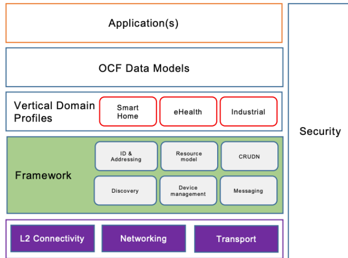
図 2.7 OCF 機能ブロック図 [8]
