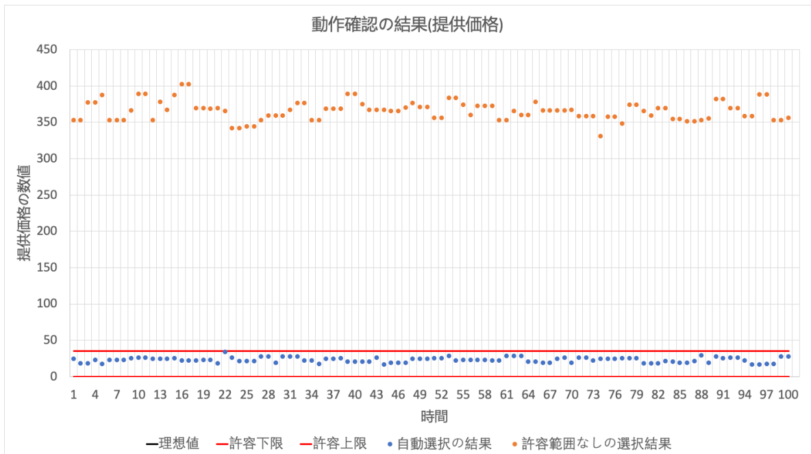
図 6.4 動作確認結果 (提供価格, 重み=1)
