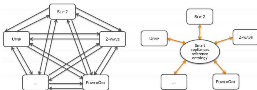
図 2.9 SAREF の位置付け [16]
