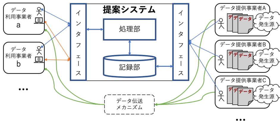
図 4.1 提案システムの全体像
