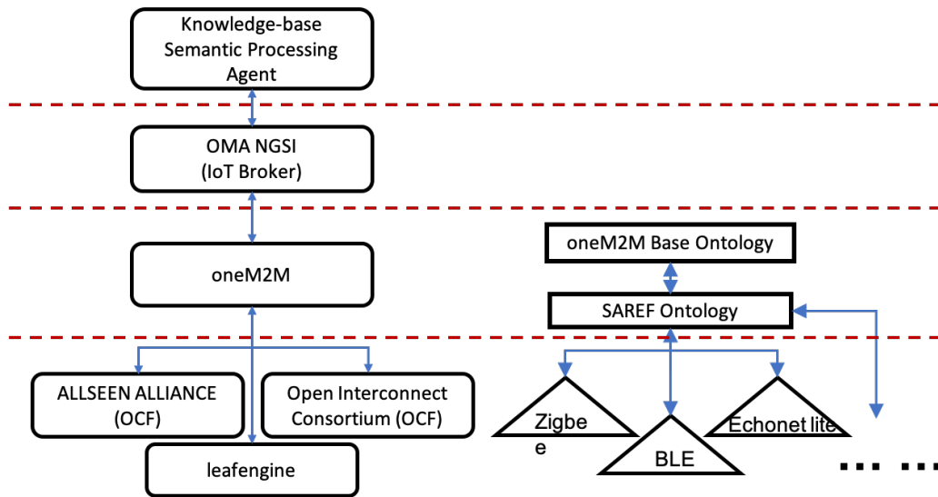
図 2.39 レイヤ構造の比較
