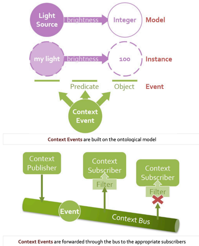
図 2.3 uAAL の Context バス [7]
