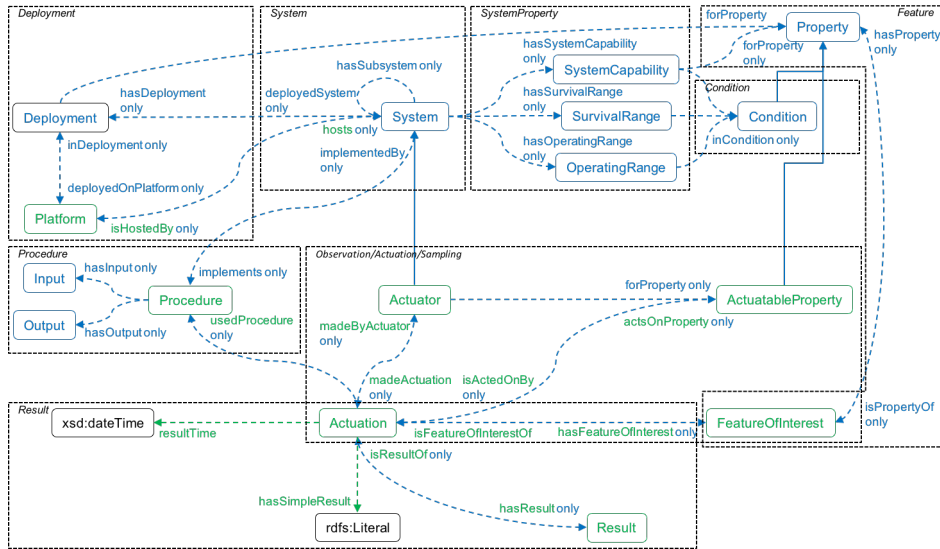
図 2.29 SSN OntStructure Actuation[23]
