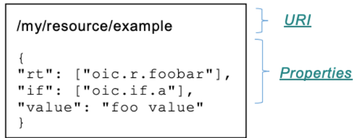
図 2.8 OCF リソースモデルの例 [8]
