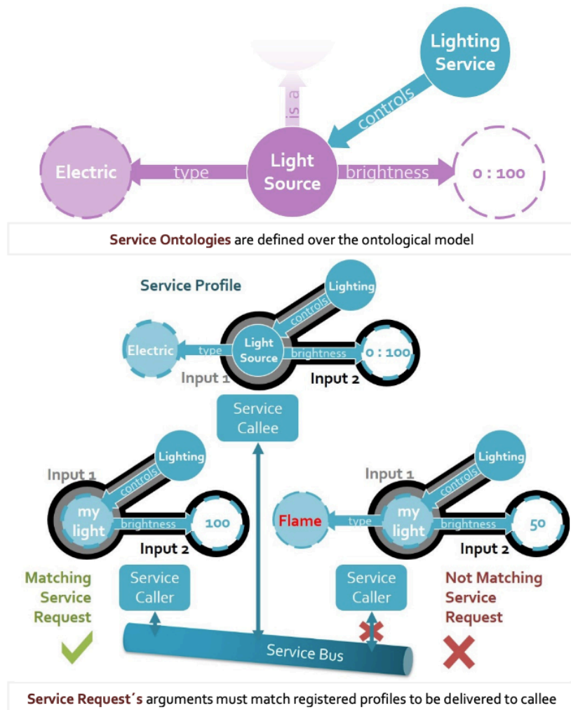
図 2.4 uAAL の Service バス [7]
