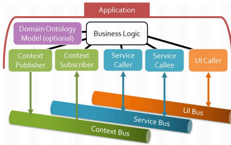
図 2.6 universAAL のバス [7]
