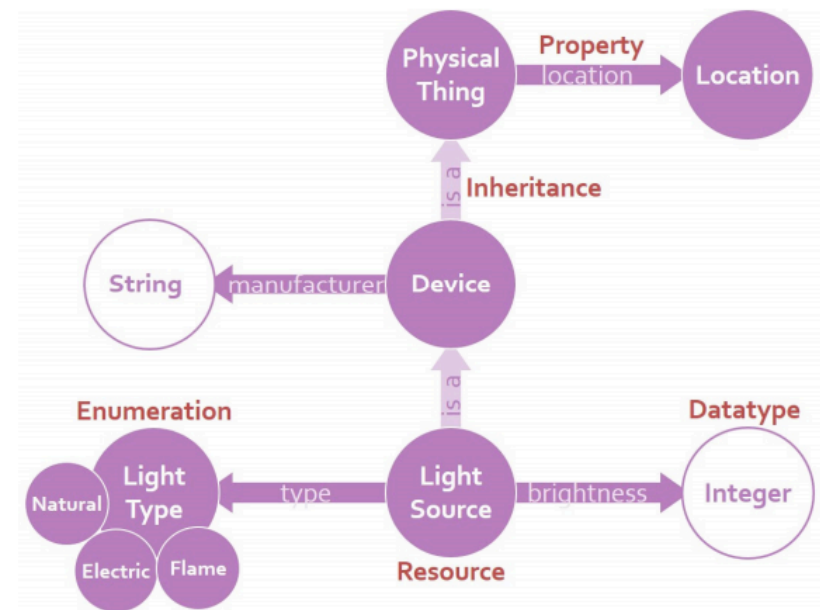
図 2.2 universAAL モデル [7]
