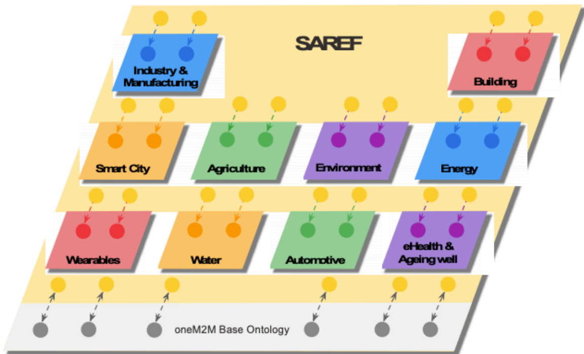
図 2.12 SAREF の拡張 [16]
