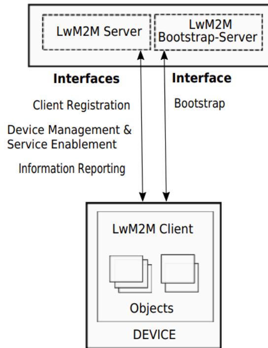
图 2.34 OMA LwM2M 全体像 [25]
