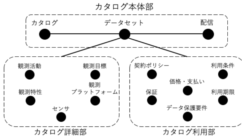
図 4.3 JEITA スマートホームデータカタログのイメージ (クラスレベルまで)
