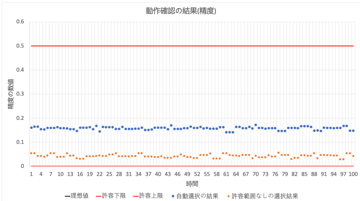
図 6.3 動作確認結果 (精度, 重み=6)
