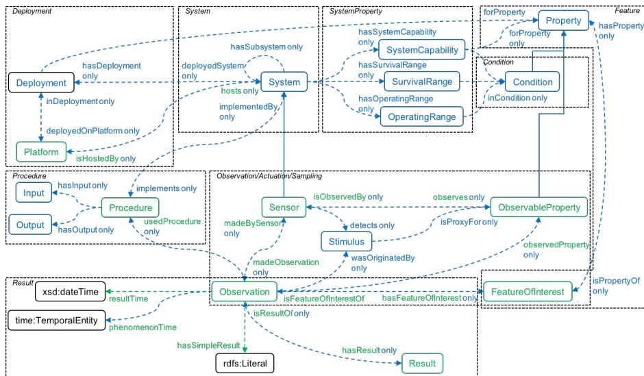
図 2.30 SSN OntStructure Observation[23]
