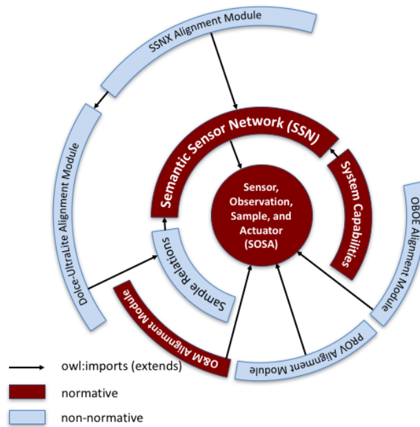
図 2.27 SOSA と SSN モデルのモジュール [23]
