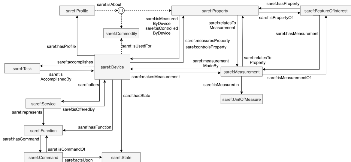
図 2.10 SAREF オントロジー [16]
