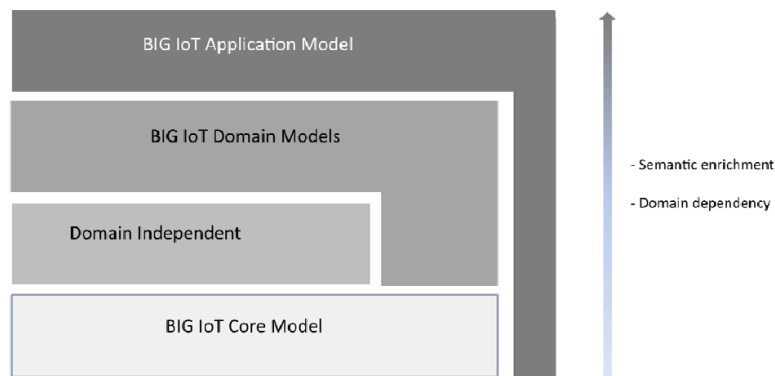
図 2.24 BIG IoT モデルのレイヤ [20]
