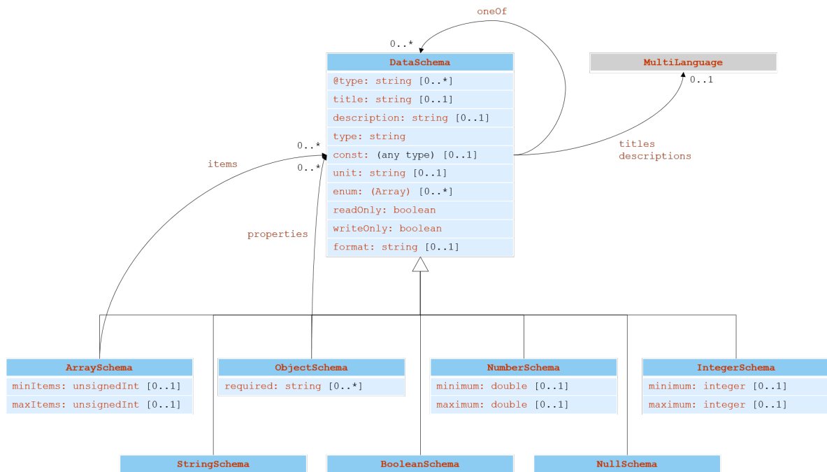
図 2.21 Data schema vocabulary[18]
