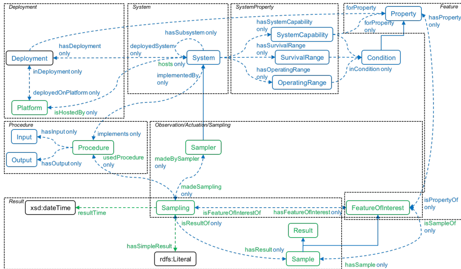
図 2.31 SSN OntStructure Sampling[23]
