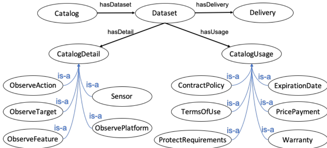
図 4.5 JEITA スマートホームデータカタログオントロジーのグラフ表現 (クラスレベルまで)
