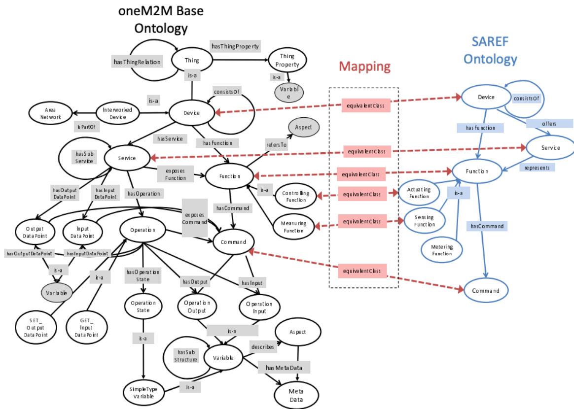
図 2.11 SAREF を oneM2M にマッピング [16]
