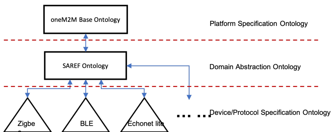
図 2.37 情報モデル角度のレイヤ
