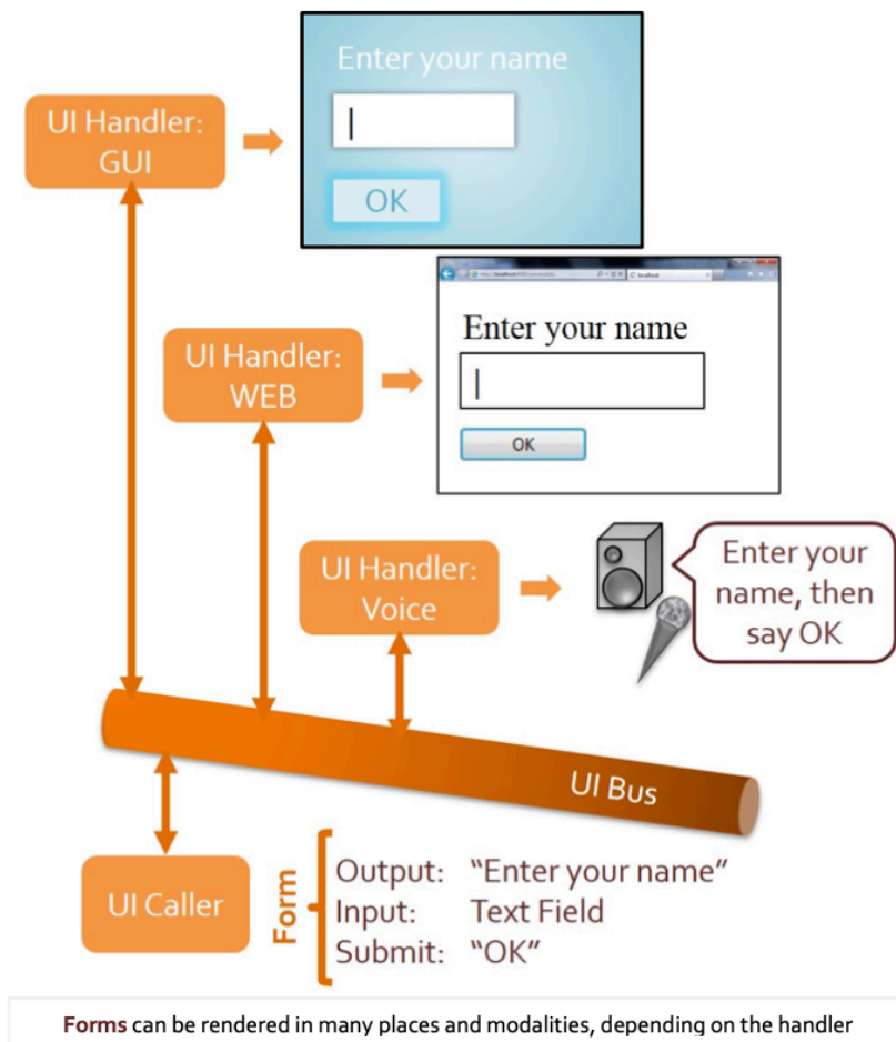
図 2.5 uAAL の UI バス [7]
