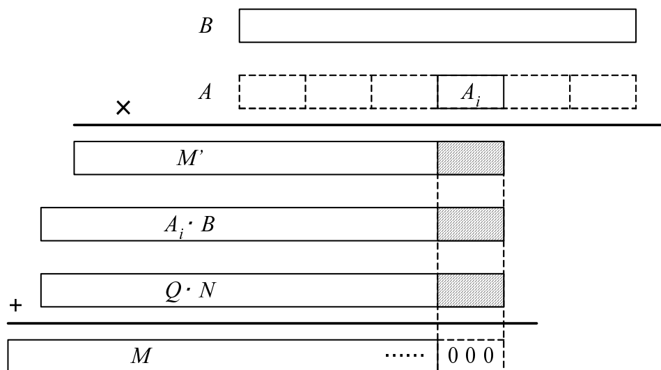
図 4.2: Step2 ~ Step4 の繰り返し
