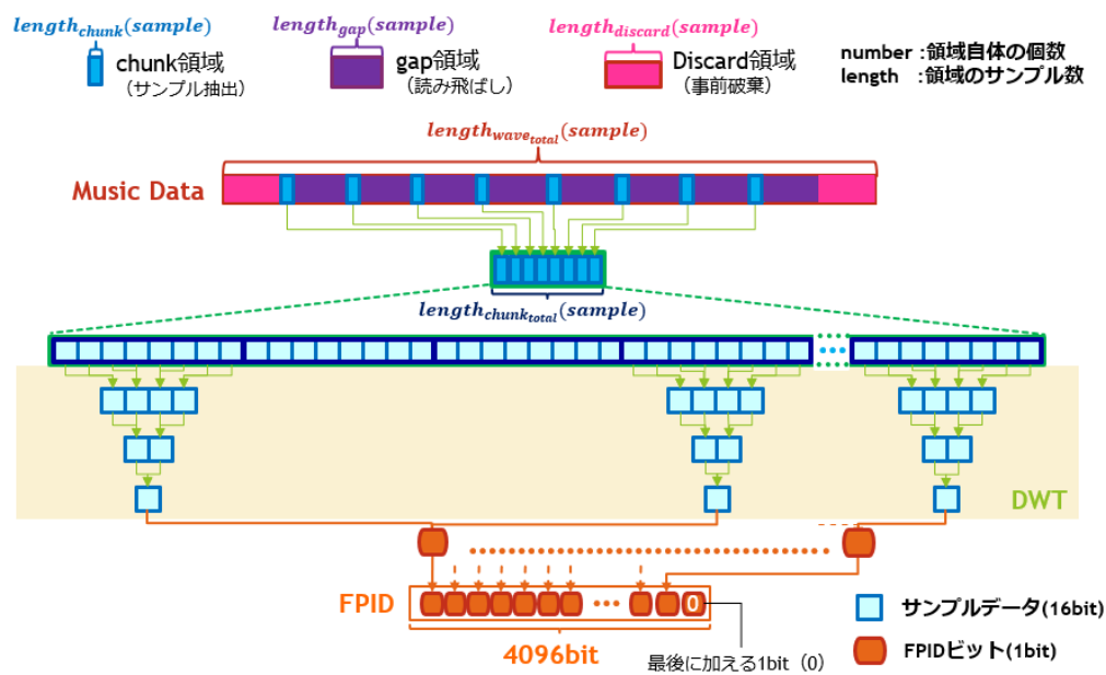
図 3.1: HiFP2.0 と HiFP2.1 の抽出領域比較図解
