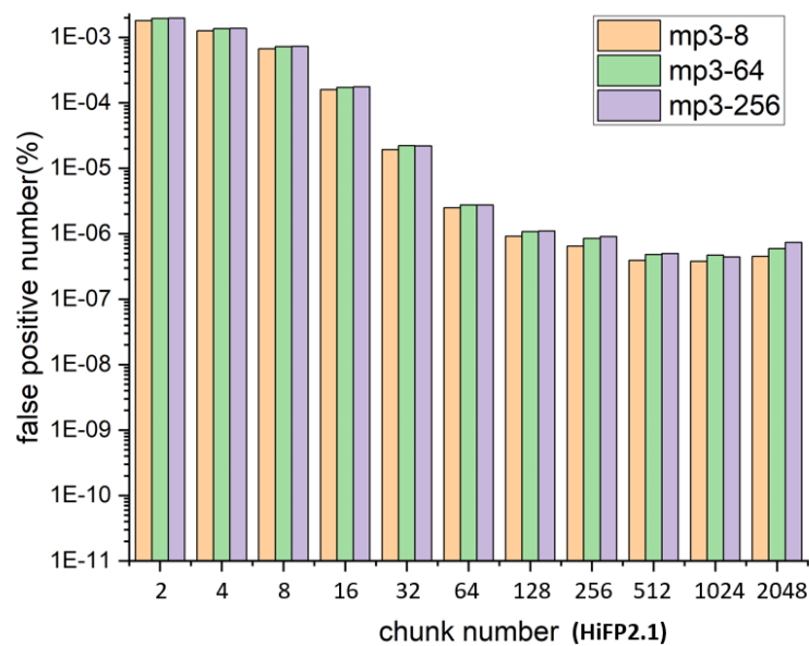
図 4.9: MP3 における偽陽性の識別失敗数のグラフ
