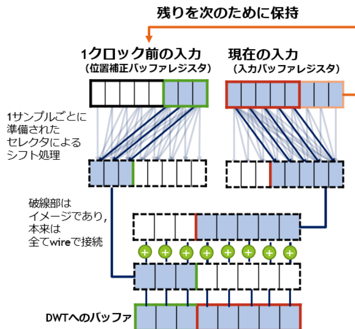
図 3.8: 抽出サンプル選択のイメージ図
