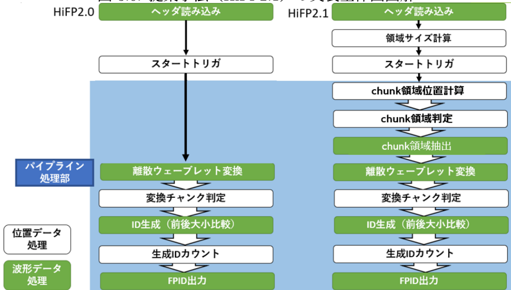
図 3.6: 提案手法 (HiFP2.1) の実装全体図図解
