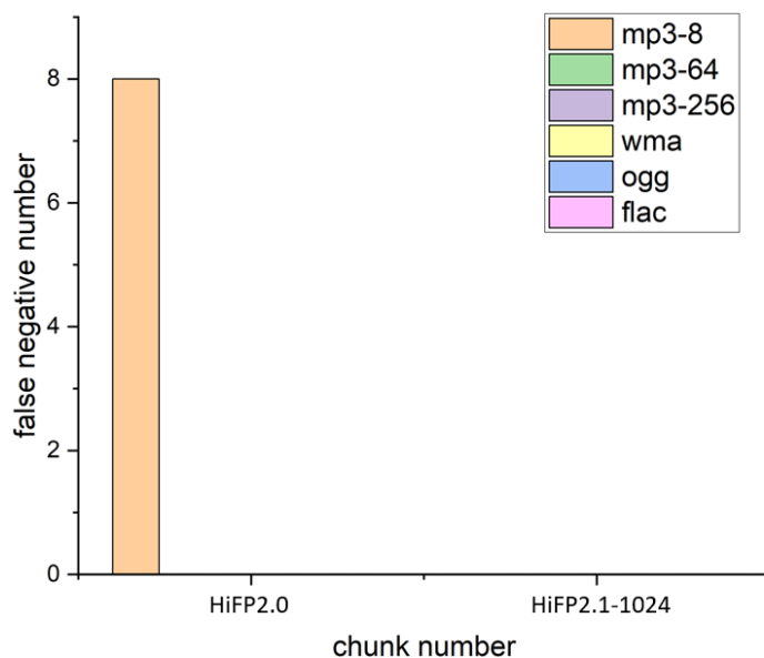
図 4.14: HiFP2.0 アルゴリズムの FPGA 上でサンプル抽出を行う FPGA 実装および提案手法の偽陰性の検索失敗数のグラフ
