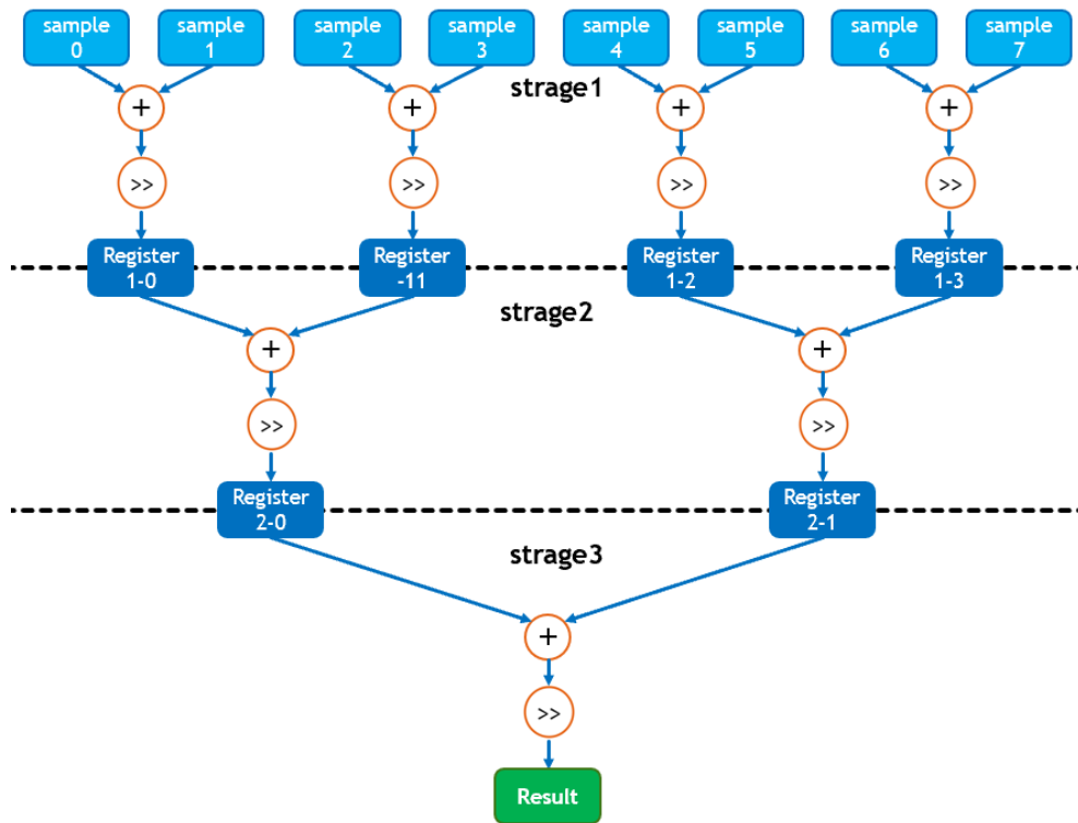
図 2.4: 離散ウェーブレット変換の回路図解
