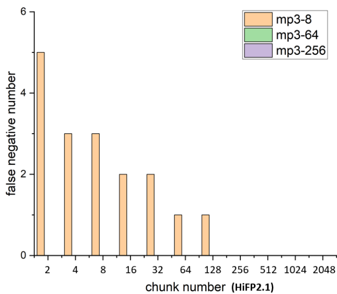
図 4.10: MP3 における偽陰性の識別失敗数のグラフ
