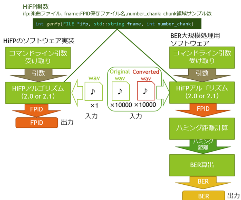
図 4.7: HiFP のソフトウェア実装と BER 大規模処理用ソフトウェアの違い
