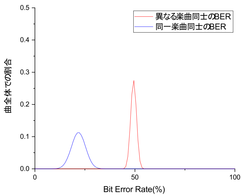
図 4.6: MP3 ABR8kbps における BER の正規分布
