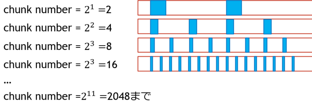
図 3.5: チャンク領域数のパターンの図解
