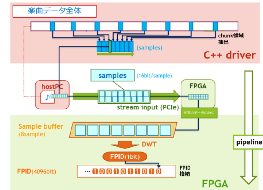
図 3.4: サンプル抽出タイミングの違いによる 2 つの実装全体図図解
