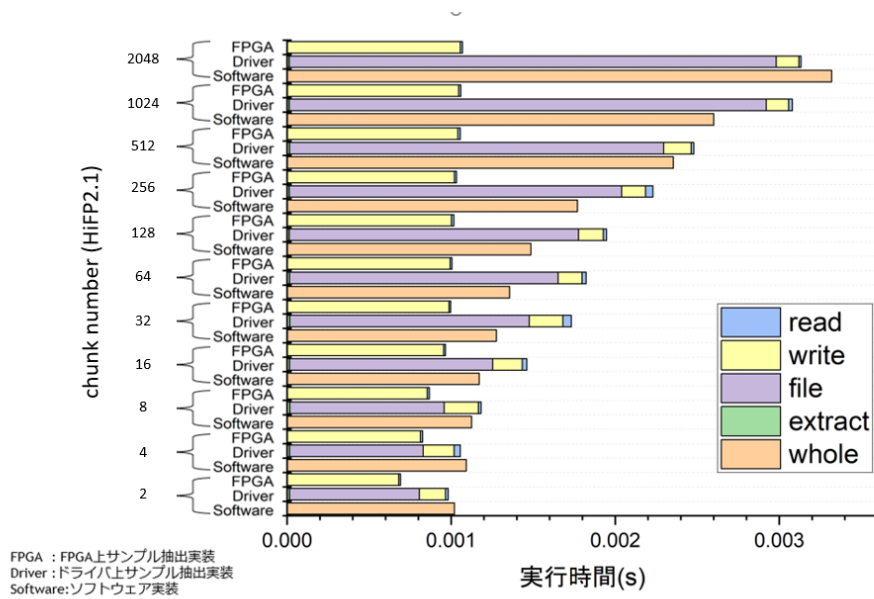
図 4.3: 各種実装形式での実行時間における実行時間のグラフ
