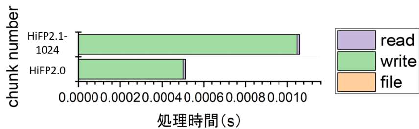
図 4.13: HiFP2.0 アルゴリズムの FPGA 上でサンプル抽出を行う FPGA 実装および提案手法の実行時間
