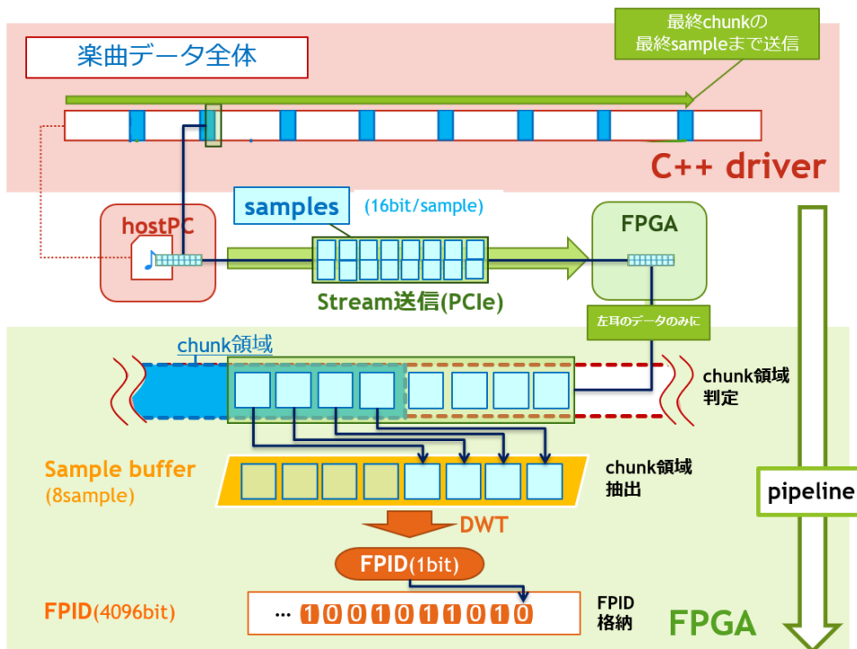
図 3.6: 提案手法 (HiFP2.1) の実装全体図図解
