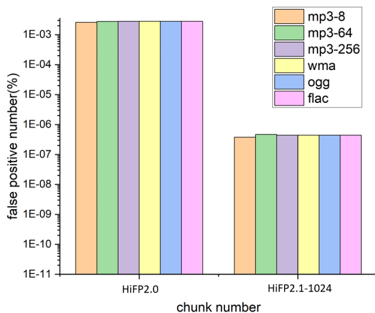
図 4.15: HiFP2.0 アルゴリズムの FPGA 上でサンプル抽出を行う FPGA 実装および提案手法の偽陽性の検索失敗数のグラフ
