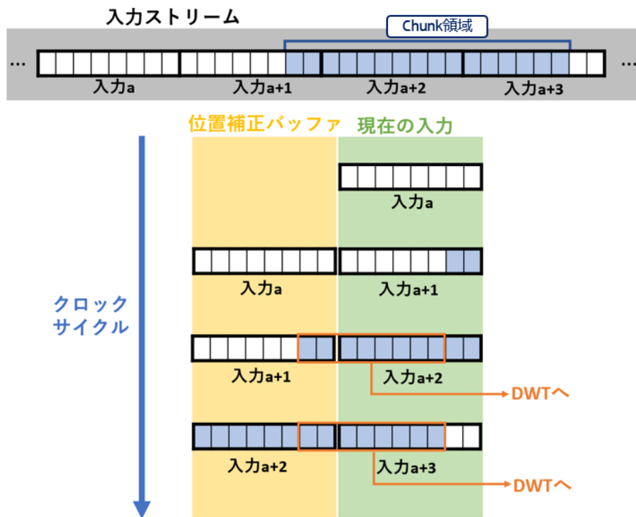
図 3.8: 抽出サンプル選択のイメージ図
