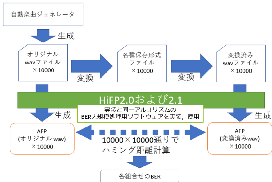
図 4.4: 実験 2 についての図解-BER 算出について
