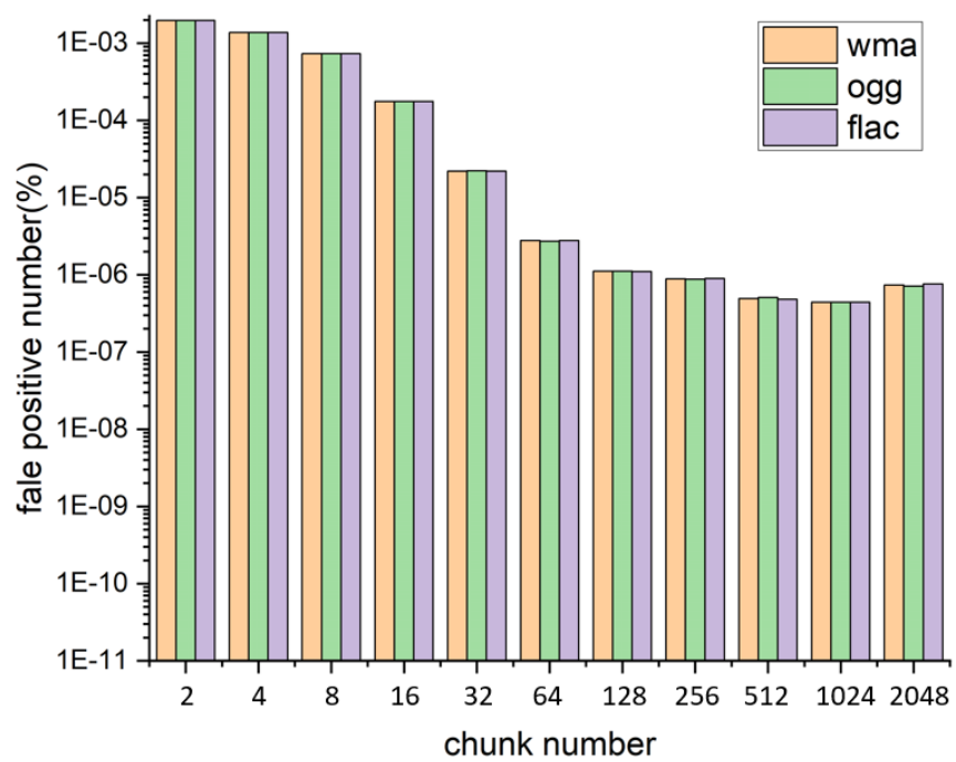
図 4.8: 各変換形式における偽陽性の識別失敗数のグラフ
