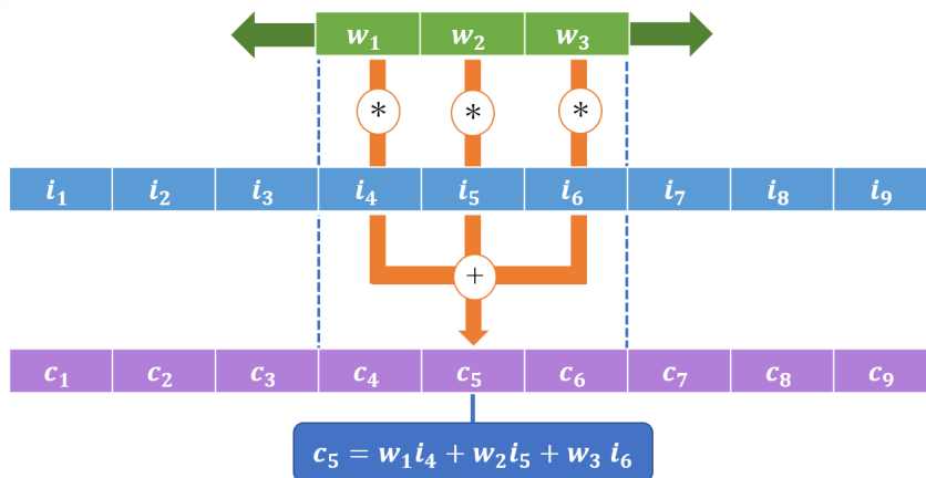
図 4.1: 1D Convolution の図解
