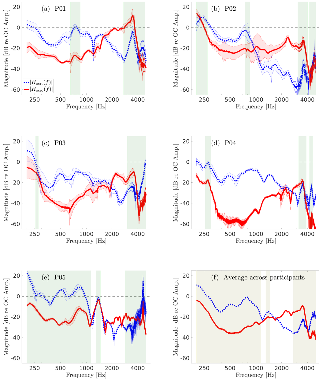
図 4.15: 口腔内音圧から側頭部振動までの伝達関数 ( |H_{ocrt}(f)| ) および口腔内音圧から外耳道内音圧までの伝達関数 ( |H_{occc}(f)| ) : (a) 参加者 P01, (b) 参加者 P02, (c) 参加者 P03, (d) 参加者 P04, (e) 参加者 P05, (f) 参加者 5 名の平均。点線は口腔内音圧から側頭部振動までの、実線は口腔内音圧から外耳道内音圧までの伝達関数の平均を表す。(a)–(e) における点線・実線の周囲の塗りつぶしは標準偏差を表す。薄く塗りつぶされた領域は、図 4.14(a)~4.14(f) における塗りつぶし領域と同様。
