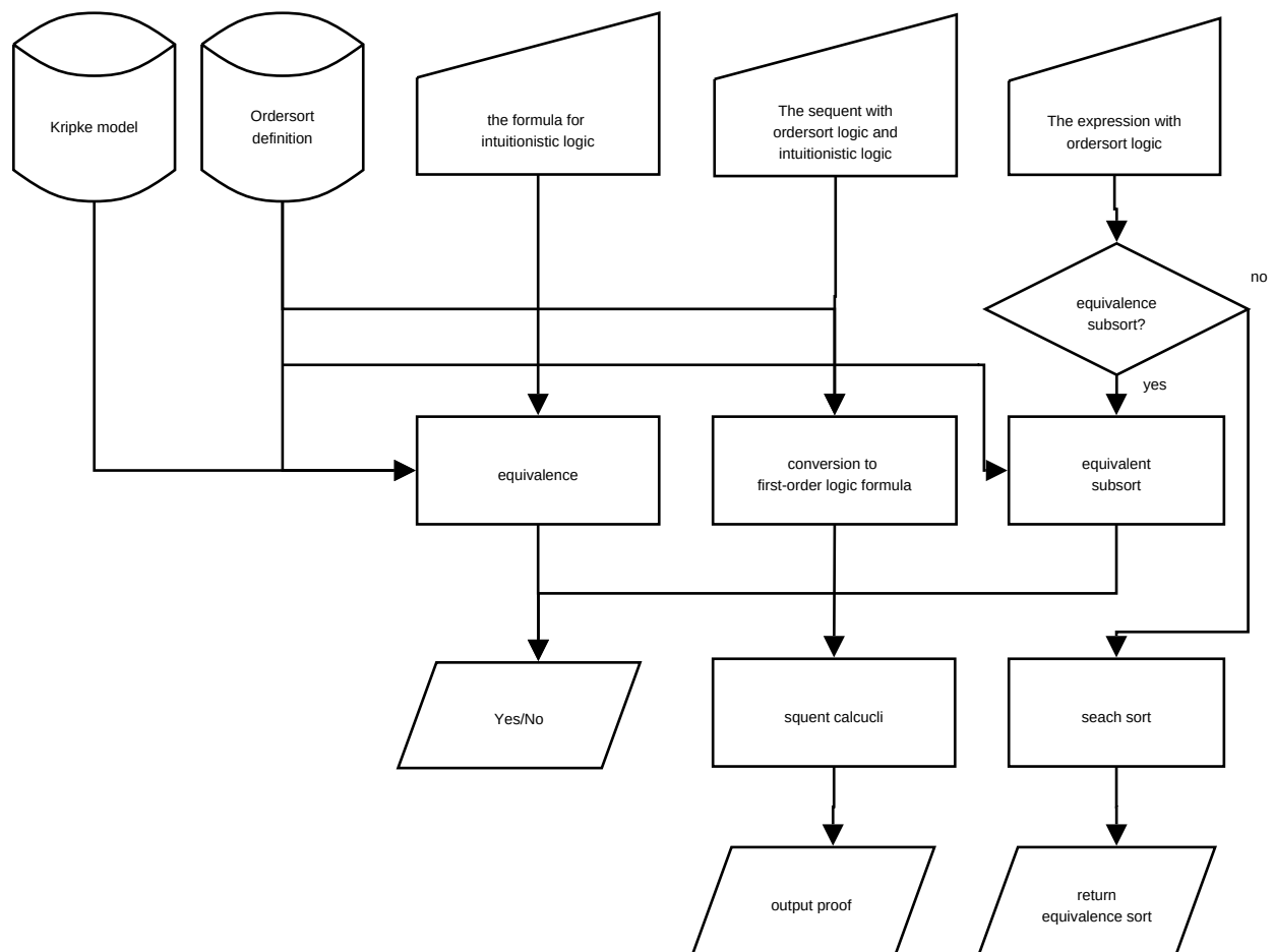
図 6.1 システム概要
