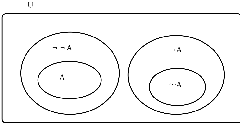
図 4.1 直観主義論理における対象領域
