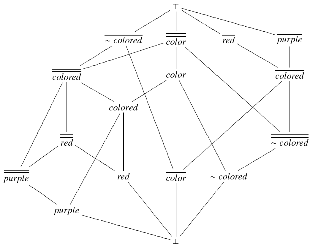
図 4.7 ソート階層の拡張（弱い否定ソートと強い否定ソート）
