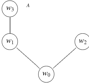
図 2.2 クリプキ・モデルの例：二重否定
