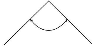
図 3.7 排他的関係・全域的關係
