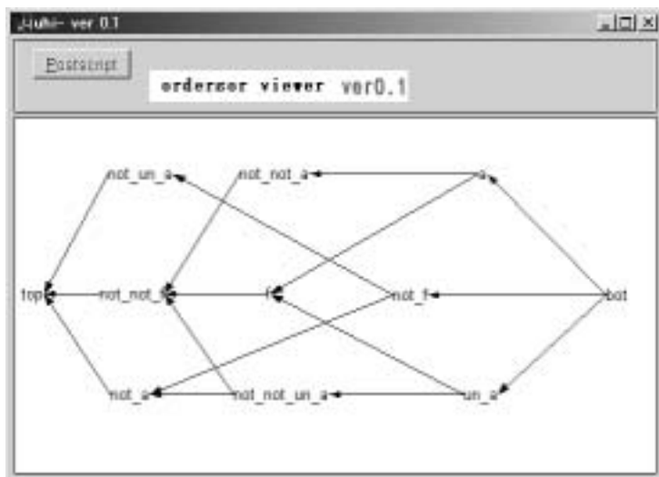
図 7.1 ソート階層の表示例
