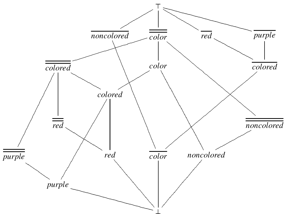
図 4.4 ソート階層の拡張（二重の弱い否定ソート例 1）
