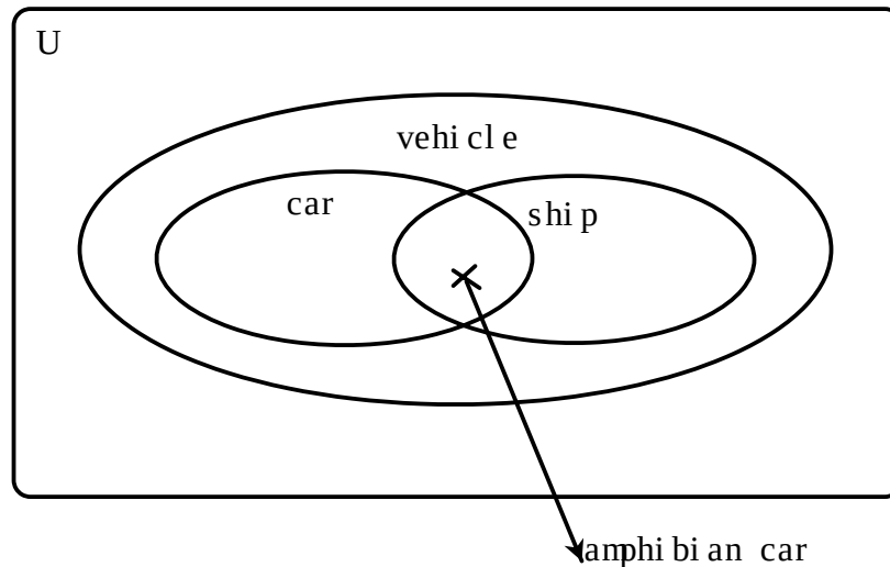
図 3.2 ソートのドメインの関係
