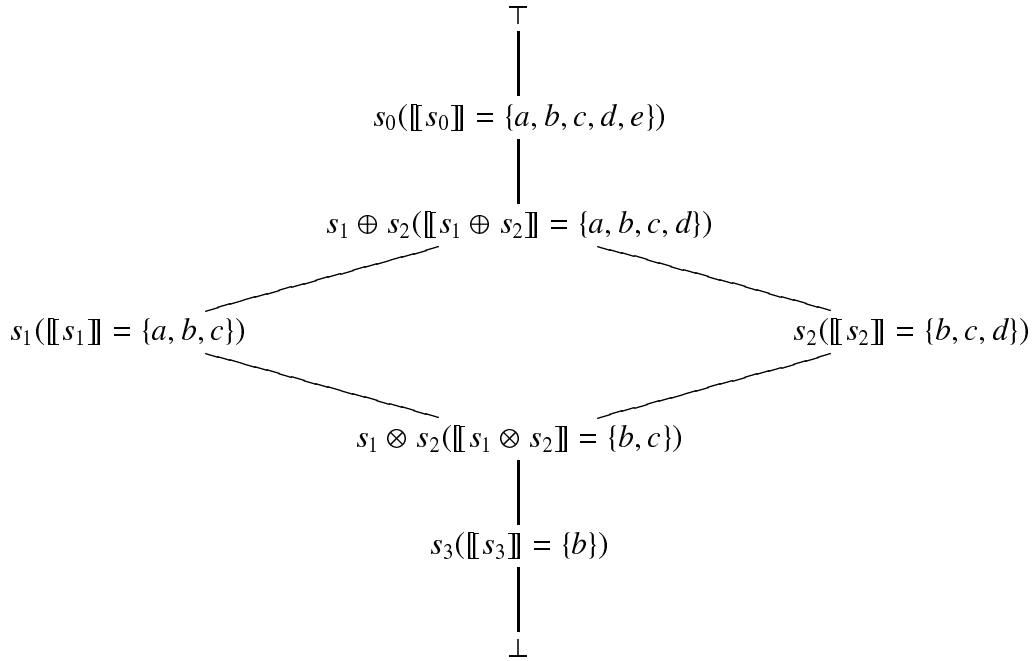
図 3.4 意味論的構造ソートを加えたソート階層の例
