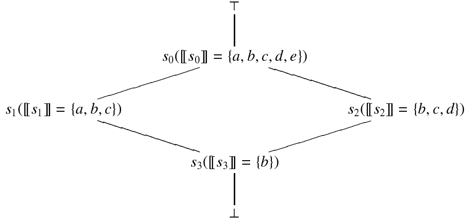
図 3.3 対象を考えたソート階層の例
