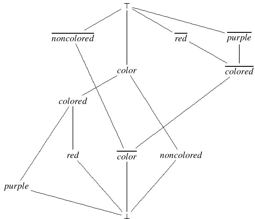
図 4.3 ソート階層の拡張（一重の弱い否定ソート）
