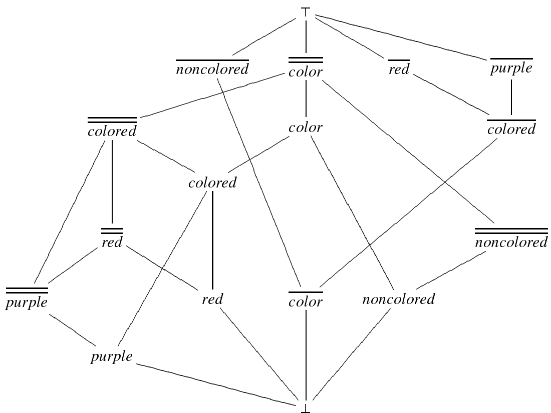
図 4.6 ソート階層の拡張（二重の弱い否定ソート例 2）
