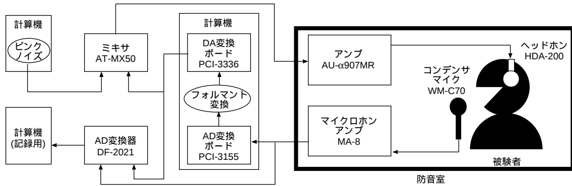
図 3.1: 実験装置
