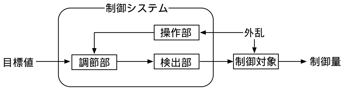
図 2.1: フィードフォワード制御 (文献 [8] より引用)
