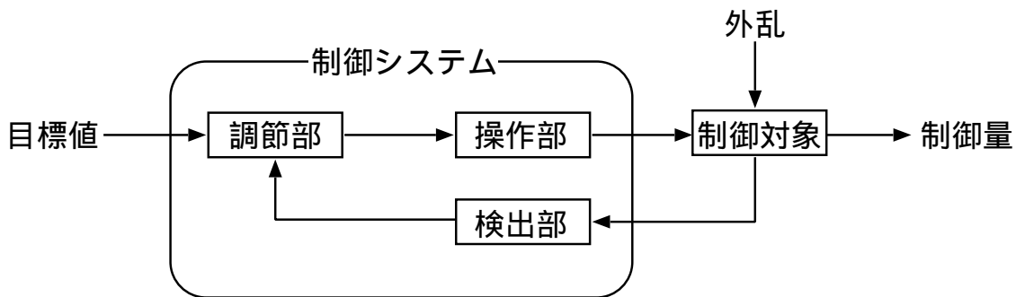
図 2.2: フィードバック制御 (文献 [8] より引用)
