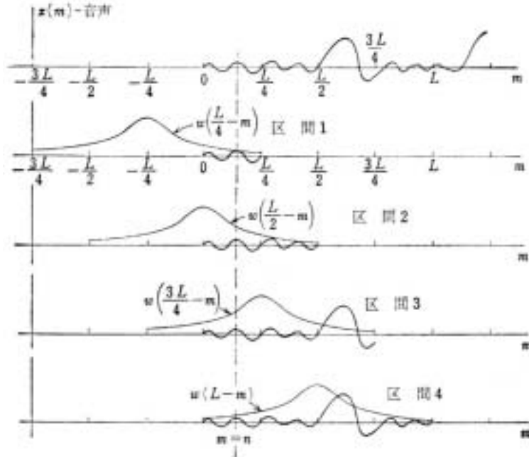
図 3.3: OLA 法 (文献 [6] より引用)
