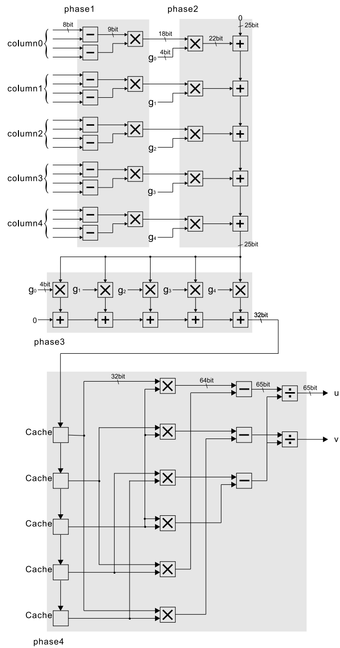
図 4.12: 全体の構成
