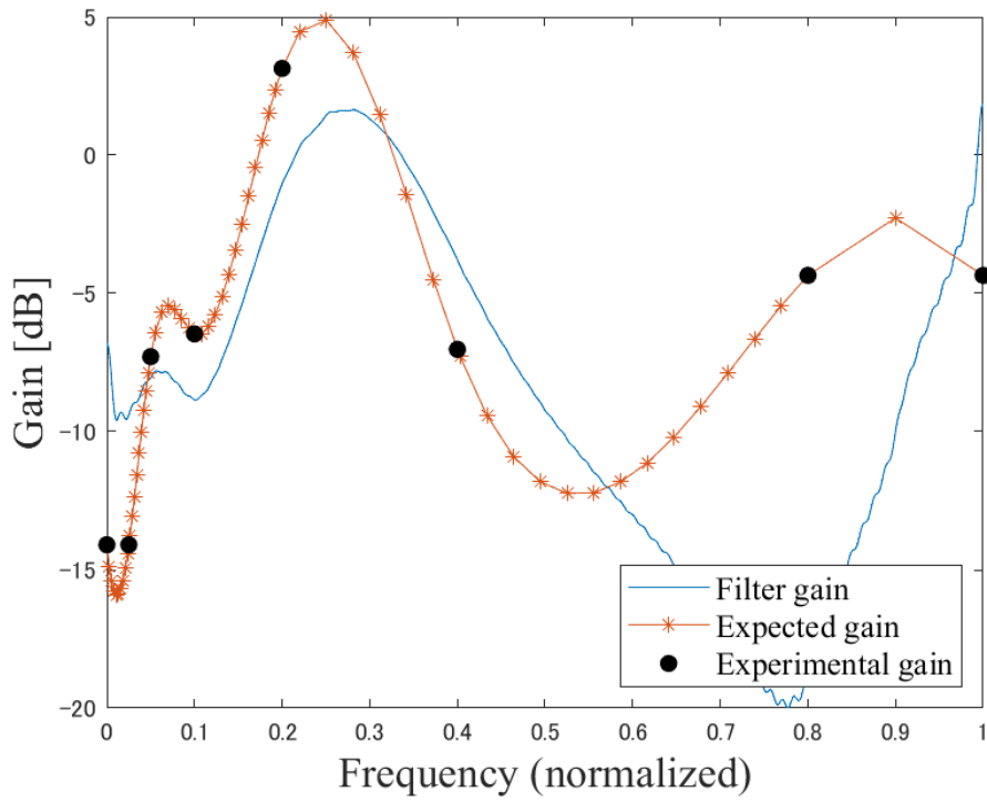
図 5.18: 実験参加者 H に適したフィルタの振幅応答
