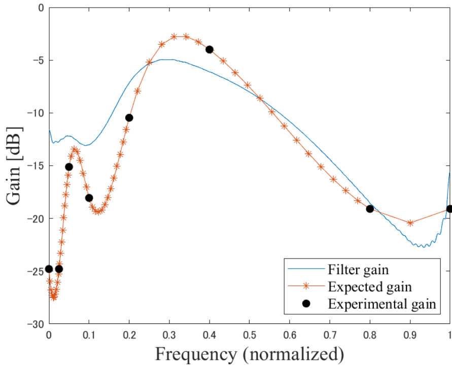
図 5.14: 実験参加者 F に適したフィルタの振幅応答
