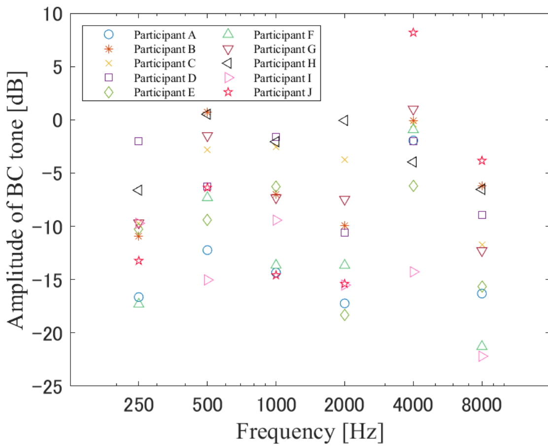
図 4.10: 純音を最も抑圧する骨導提示音の振幅
