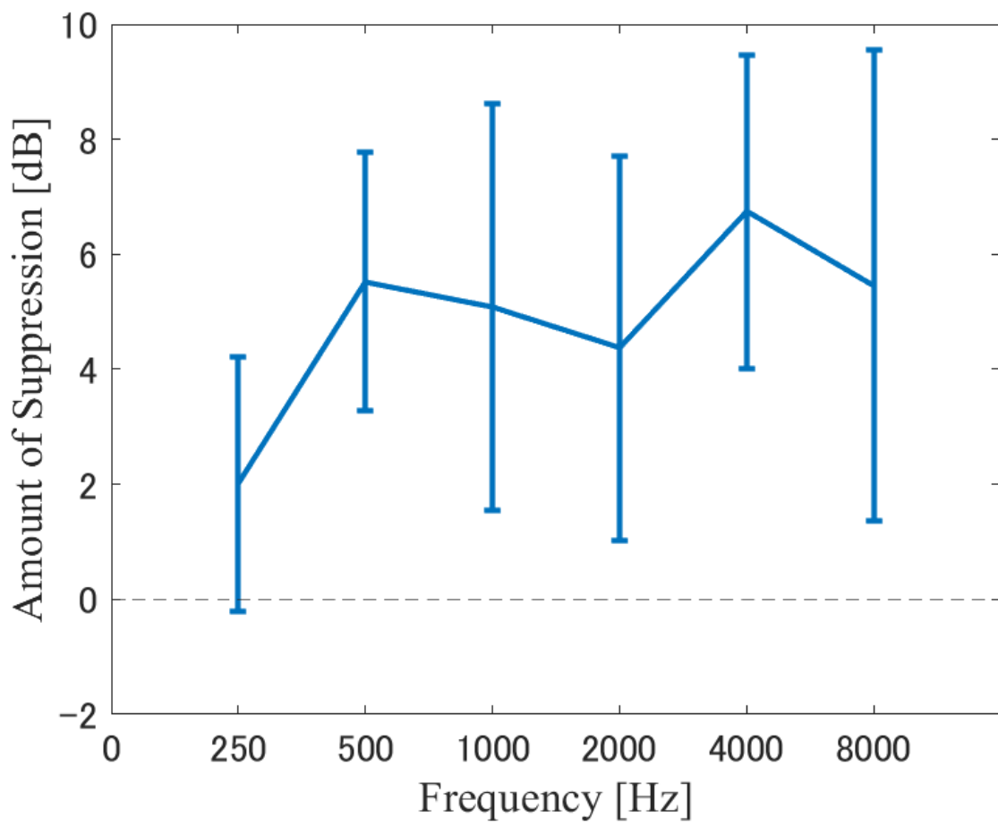
図 4.13: 純音の抑圧量の平均値と分散
