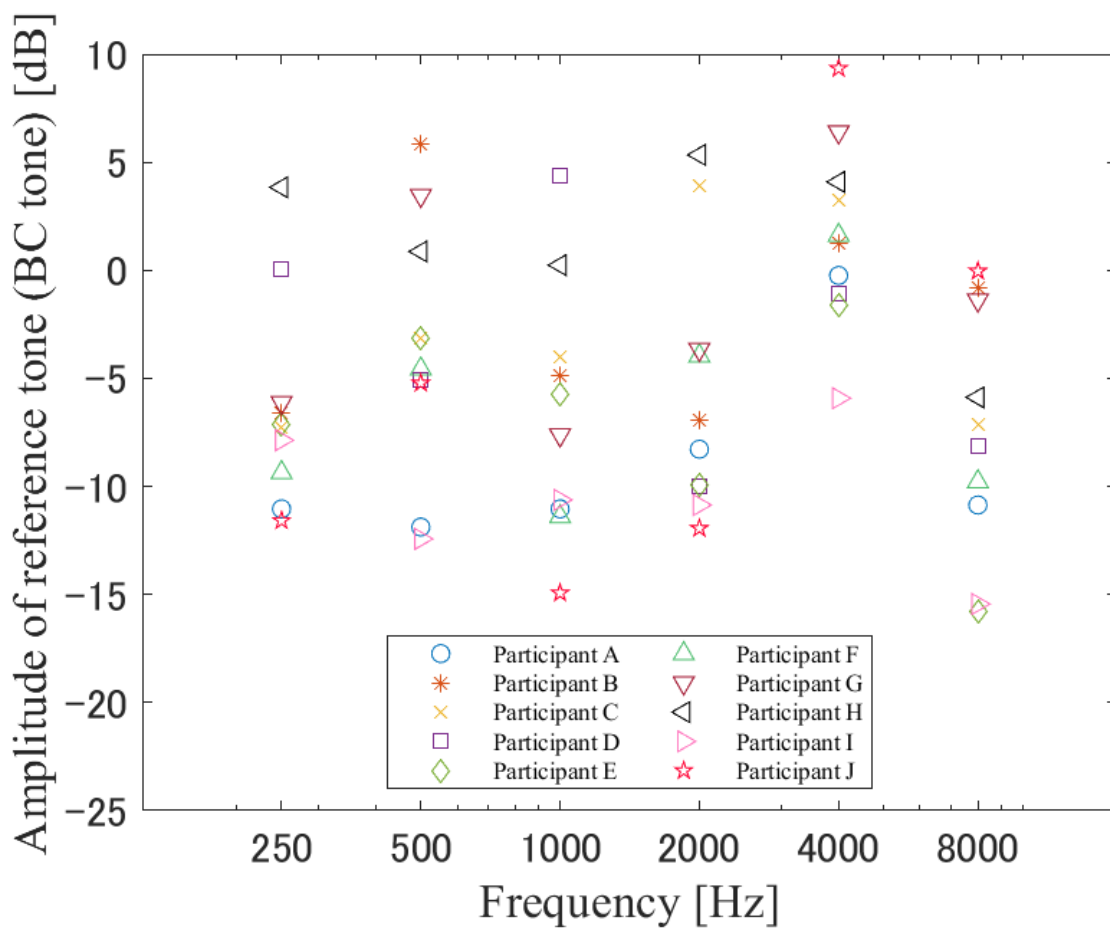
図 4.7: 実験 (1), 手順 I の結果
