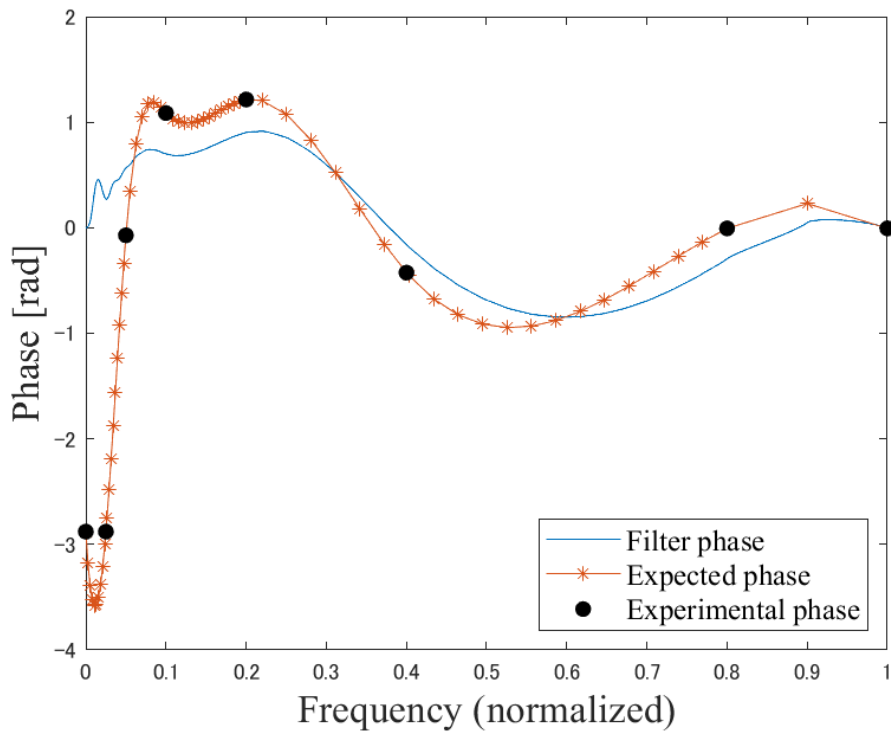
図 5.5: 実験参加者 A に適したフィルタの位相応答
