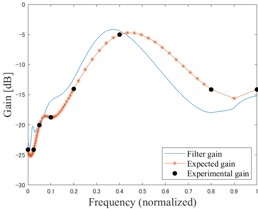
図 5.4: 実験参加者 A に適したフィルタの振幅応答
