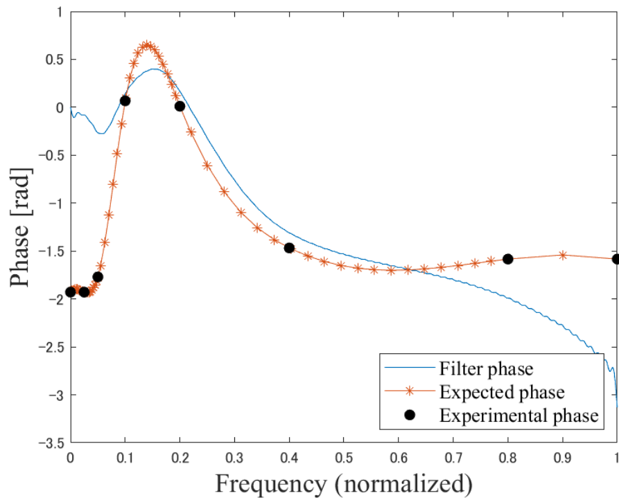
図 5.7: 実験参加者 B に適したフィルタの位相応答
