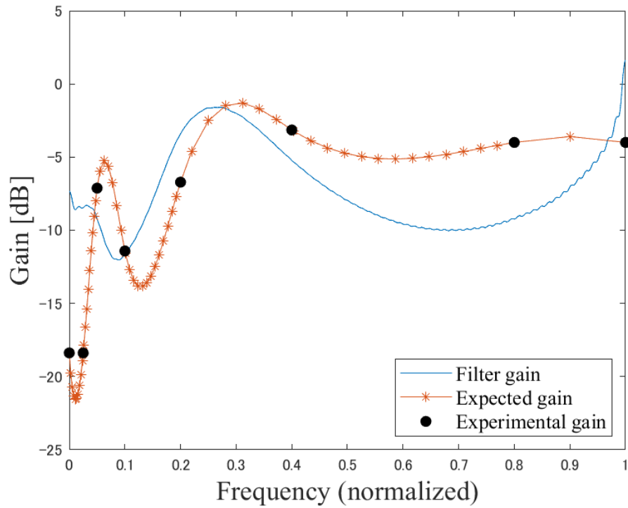
図 5.6: 実験参加者 B に適したフィルタの振幅応答
