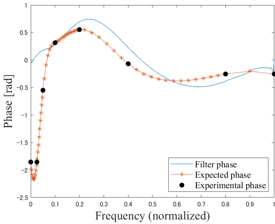
図 5.23: 実験参加者 J に適したフィルタの位相応答
