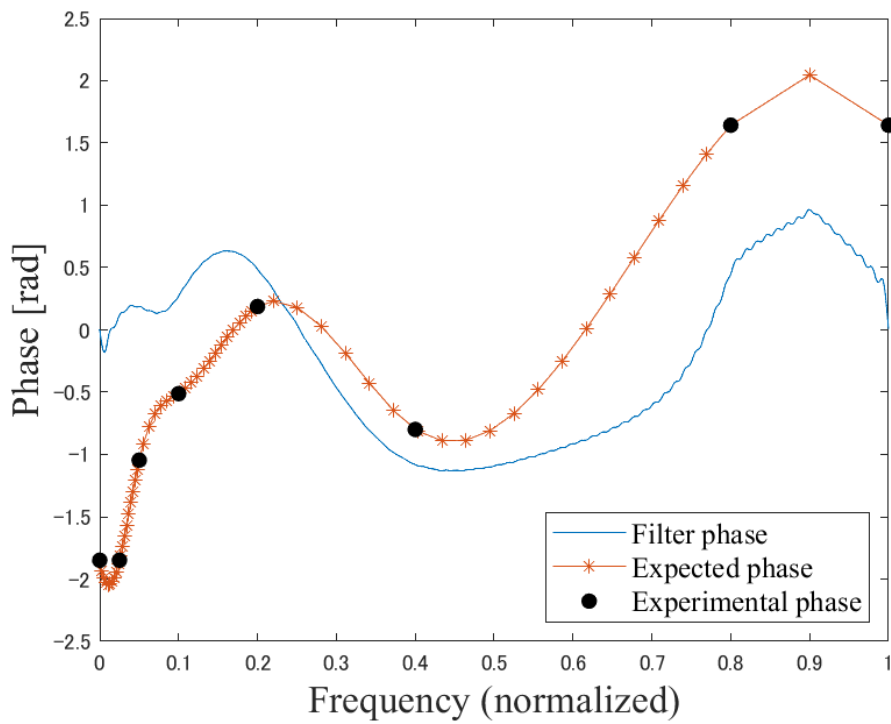
図 5.19: 実験参加者 H に適したフィルタの位相応答
