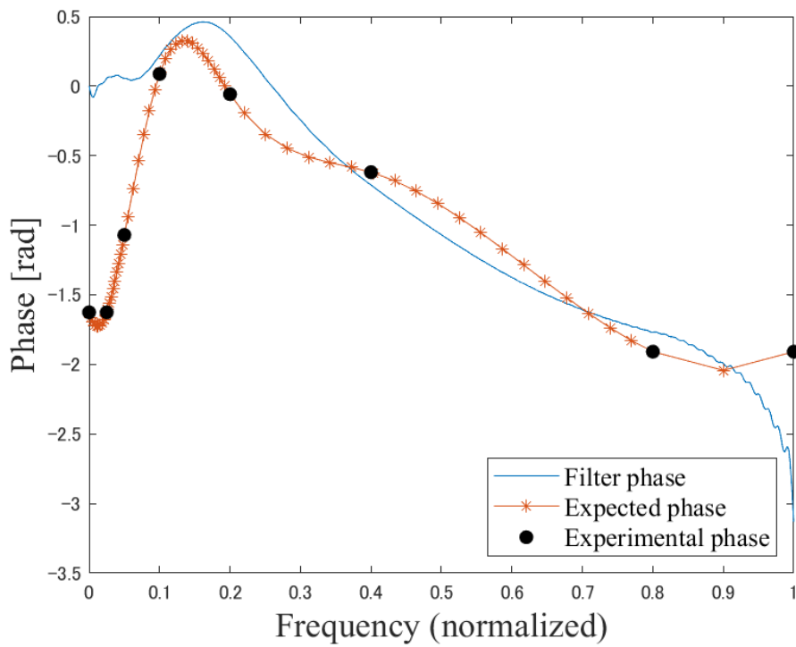
図 5.15: 実験参加者 F に適したフィルタの位相応答
