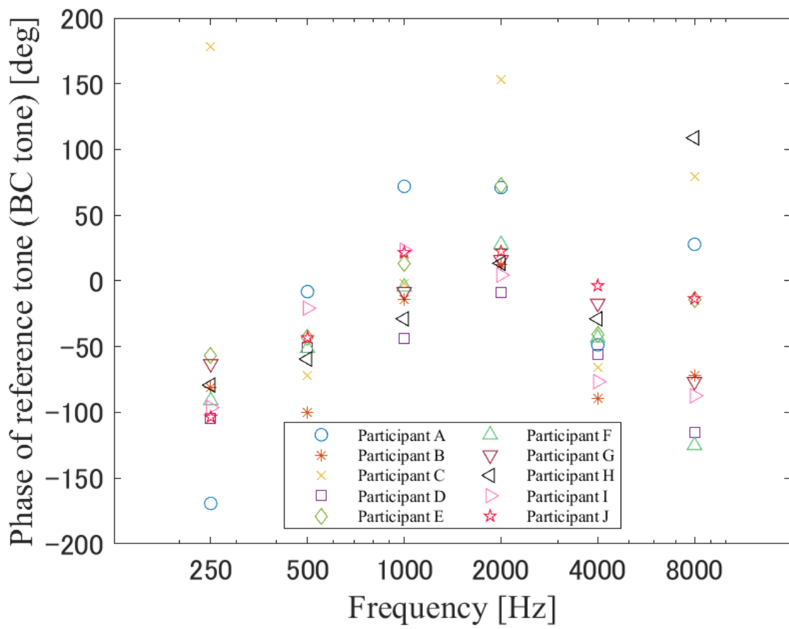
図 4.8: 実験(1), 手順 II の結果
