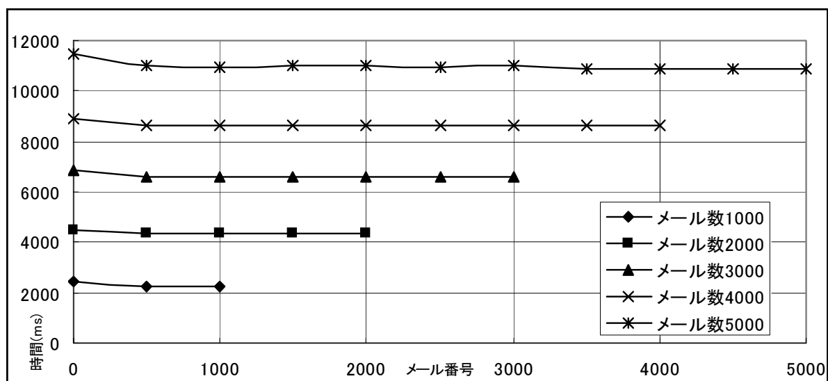
図 6.3: 方式4 の処理時間
