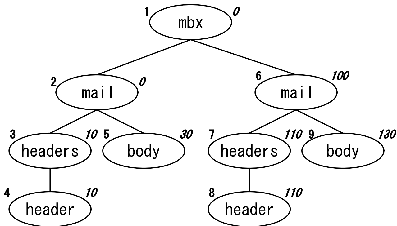
図 5.1: MBX データの木構造での表現
