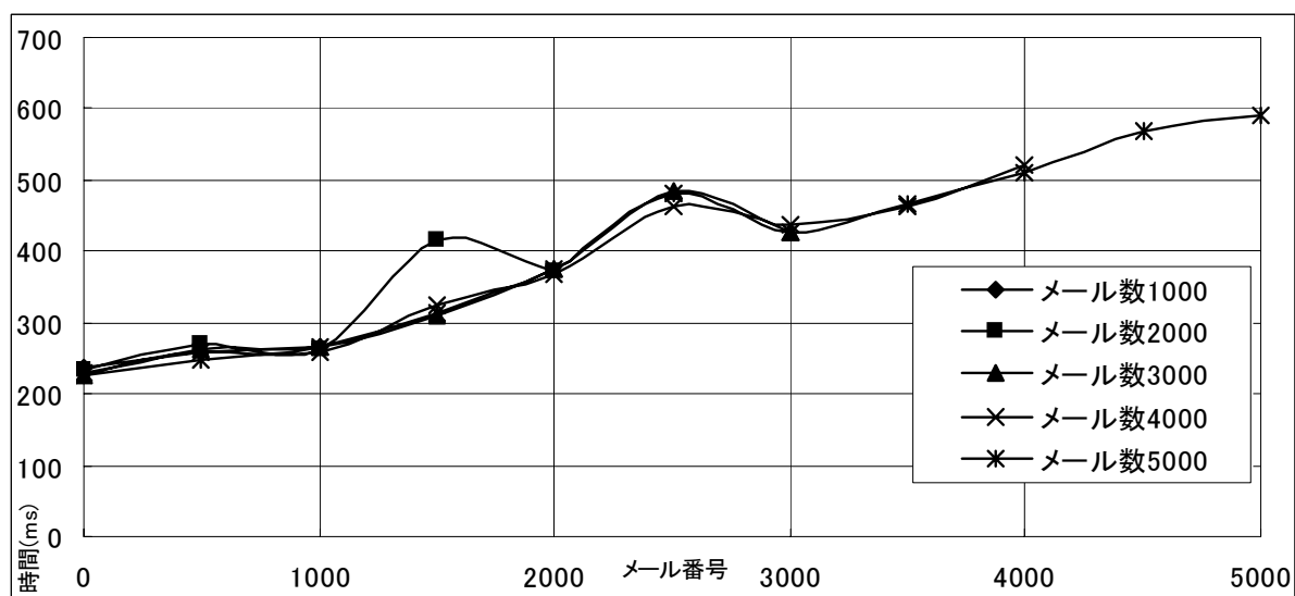
図 6.2: 方式3 の処理時間
