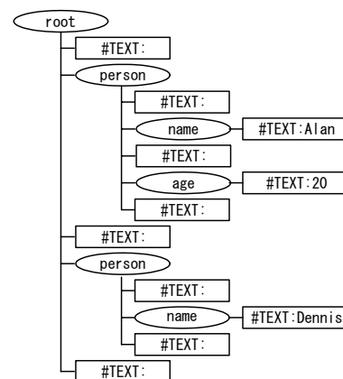
図 2.2: XML の木構造
