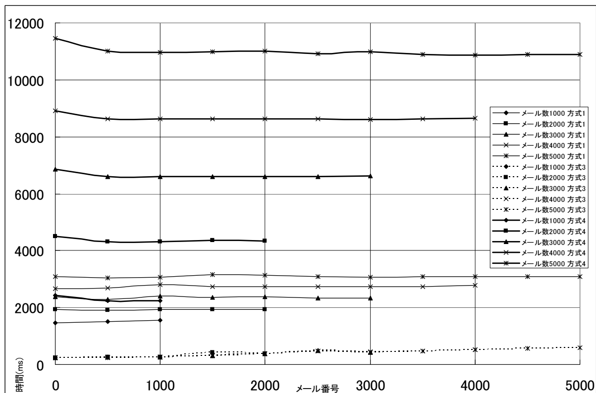
図 6.4: 方式 1,3,4 の処理時間
