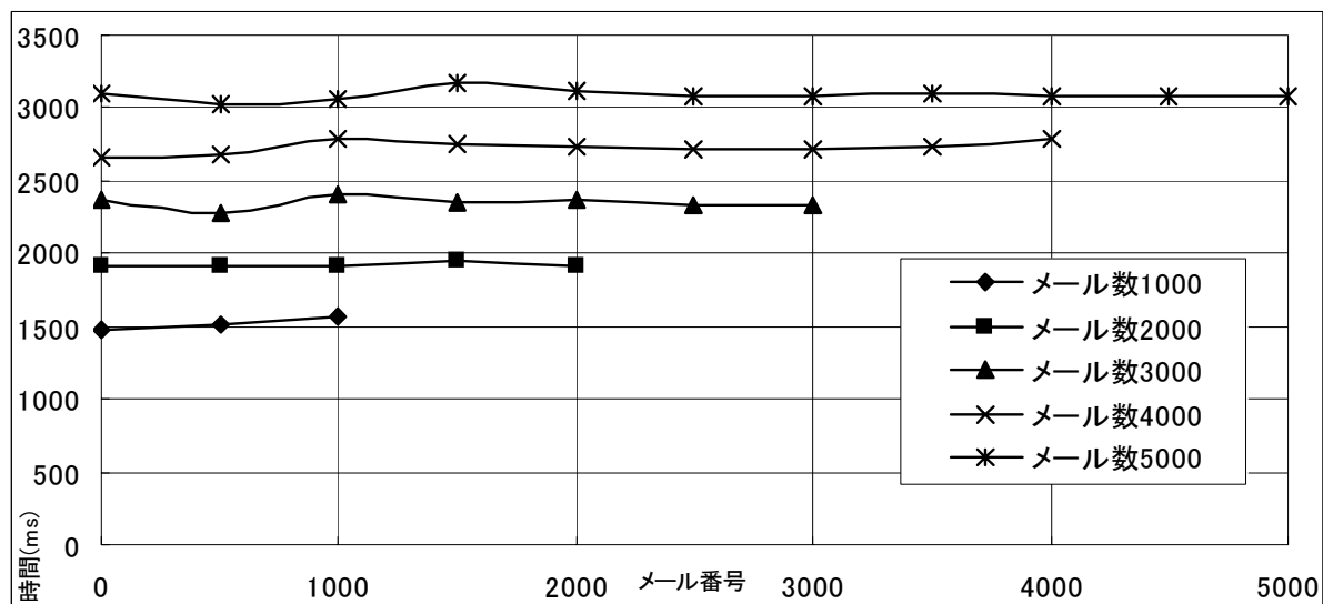
図 6.1: 方式 1 の処理時間
