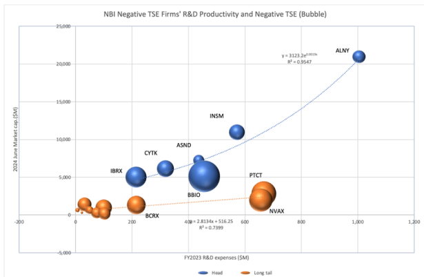
図 5. 債務超過のヘッド・ロングテール企業の R&D 生産性比較（バブル：債務超過）
