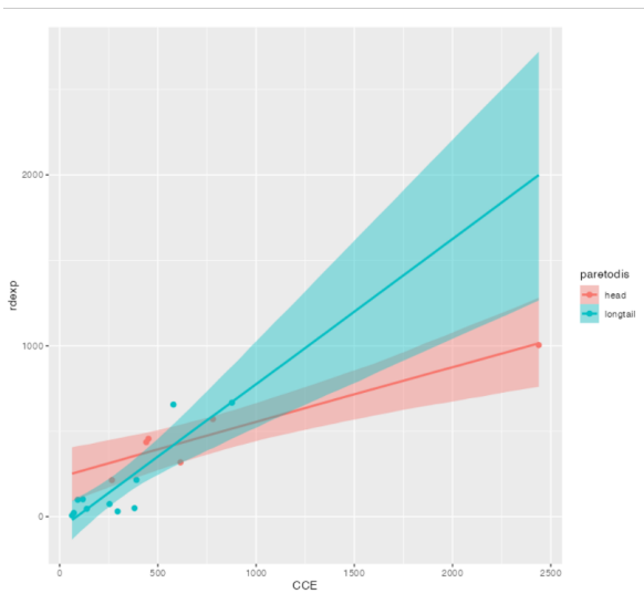
図 10. 債務超過企業のヘッド・ロングテール間の R&D 投資の CCE への依存度のベイズ McMC 交互作用解析
