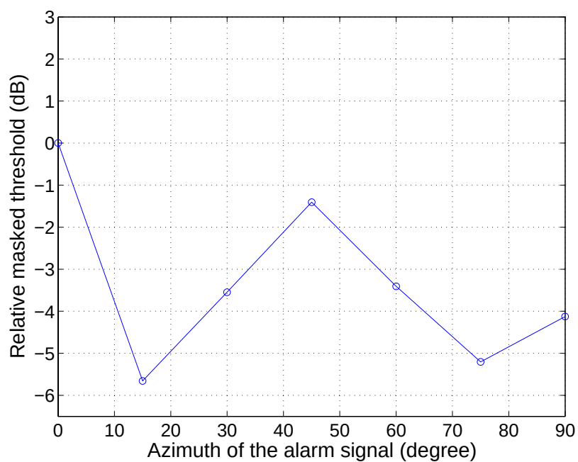
図 4.27: 成分周波数が 2.5 kHz の報知音の知覚特性: 被験者 H
