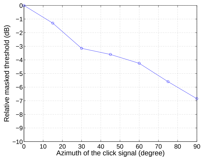
図 3.9: クリック音の知覚特性: 被験者 E
