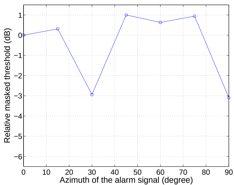
図 4.16: 成分周波数が 2.0 kHz の報知音の知覚特性: 被験者 F
