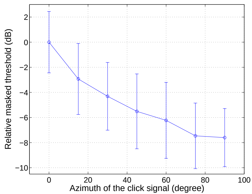
図 3.13: クリック音の知覚特性: 全被験者の平均
