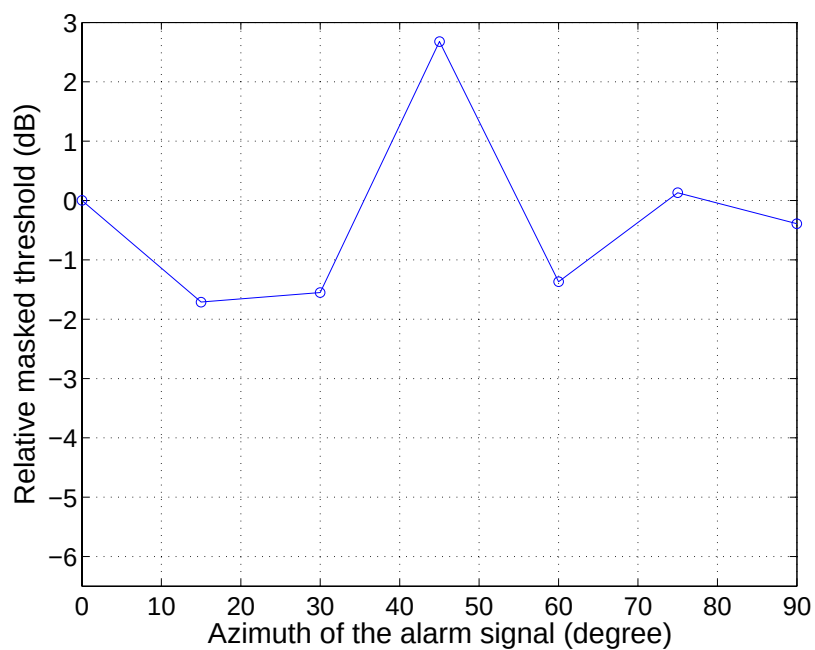
図 4.22: 成分周波数が 2.5 kHz の報知音の知覚特性: 被験者 C
