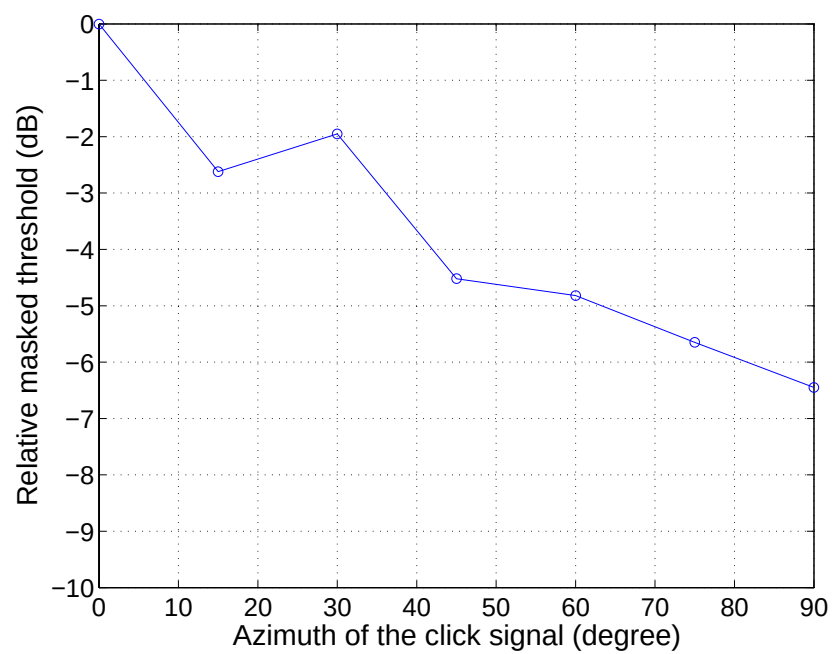
図 3.12: クリック音の知覚特性: 被験者 H
