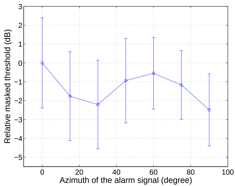
図 4.19: 成分周波数が 2.0 kHz の報知音の知覚特性: 全被験者の平均
