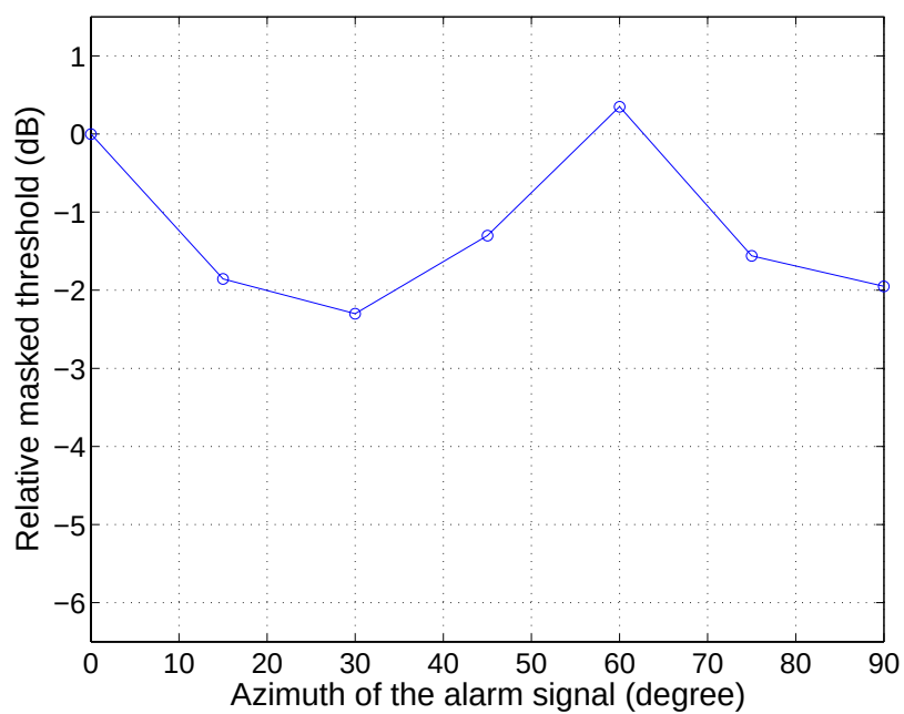
図 4.11: 成分周波数が 2.0 kHz の報知音の知覚特性: 被験者 A
