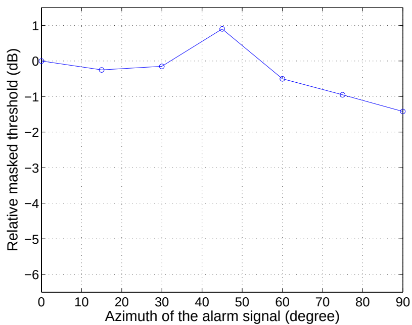
図 4.17: 成分周波数が 2.0 kHz の報知音の知覚特性: 被験者 G
