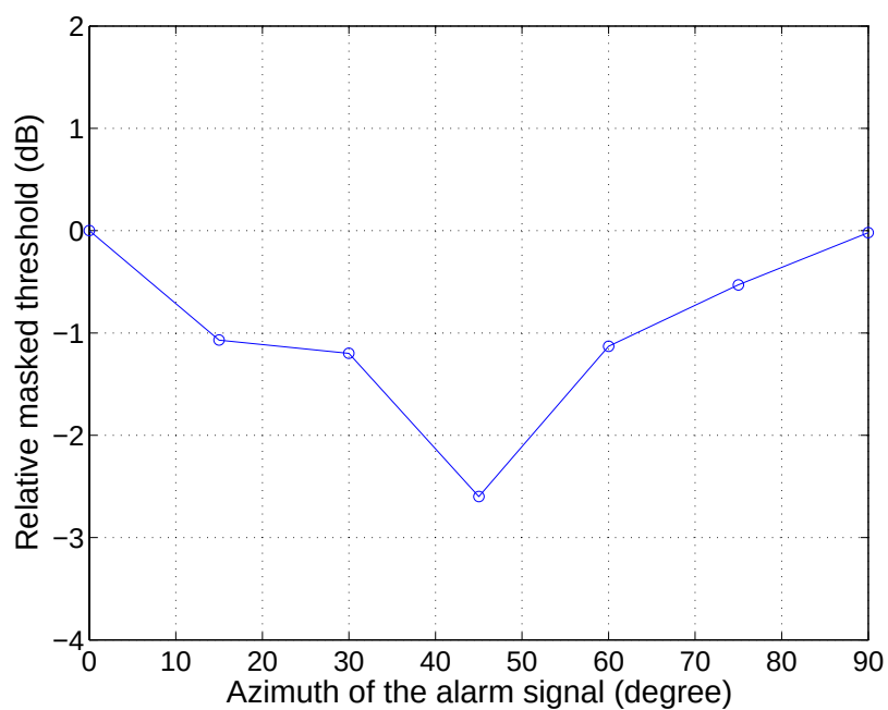
図 4.7: 成分周波数が 1.5 kHz の報知音の知覚特性: 被験者 F
