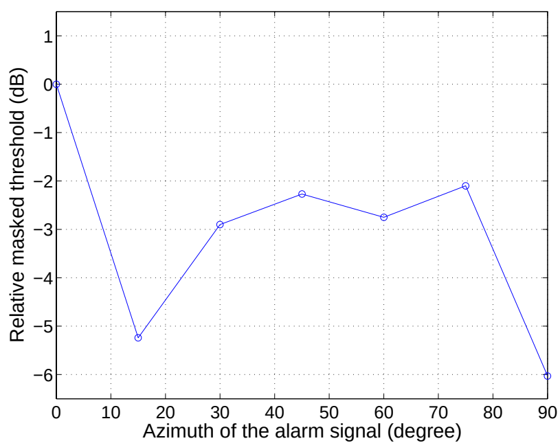
図 4.14: 成分周波数が 2.0 kHz の報知音の知覚特性: 被験者 D
