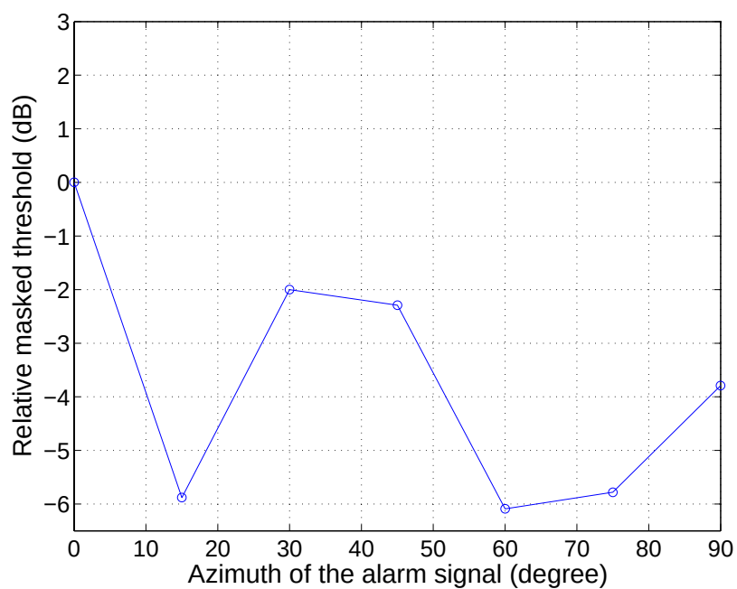
図 4.23: 成分周波数が 2.5 kHz の報知音の知覚特性: 被験者 D
