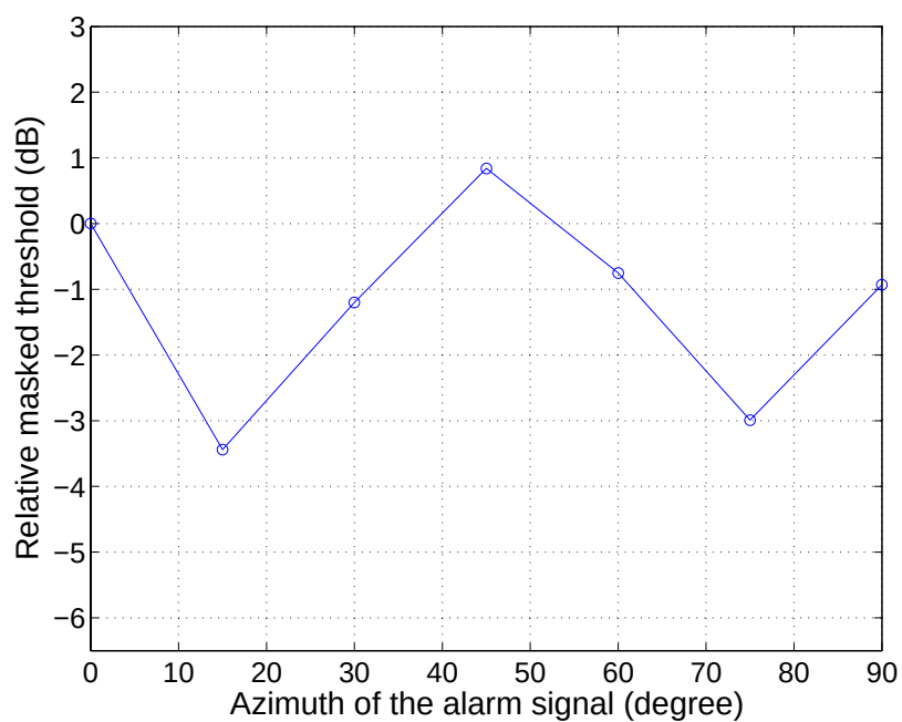
図 4.25: 成分周波数が 2.5 kHz の報知音の知覚特性: 被験者 F
