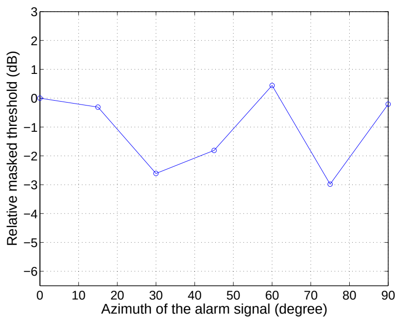
図 4.21: 成分周波数が 2.5 kHz の報知音の知覚特性: 被験者 B
