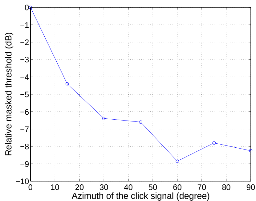
図 3.10: クリック音の知覚特性: 被験者 F
