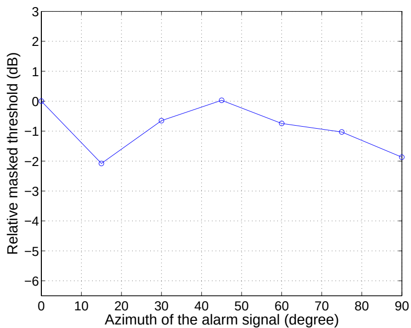
図 4.20: 成分周波数が 2.5 kHz の報知音の知覚特性: 被験者 A
