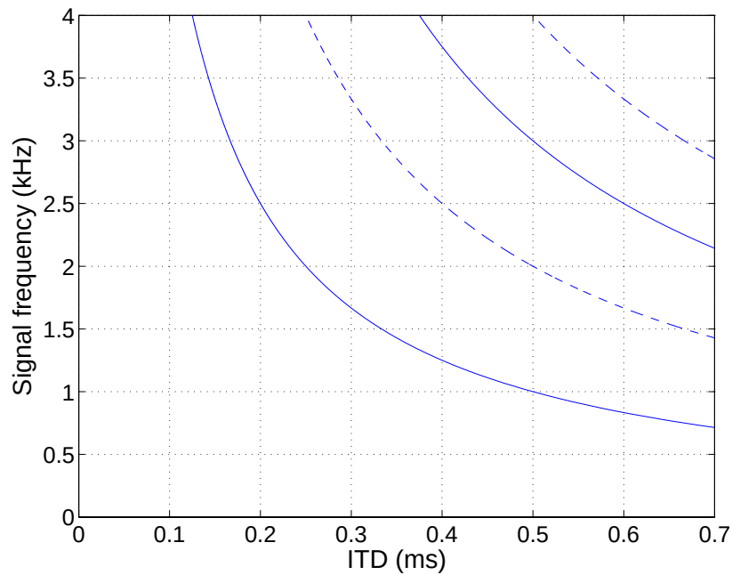
図 5.1: 両耳間時間差と報知音の成分周波数の関係。実線は逆位相条件、破線は同位相条件となる状態を示す。ITD が最大となる場合 (信号音が被験者の右側、または左側から呈示される場合) の時間差は約 0.68 ms である。
