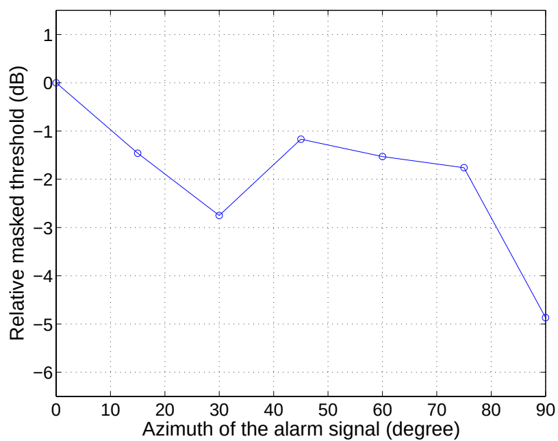
図 4.15: 成分周波数が 2.0 kHz の報知音の知覚特性: 被験者 E
