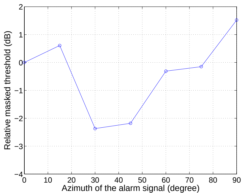
図 4.4: 成分周波数が 1.5 kHz の報知音の知覚特性: 被験者 C
