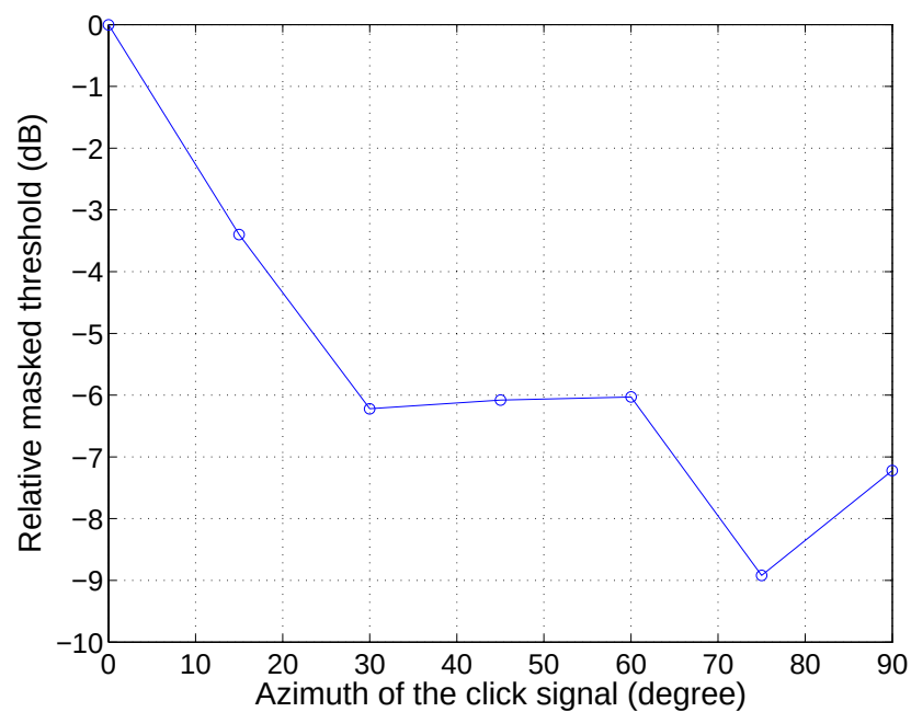
図 3.7: クリック音の知覚特性: 被験者 C
