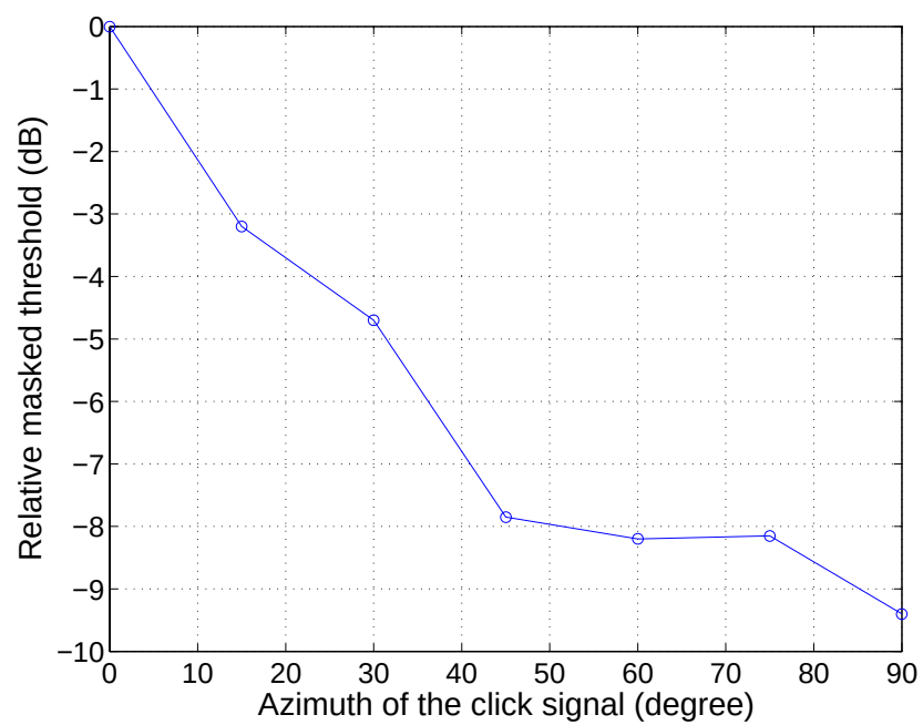
図 3.6: クリック音の知覚特性: 被験者 B
