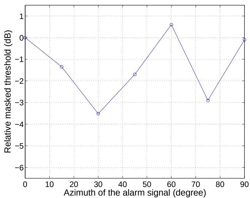
図 4.12: 成分周波数が 2.0 kHz の報知音の知覚特性: 被験者 B
