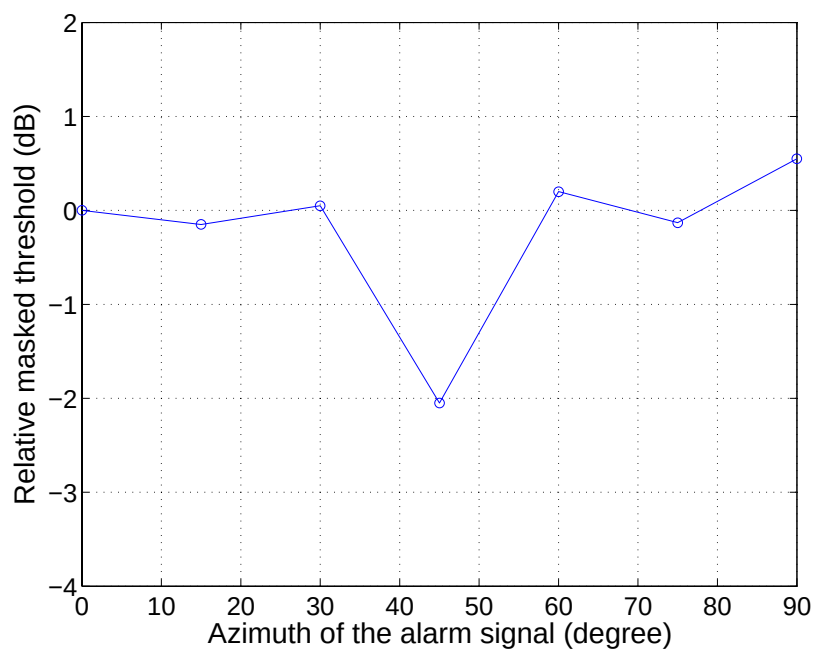
図 4.2: 成分周波数が 1.5 kHz の報知音の知覚特性: 被験者 A
