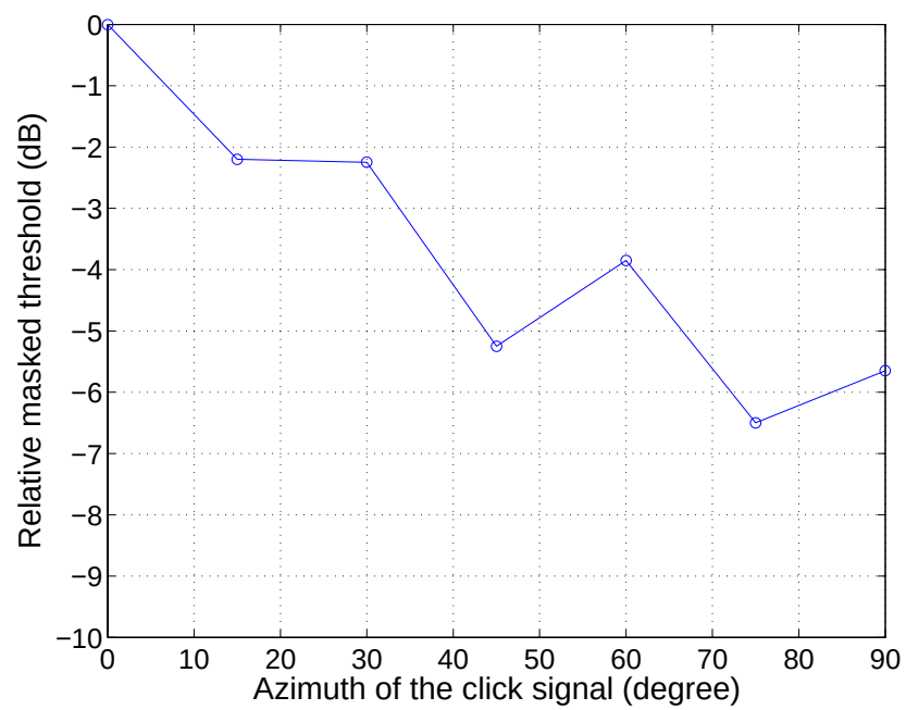
図 3.5: クリック音の知覚特性: 被験者 A
