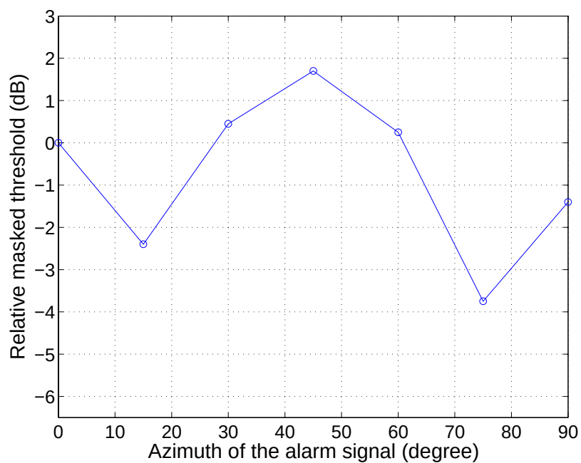
図 4.24: 成分周波数が 2.5 kHz の報知音の知覚特性: 被験者 E
