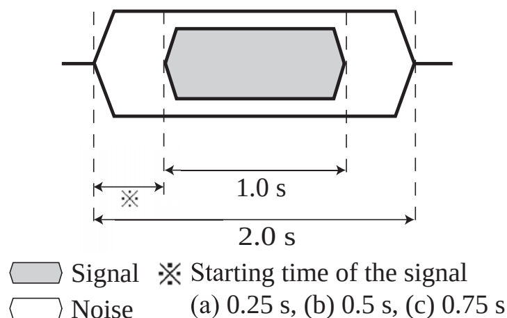
図 3.4: 白色雑音中の信号音呈示状況図。信号音の呈示開始時刻は (a)、(b)、(c) からランダムに決定する。
