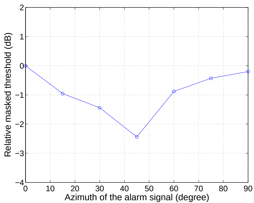
図 4.9: 成分周波数が 1.5 kHz の報知音の知覚特性: 被験者 H
