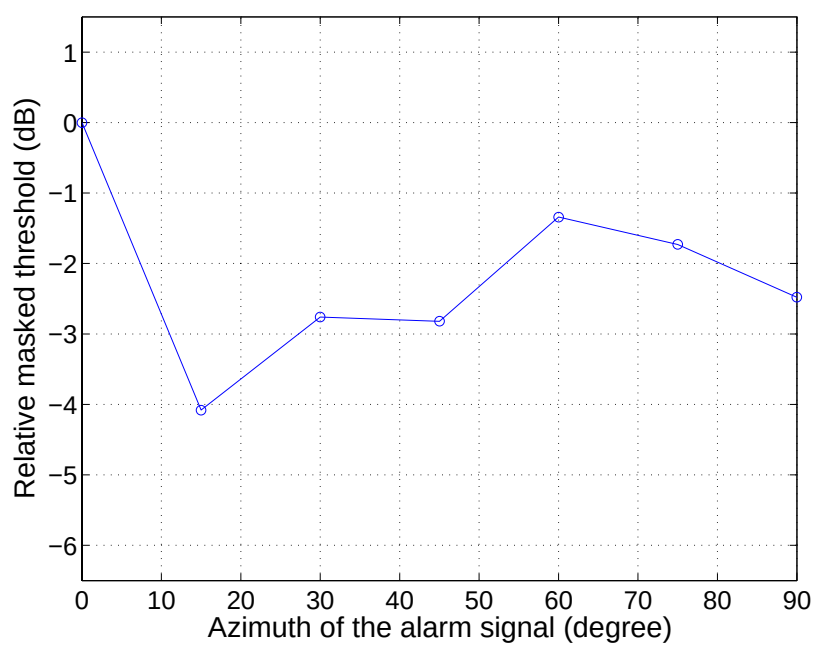
図 4.18: 成分周波数が 2.0 kHz の報知音の知覚特性: 被験者 H
