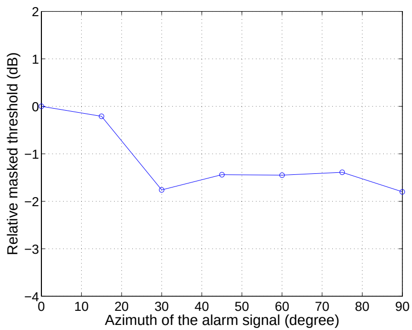
図 4.8: 成分周波数が 1.5 kHz の報知音の知覚特性: 被験者 G
