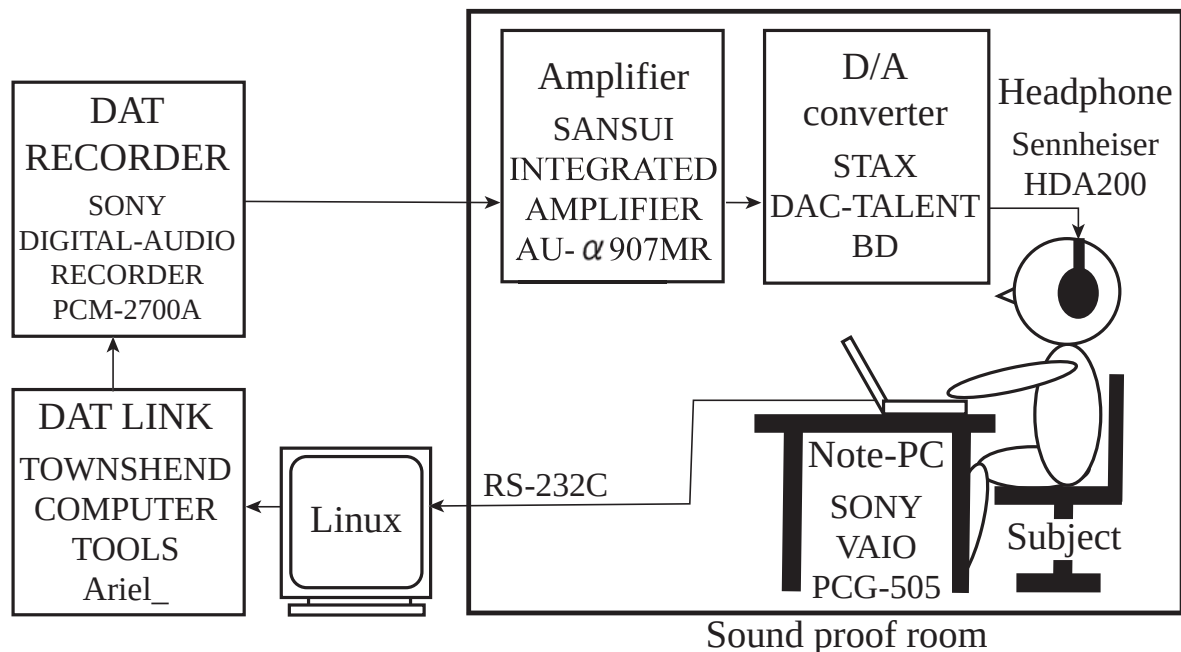
図 3.3: 実験システム
