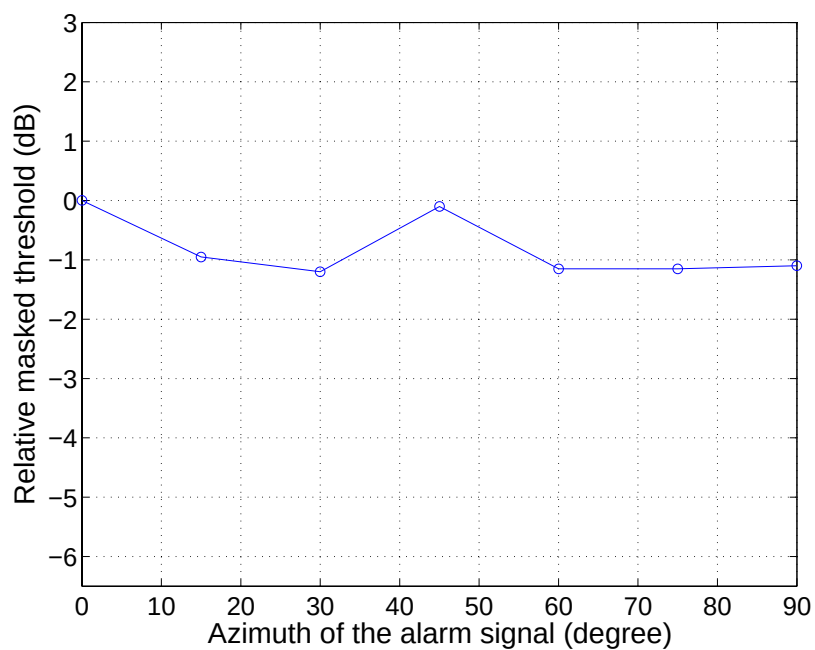
図 4.26: 成分周波数が 2.5 kHz の報知音の知覚特性: 被験者 G
