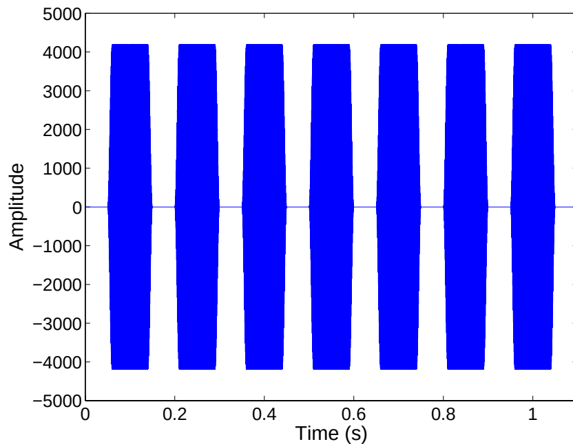
図 4.1: 実験に用いた報知音の例
