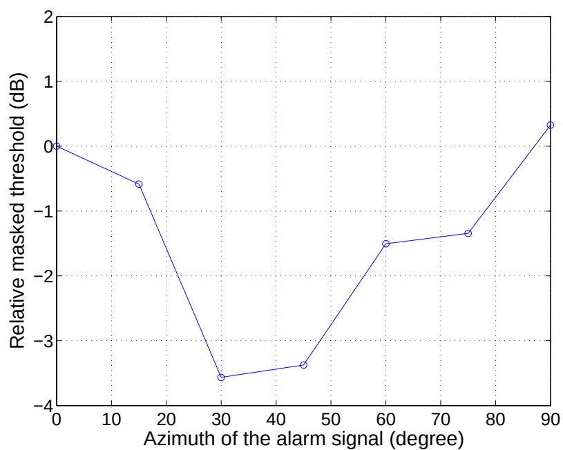
図 4.5: 成分周波数が 1.5 kHz の報知音の知覚特性: 被験者 D
