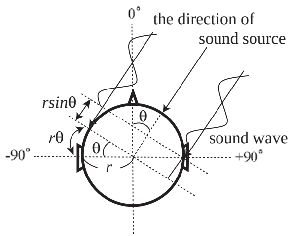
図 3.2: 角度 \theta (radian) から到来する音による ITD
