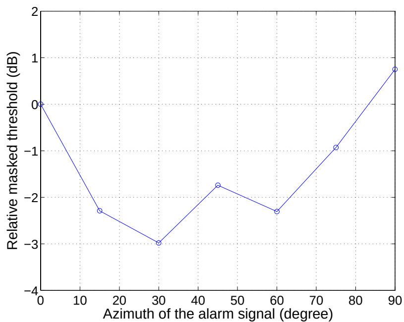
図 4.6: 成分周波数が 1.5 kHz の報知音の知覚特性: 被験者 E
