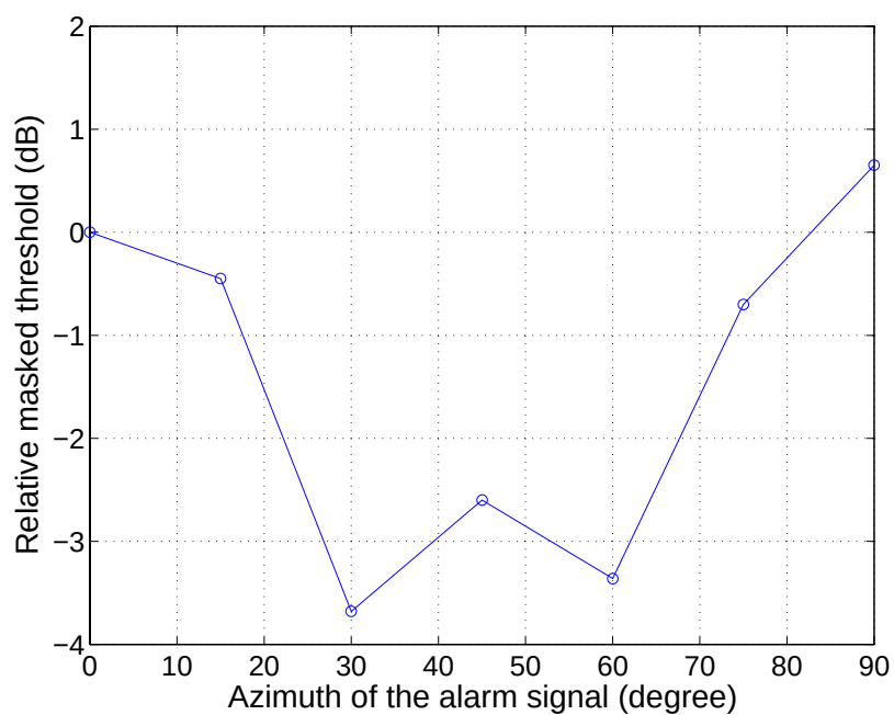
図 4.3: 成分周波数が 1.5 kHz の報知音の知覚特性: 被験者 B
