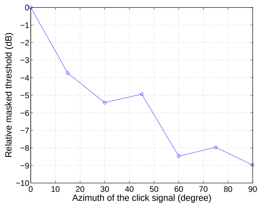
図 3.8: クリック音の知覚特性: 被験者 D
