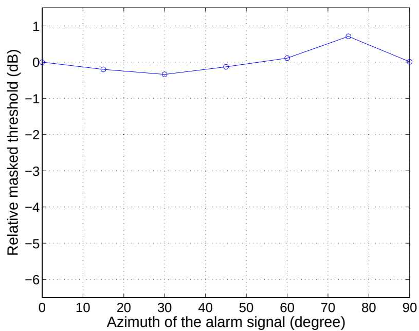
図 4.13: 成分周波数が 2.0 kHz の報知音の知覚特性: 被験者 C
