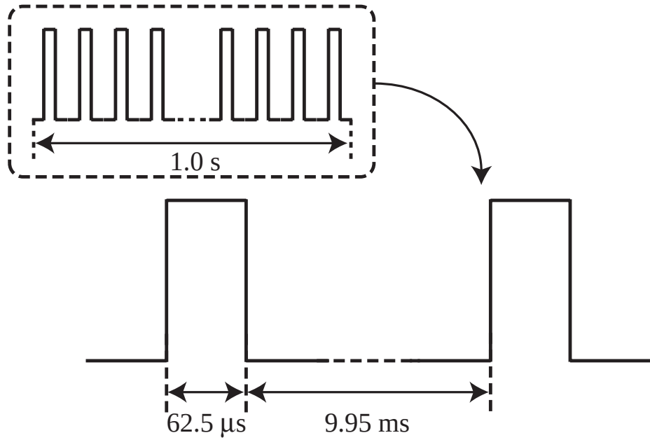
図 3.1: クリック音の概略図
