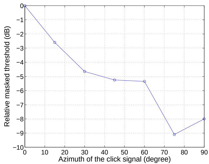
図 3.11: クリック音の知覚特性: 被験者 G
