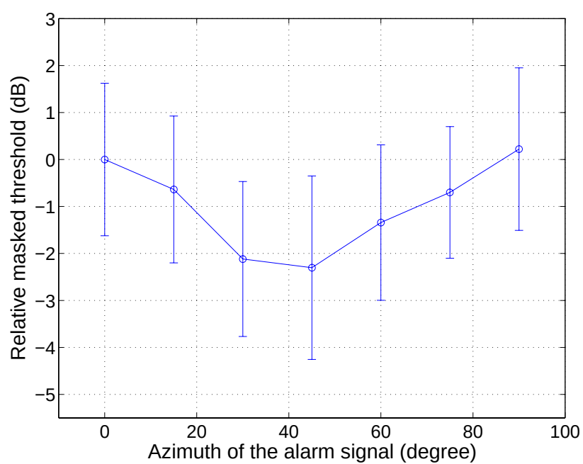
図 4.10: 成分周波数が 1.5 kHz の報知音の知覚特性: 全被験者の平均
