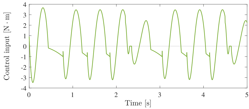
(e) 股関節の入力 u_3
