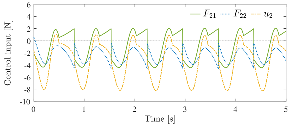
(d) 遊脚の入力 u_2 と遊脚の並進駆動力 F_{21} , F_{21}
