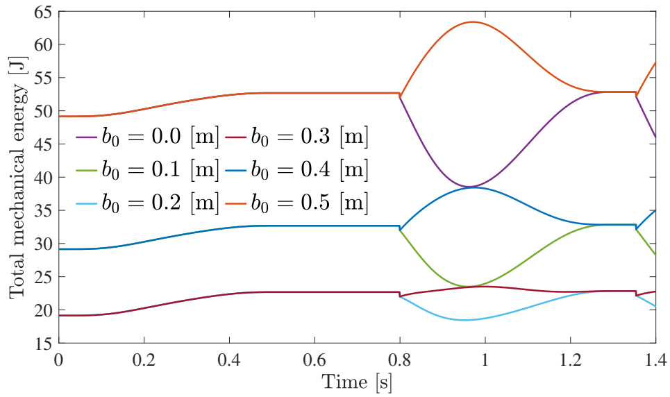
(b) k = 0.25 [N/m] における 6 つの自然長 b_0 の比較
