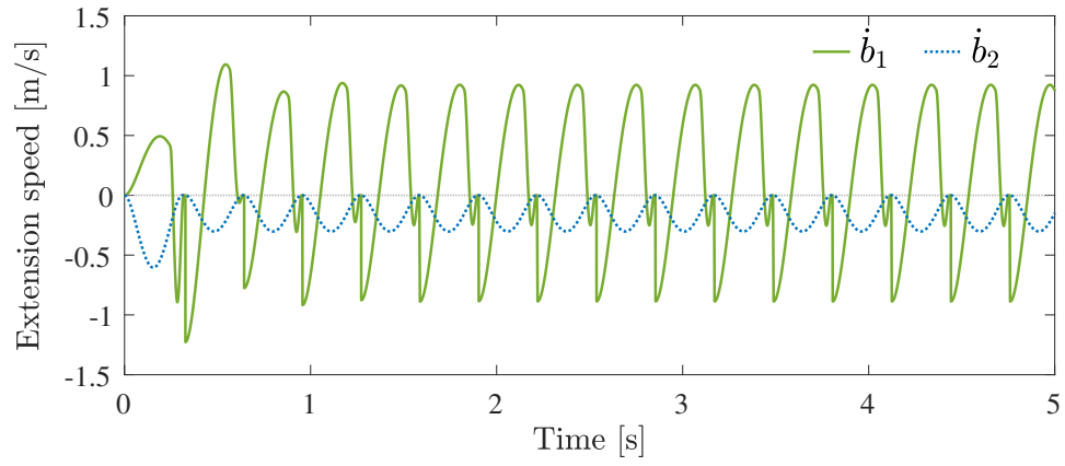
(g) 支持脚の伸縮速度 \dot{b}_1 と遊脚の伸縮速度 \dot{b}_2
