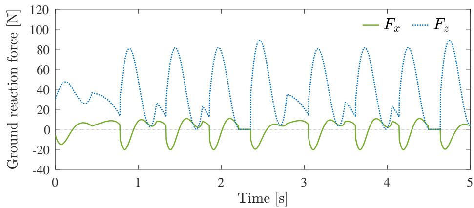
(f) 床反力 F_x と F_z
