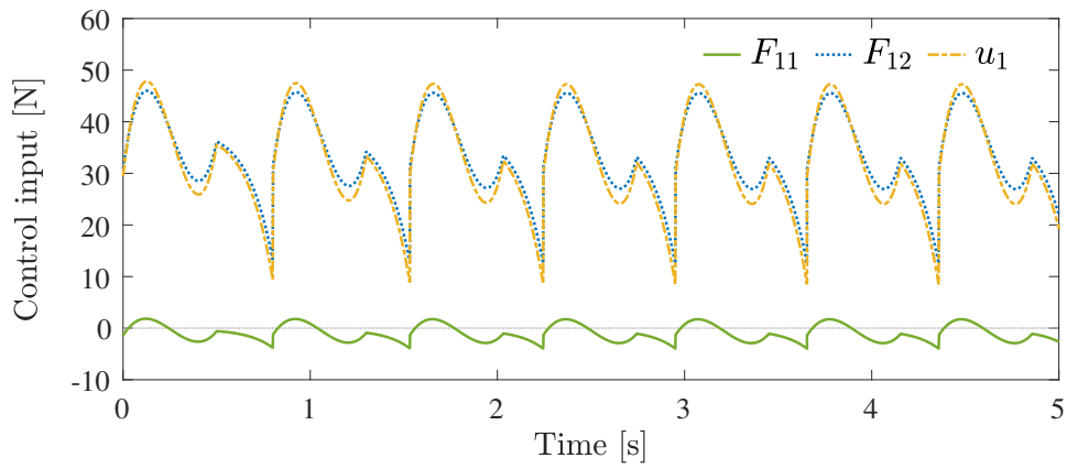
(c) 支持脚の入力 u_1 と支持脚の並進駆動力 F_{11} , F_{12}
