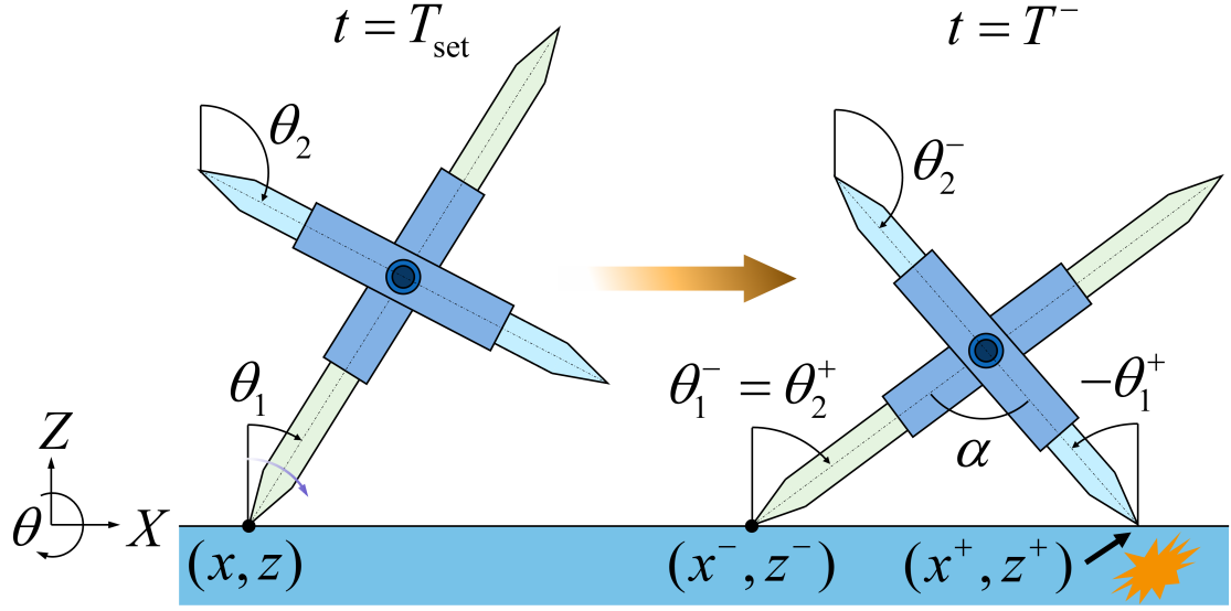
図 2.3: 脚交換の瞬間における座標系
