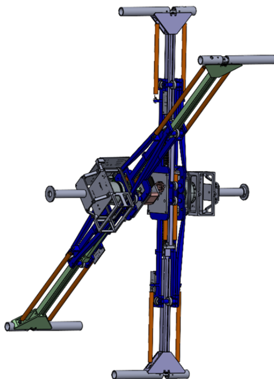
図 4.2: 弾性脚をもつ X 字型 2 脚ロボットの設計図
