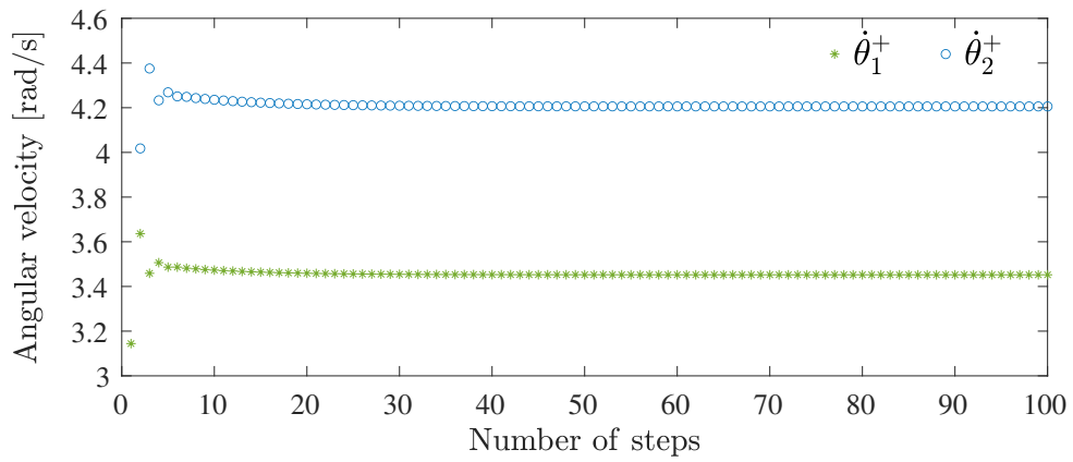
(c) 衝突直後の支持脚の角速度 \dot{\theta}_1^+ と遊脚の角速度 \dot{\theta}_2^+
