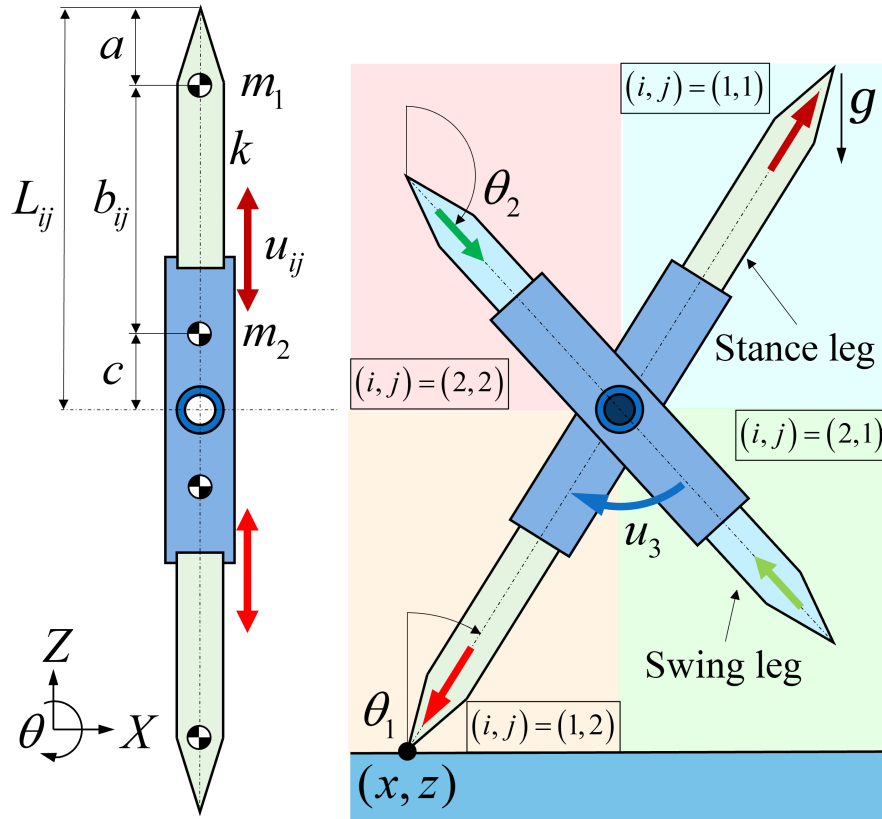
図 3.1: 伸縮脚をもつ X 字型 2 脚ロボットの冗長モデル
