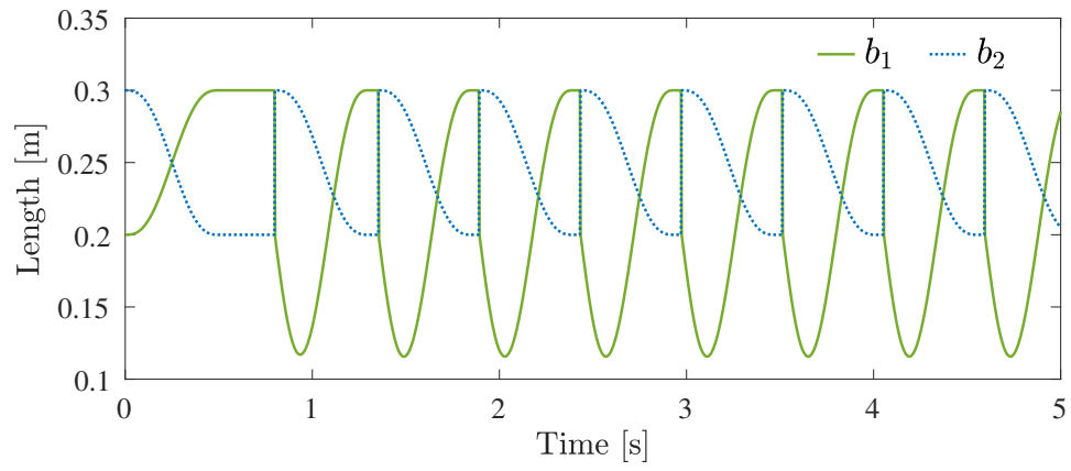
(b) 支持脚の長さ b_1 と遊脚の長さ b_2
