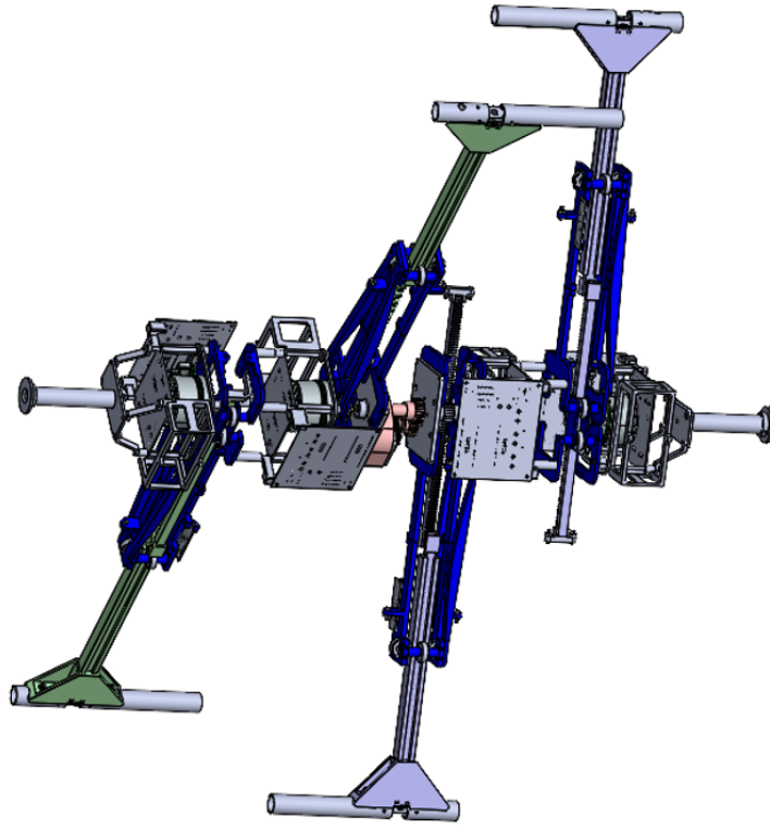
図 3.2: 5 入力モデルの設計図
