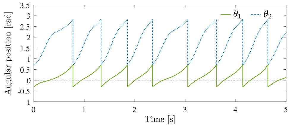
(b) 支持脚の角度 \theta_1 と遊脚の角度 \theta_2
