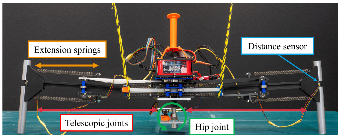
図 6.2: 股関節と伸縮脚の構造
