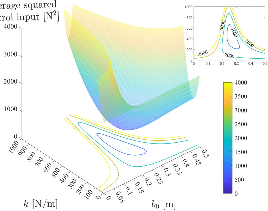
(b) 制御入力 2 の平均値
