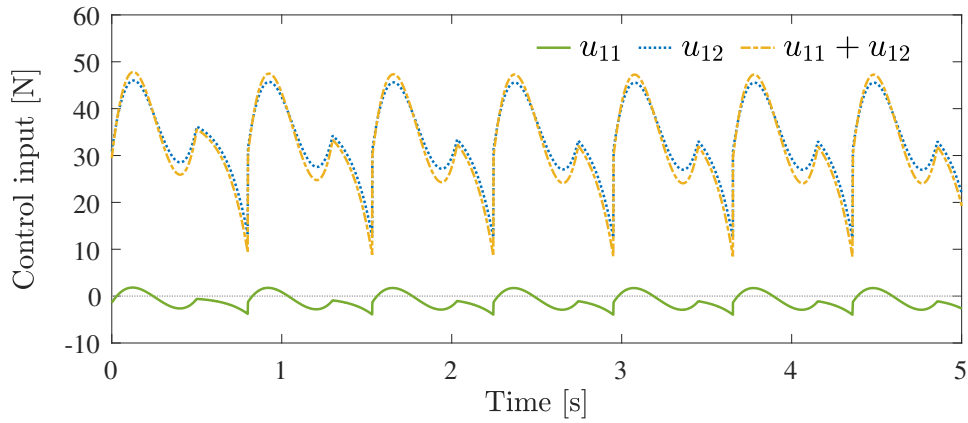
(a) 支持脚の入力 u_{11} と u_{12} およびそれらの合計値
