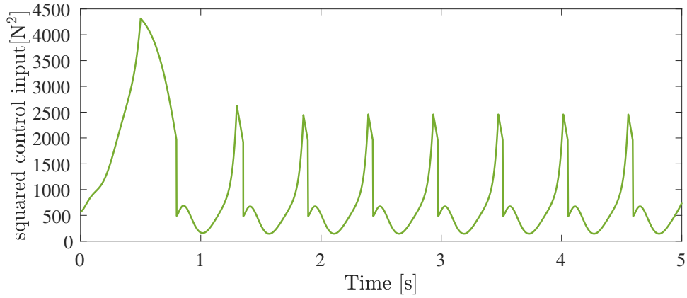
(d) 制御入力の2乗和 J
