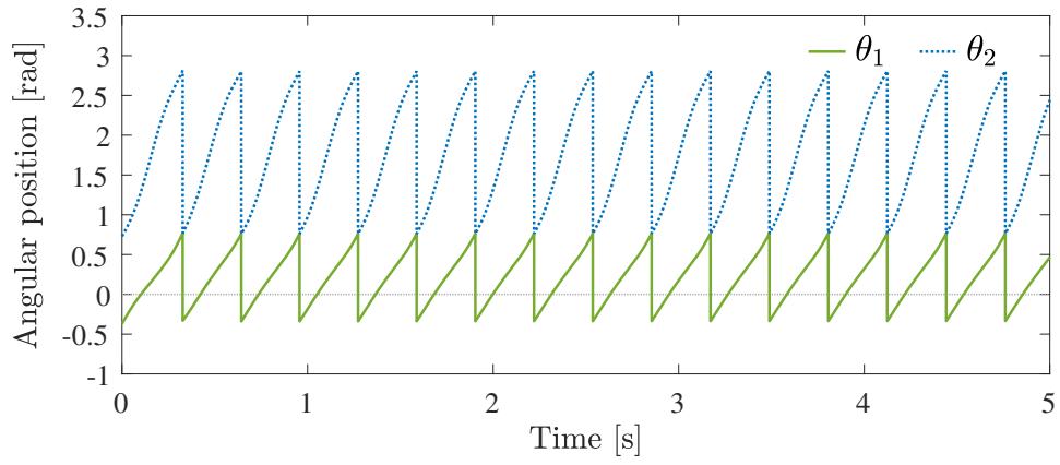
(d) 支持脚の角度 \theta_1 と遊脚の角度 \theta_2
