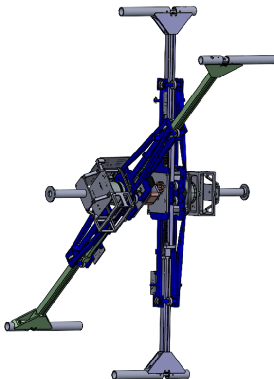
図 2.2: 伸縮脚をもつ X 字型 2 脚ロボットの設計図
