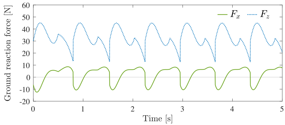
(e) 床反力 F_x と F_z
