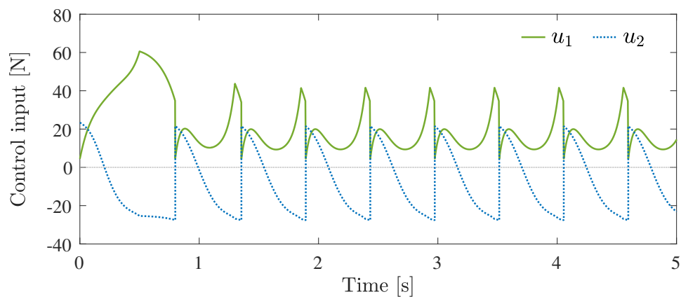
(a) 支持脚の入力 u_1 と遊脚の入力 u_2
