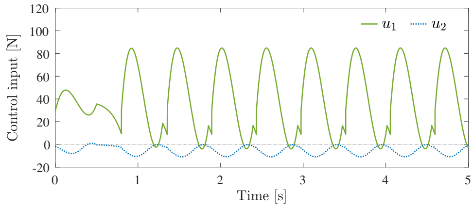
(c) 支持脚の入力 u_1 と遊脚の入力 u_2
