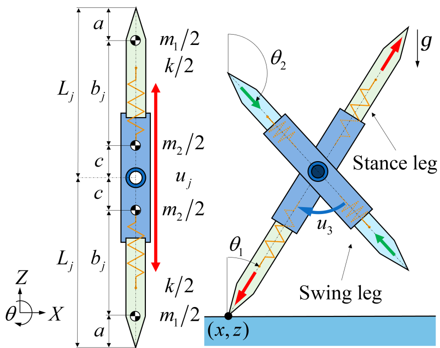
図 4.1: 弾性脚をもつ X 字型 2 脚ロボット
