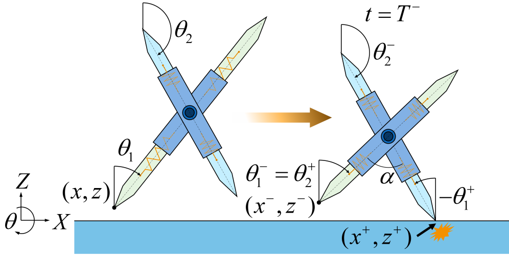
図 5.1: 脚交換の瞬間
