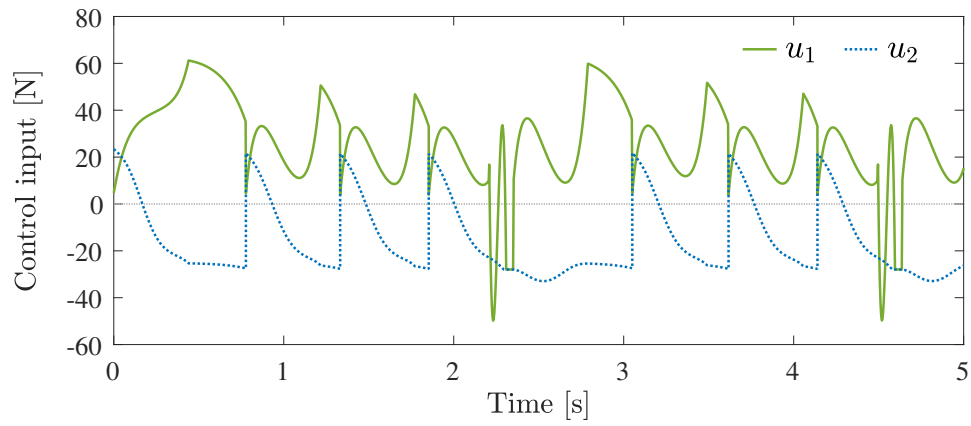
(d) 支持脚の入力 u_1 と遊脚の入力 u_2
