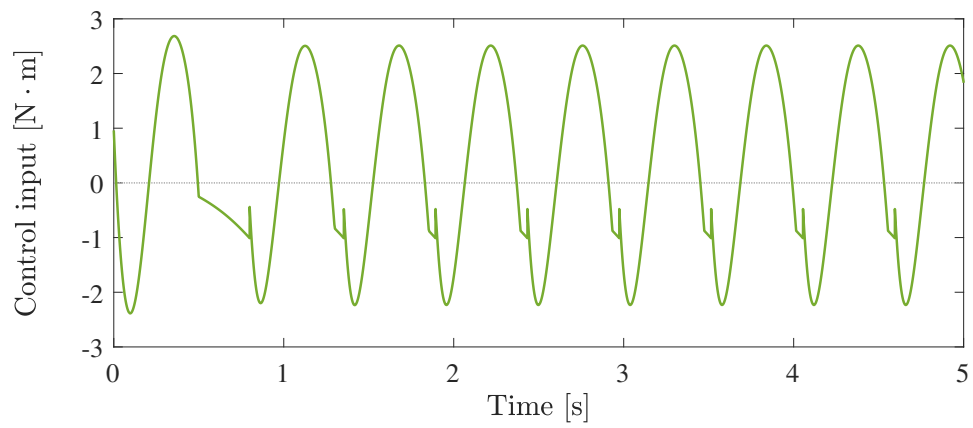
(d) 股関節の入力 u_3
