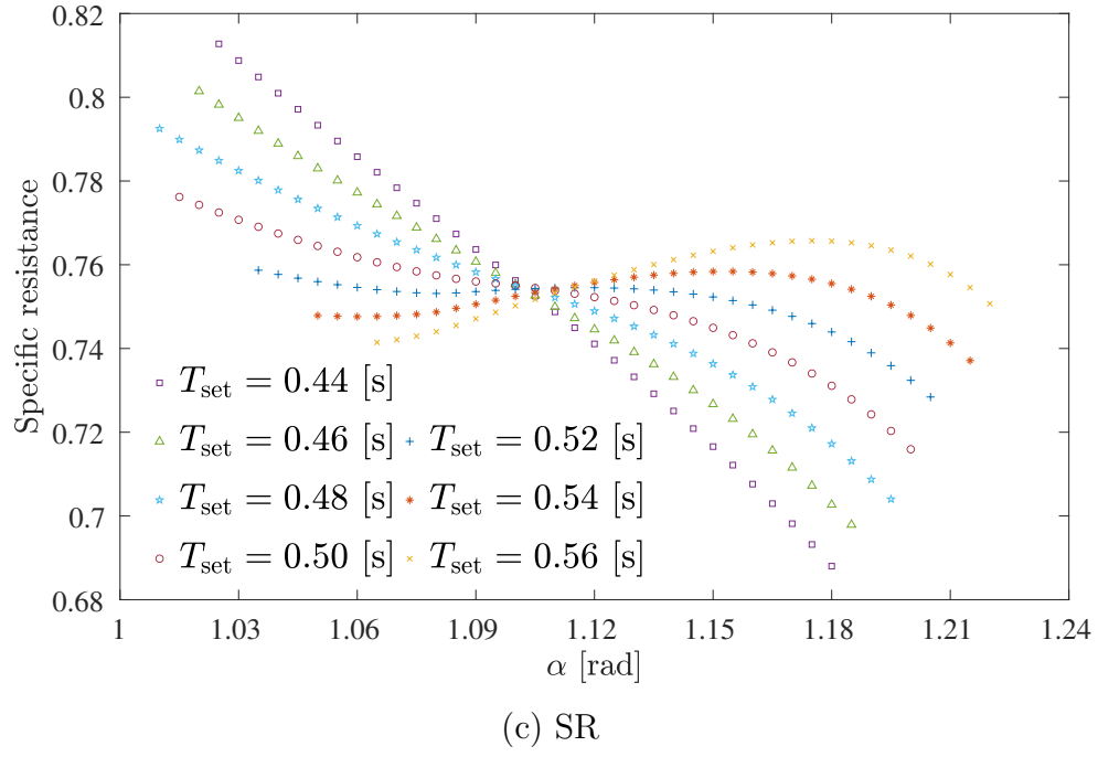
図 2.8: 衝突時に伸縮関節の機械的拘束を行わない車輪型歩容の歩行性能
