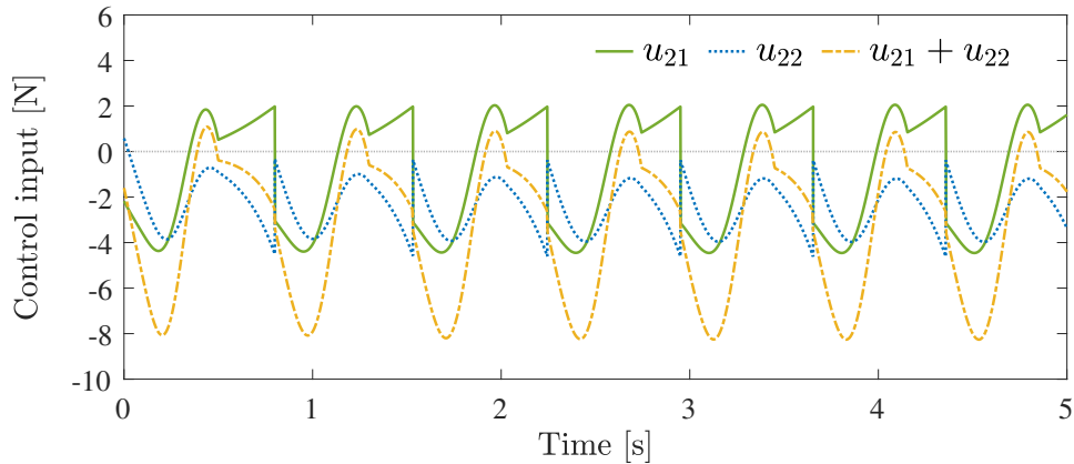
(b) 遊脚の入力 u_{11} と u_{12} およびそれらの合計値
