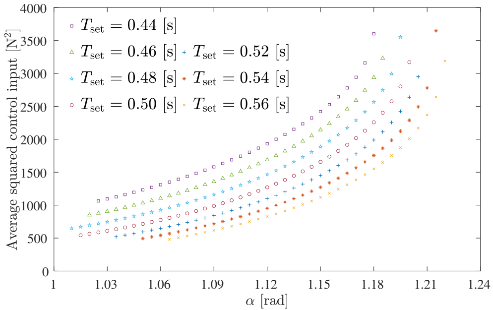
(b) 制御入力の2乗平均値
