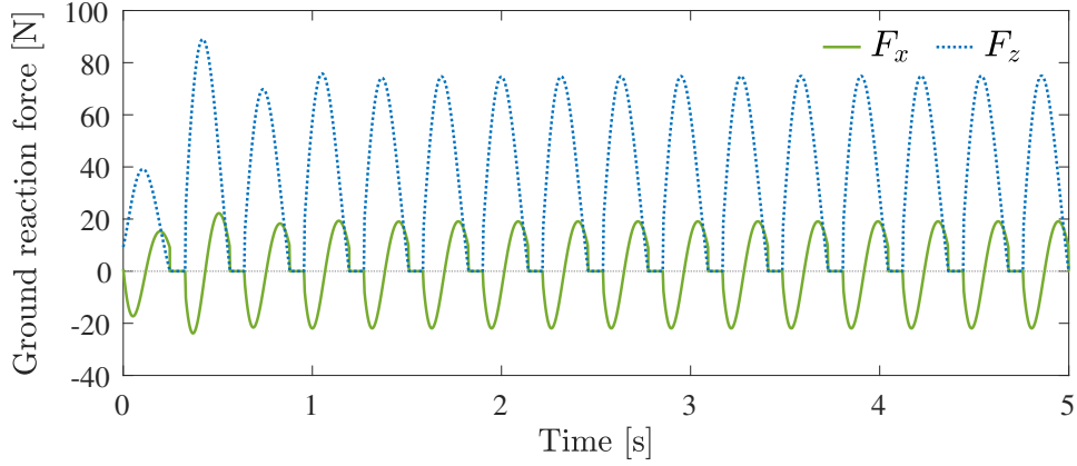
(j) 床反力 F_x と F_z
