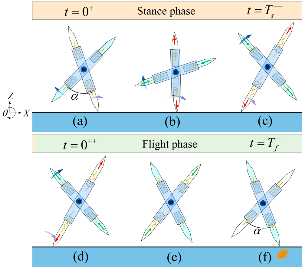
図 5.2: 車輪型走行歩容のシーケンス図
