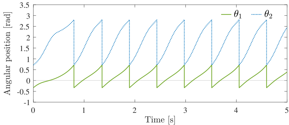
(a) 支持脚の角度 \theta_1 と遊脚の角度 \theta_2
