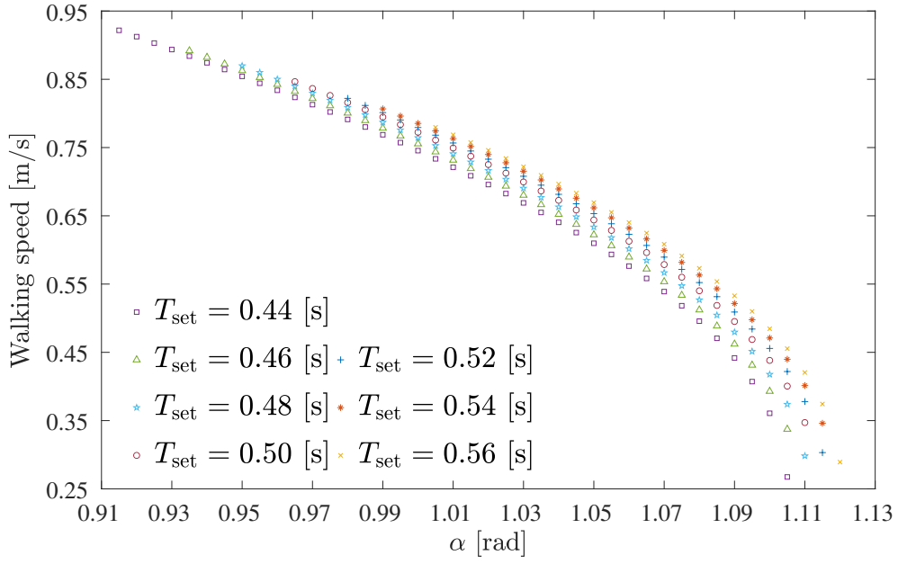
(b) 歩行速度
