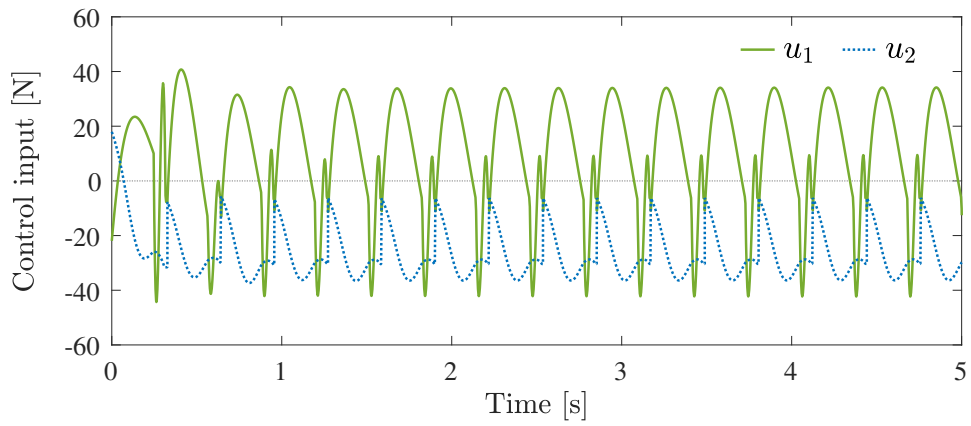
(f) 支持脚の入力 u_1 と遊脚の入力 u_2
