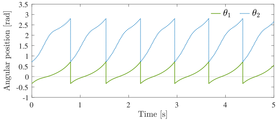
(a) 支持脚の角度 \theta_1 と遊脚の角度 \theta_2
