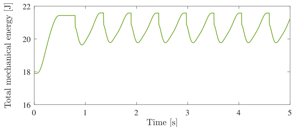
(b) 全力的エネルギー E
