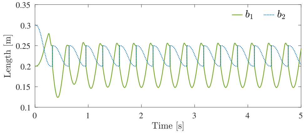
(e) 支持脚の長さ b_1 と遊脚の長さ b_2
