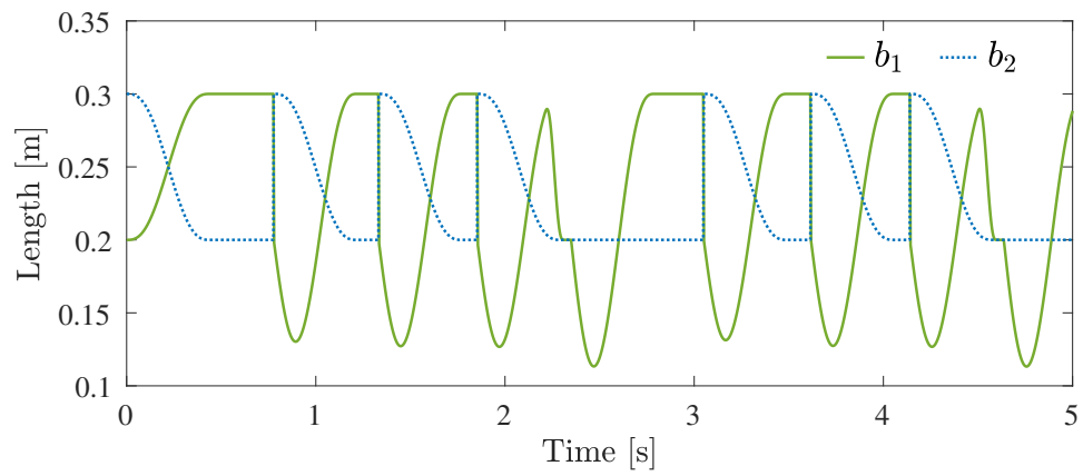
(c) 支持脚の長さ b_1 と遊脚の長さ b_2
