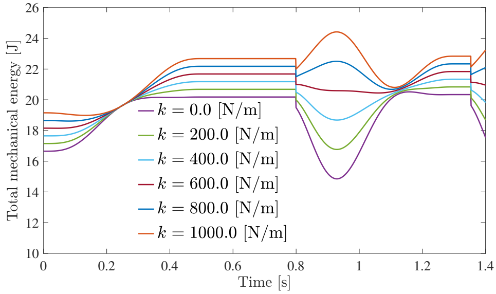
(a) b_0 = 0.25 [m] における 6 つの弾性係数 k の比較
