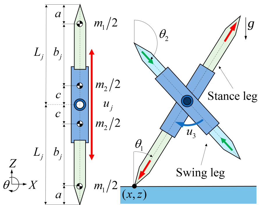
図 2.1: 伸縮脚をもつ X 字型 2 脚ロボット
