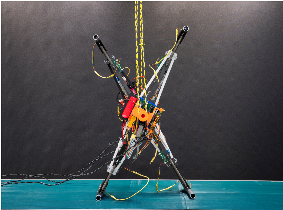
図 6.1: 弾性脚をもつ X 字型 2 脚ロボットの実験機
