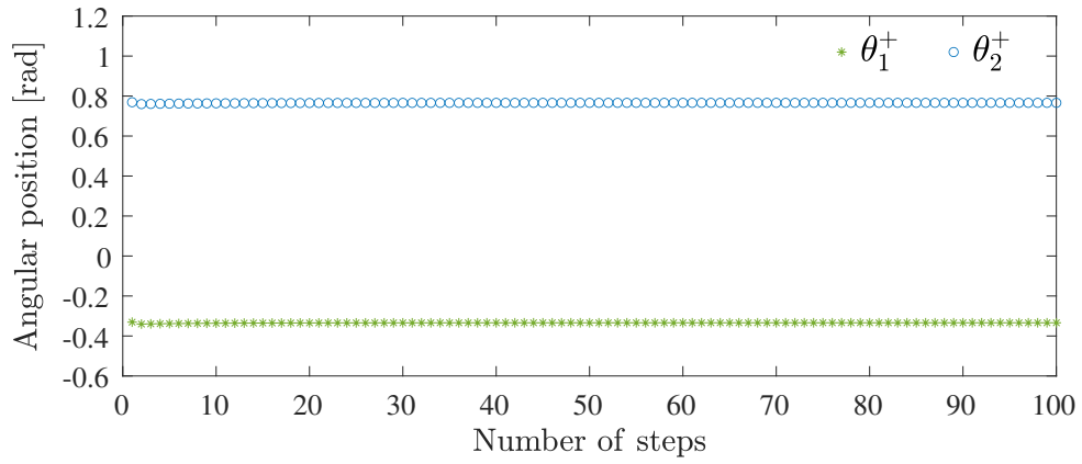
(b) 衝突直後の支持脚の角度 \theta_1^+ と遊脚の角度 \theta_2^+
