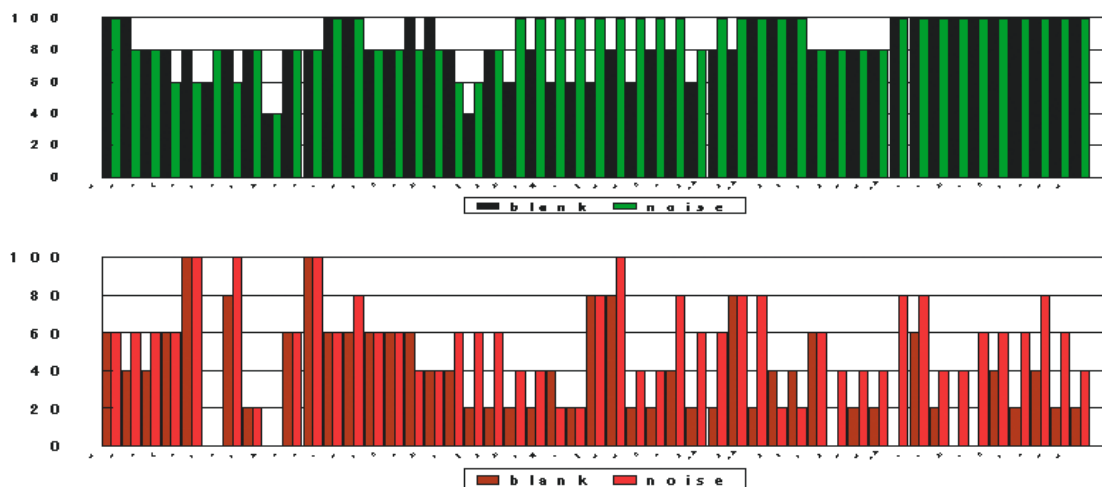
図 3.3: 文章 1 の各音素の正解率
